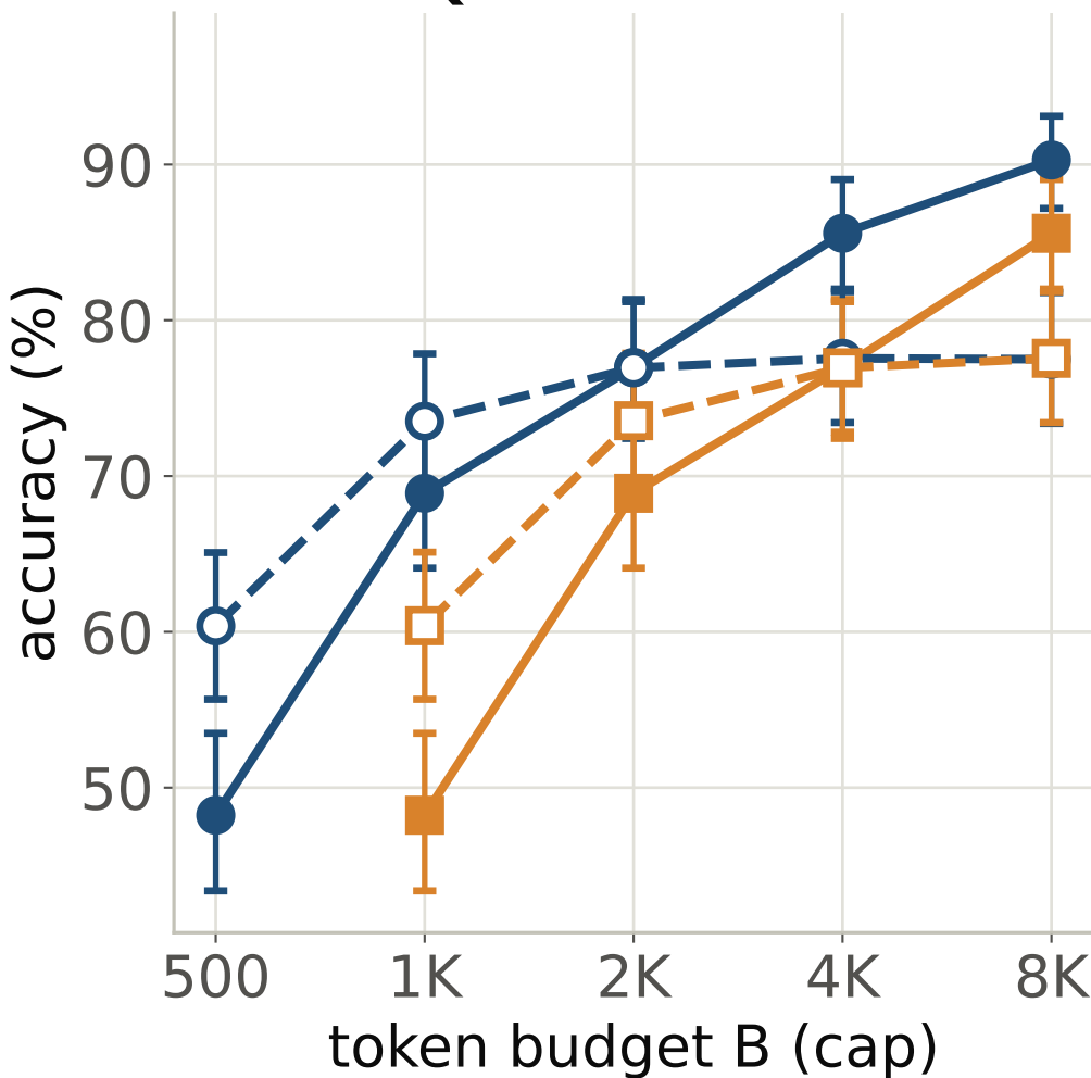
Qwen3-1.7B
