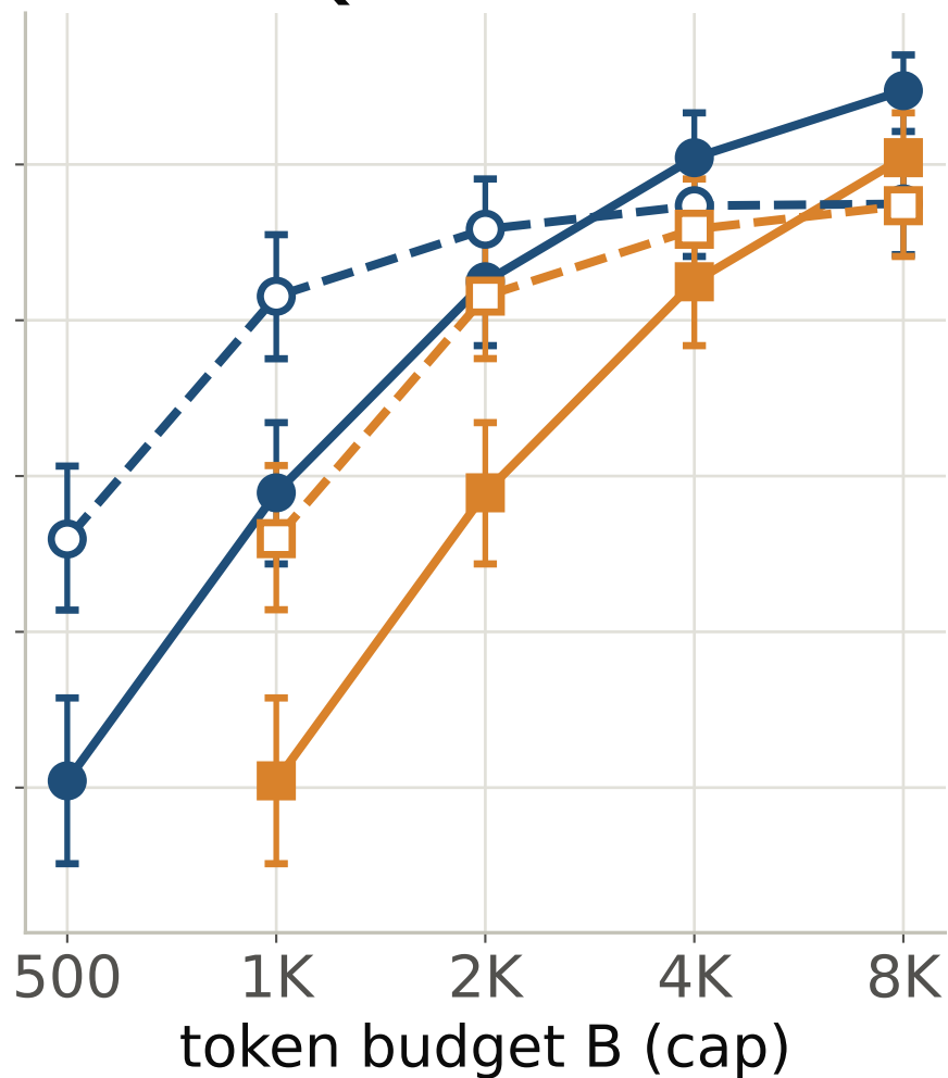
Qwen3-4B
