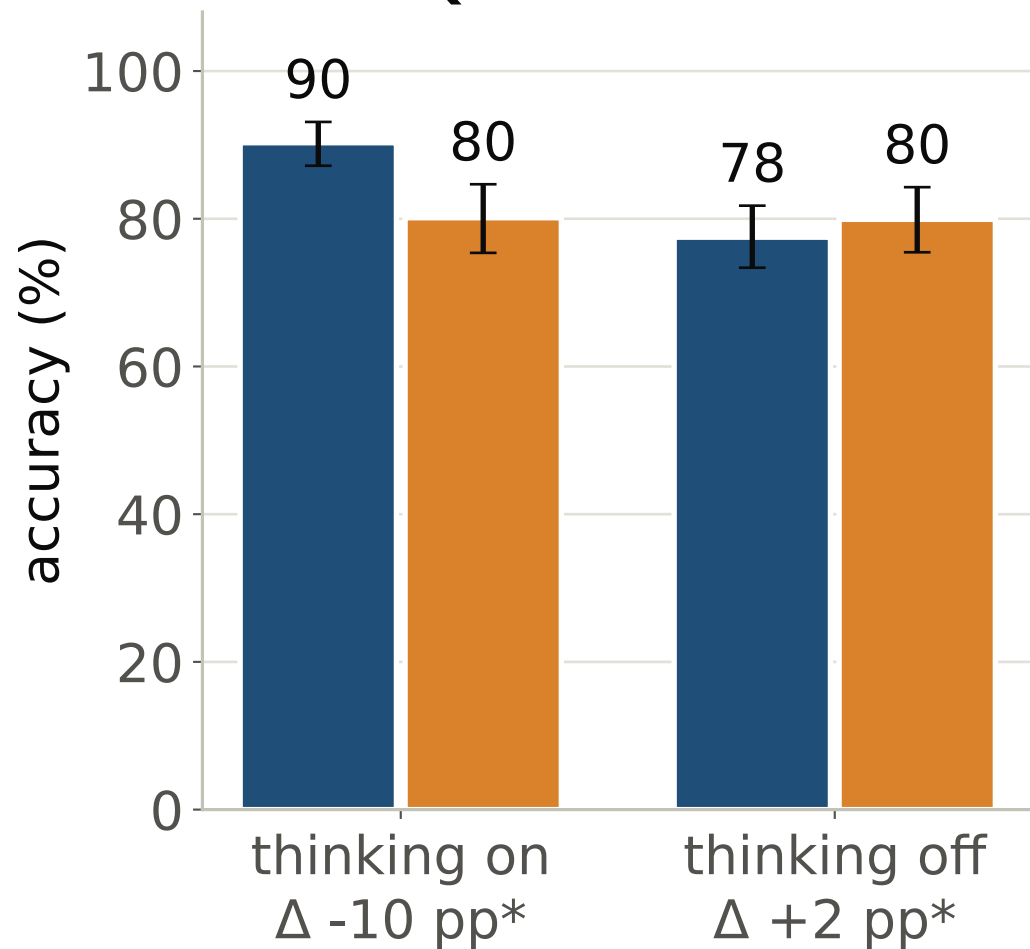
Qwen3-1.7B
