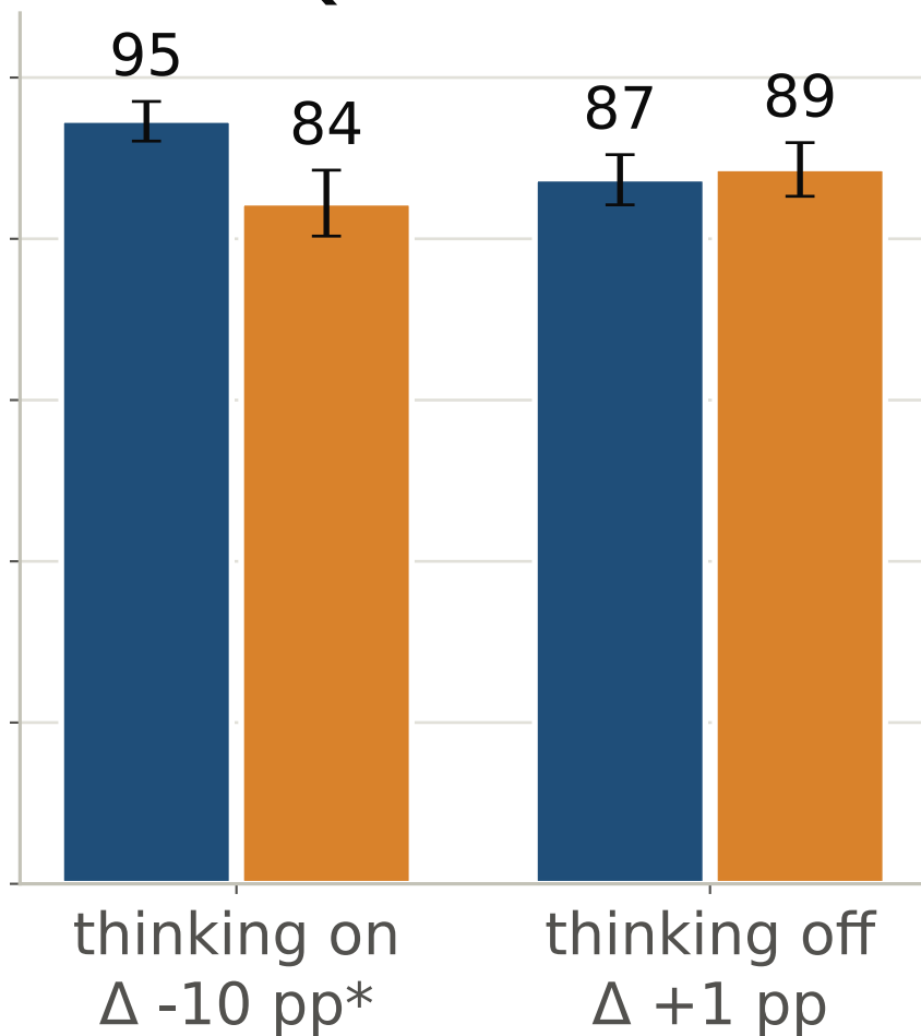
Qwen3-4B
