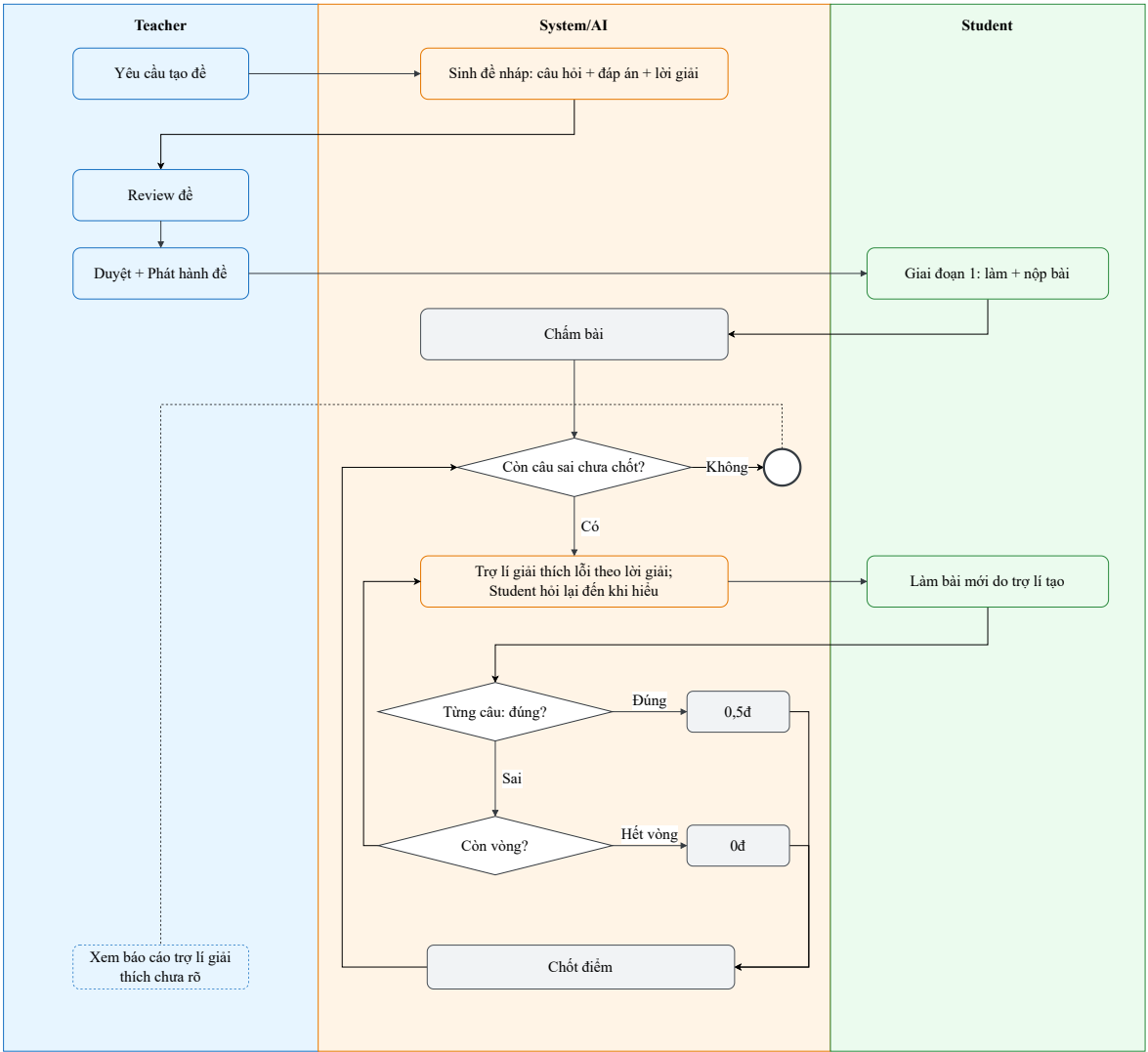
Hình 4.2: Business Workflows
