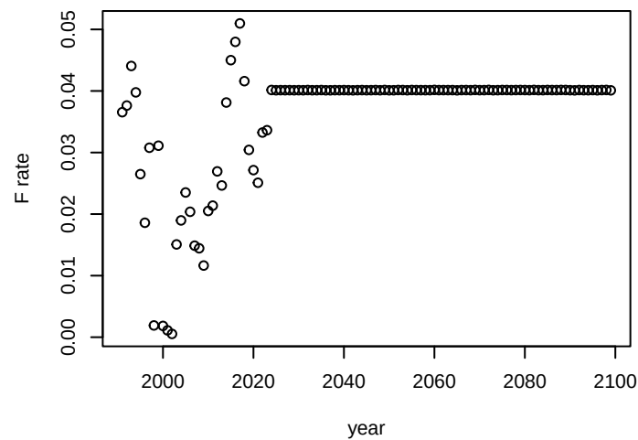
pacific_cod_adult gfdl_245
