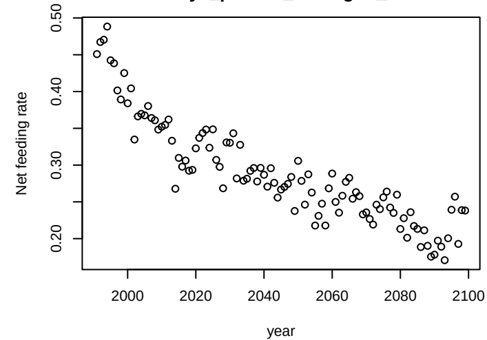
pacific_cod_adult gfdl_245
