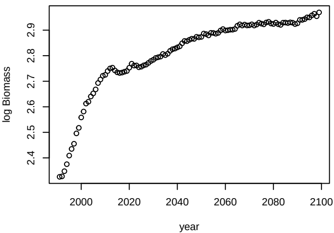
pacific_cod_adult gfdl_245
