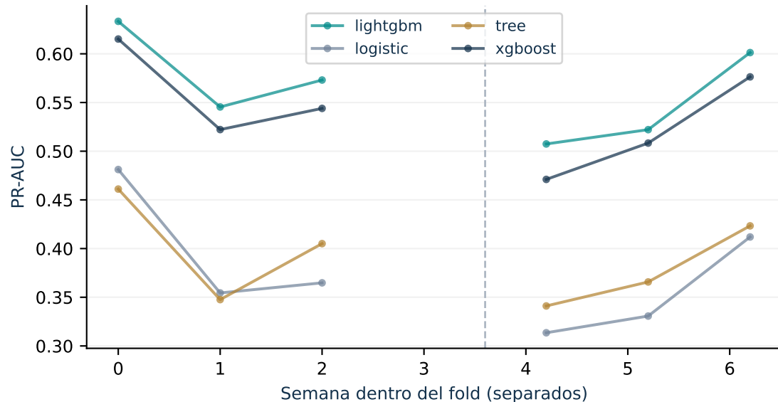
PR-AUC semanal en dos folds históricos
