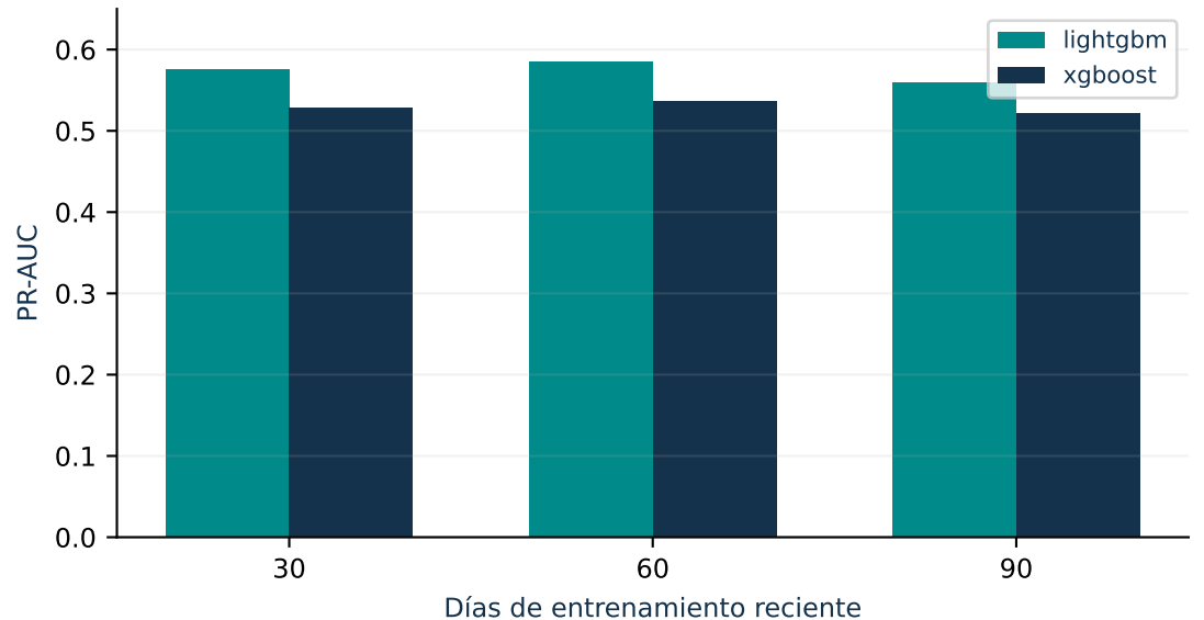
PR-AUC en validación por ventana
