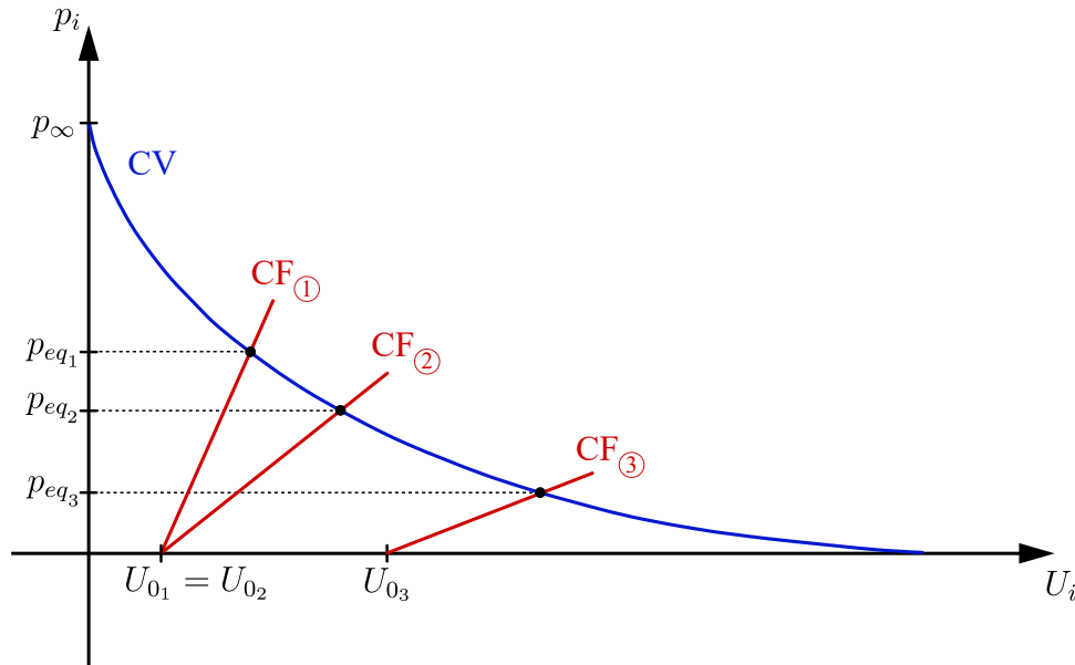
Figura 2.20 – Curvas características do maciço (CV) e do revestimento (CF)
