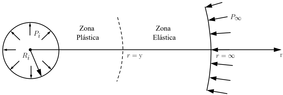
Figura 2.17 – Delimitação das regiões plástica e elástica (adaptado de Bernaud (1991))
