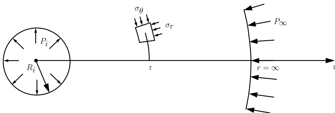
Figura 2.16 – Geometria e carregamento do túnel (adaptado de Bernaud (1991))
