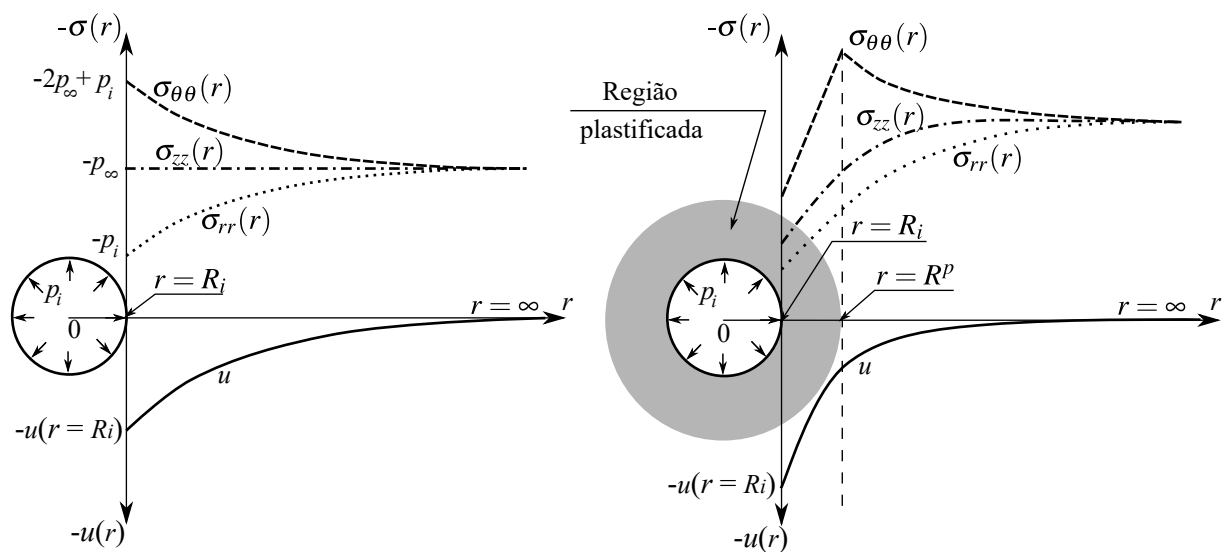
Figura 2.18 – Deslocamentos e tensões no entorno de um maciço submetido à pressão geostática-hidrostatica p_\infty e pressão interna p_i no interior da seção do túnel. Esquerda: elasticidade. Direita: elastoplasticidade. (QUEVEDO, 2021)
