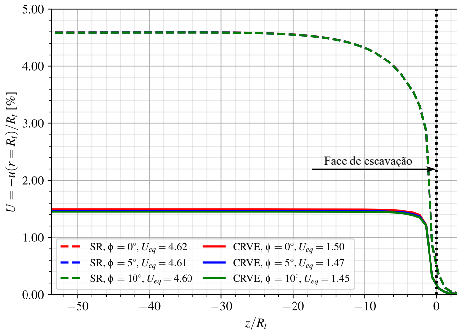
Figura 6.4 – Perfis de convergência no longo prazo - túnel isolado sem revestimento (SR) e com revestimento viscoelástico (CRVE)
