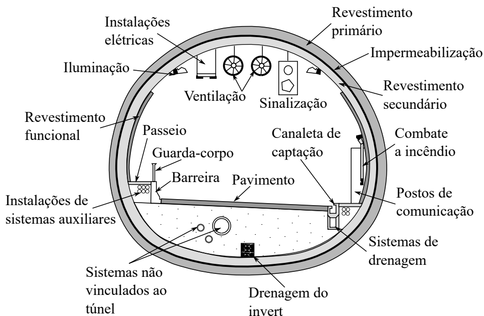
Figura 2.8 – Elementos de revestimento de túnel rodoviário (adaptado de DEPARTAMENTO DE ESTRADAS E RODAGEM (SÃO PAULO) (2005))
