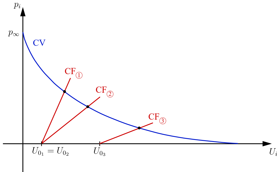
Figura 2.13 – Curvas características do maciço e do revestimento
