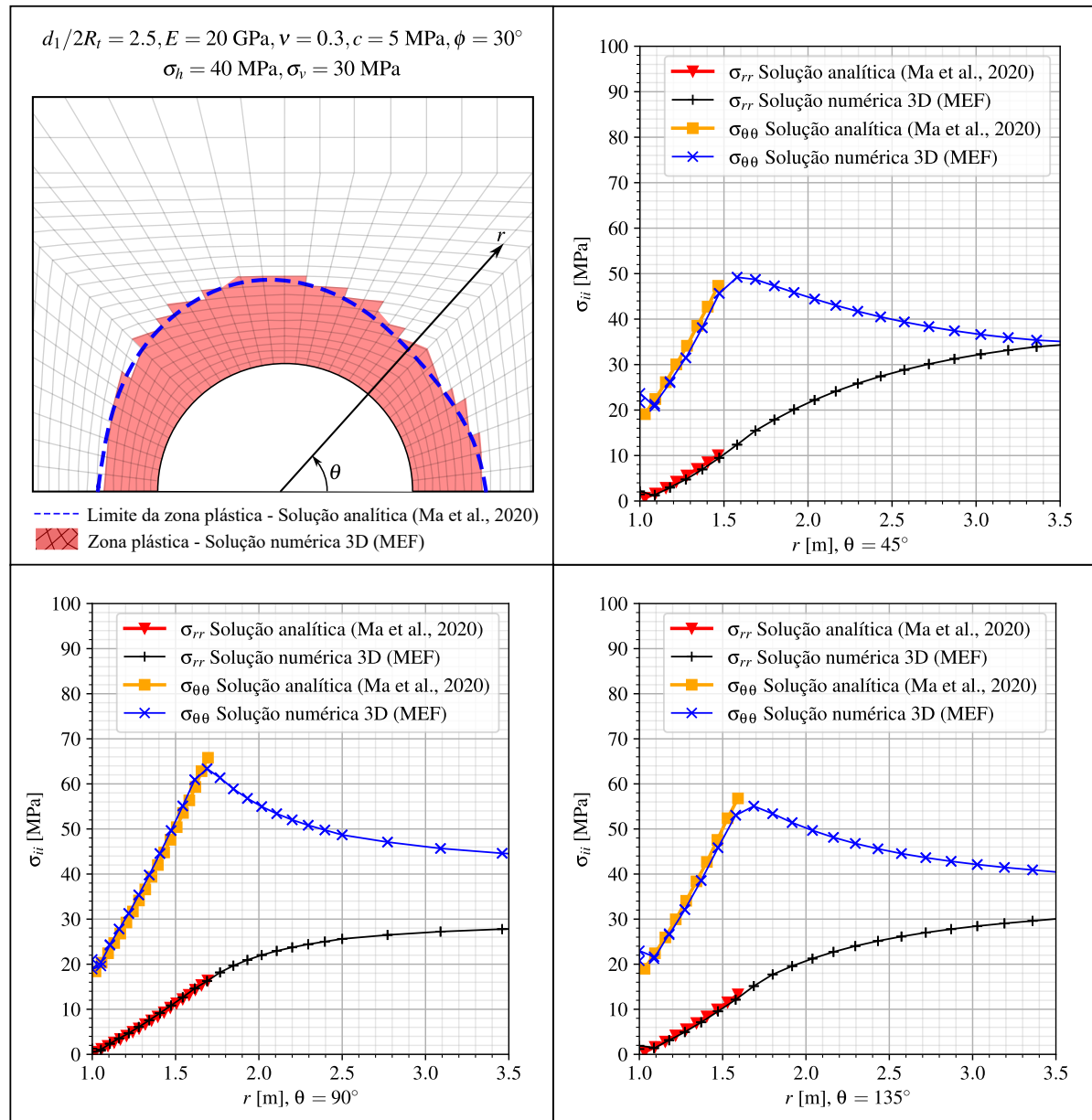
Figura 4.15 – Distribuição dos componentes de tensão radial e ortoradial ao longo de diferentes direções radiais: comparação entre simulações numérica e analítica - critério Mohr-Coulomb
