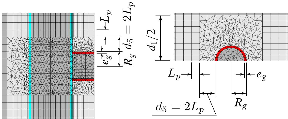
Figura 4.6 – Detalhamento da galeria transversal. Esquerda: vista da região de encontro entre o túnel longitudinal e a galeria no plano de simetria y = 0 ; Direita: detalhe da malha de elementos finitos na seção transversal da galeria (adaptado de Colombo (2023))
