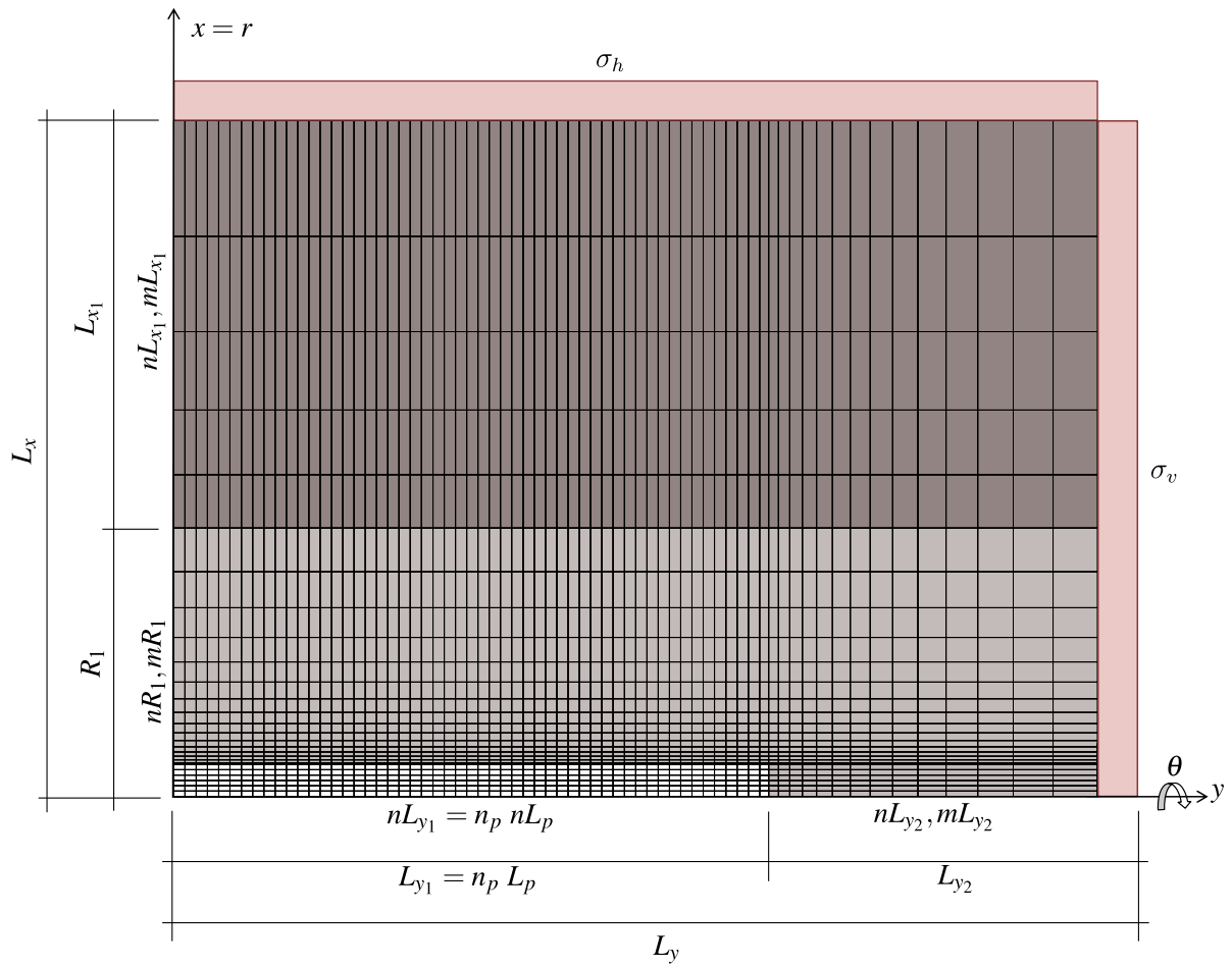
Figura 4.2 – a) Domínio, condições de contorno e parâmetros geométricos do modelo axissimétrico (b) Detalhe dos parâmetros que envolvem a escavação (adaptado de Quevedo (2021))
