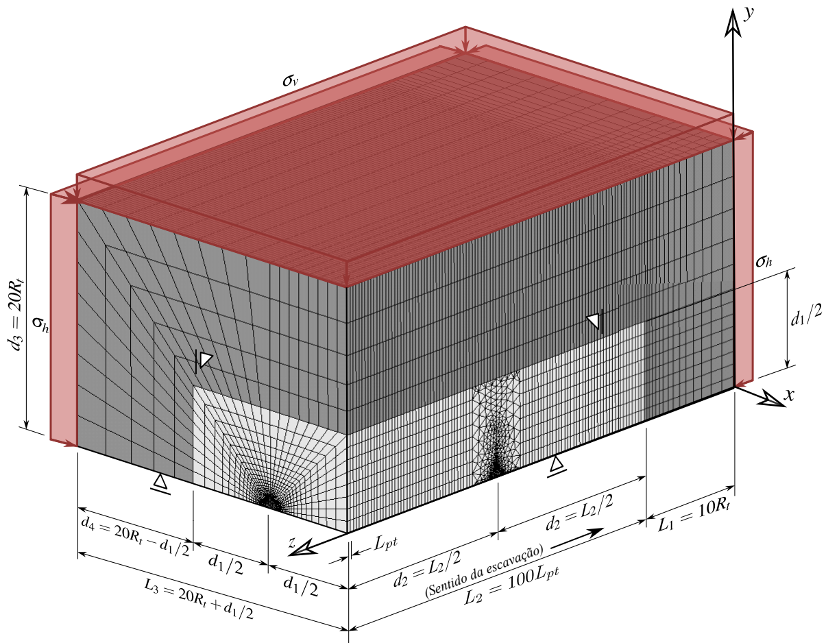
Figura 4.4 – Malha, dimensões e condições de contorno do domínio dos túneis gêmeos tridimensionais (adaptado de Colombo (2023))
