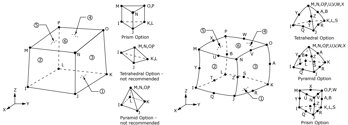
Figura 4.3 – Elementos SOLID185 e SOLID186 (ANSYS Inc, 2024)
