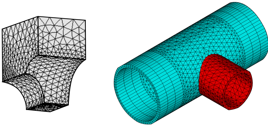
Figura 4.7 – Esquerda: vista isométrica da zona de transição no maciço; Direita: vista isométrica da zona de intersecção do revestimento túnel/galeria (adaptado de Colombo (2023))
