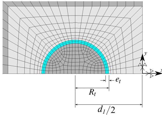
Figura 4.5 – Detalhe da malha de elementos finitos na seção transversal do túnel longitudinal (adaptado de Colombo (2023))
