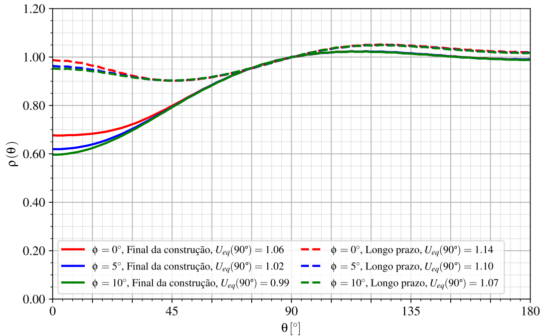
Figura 7.13 – Anisotropia das deformações - túneis gêmeos sem galeria com revestimento elástico (CRE)
