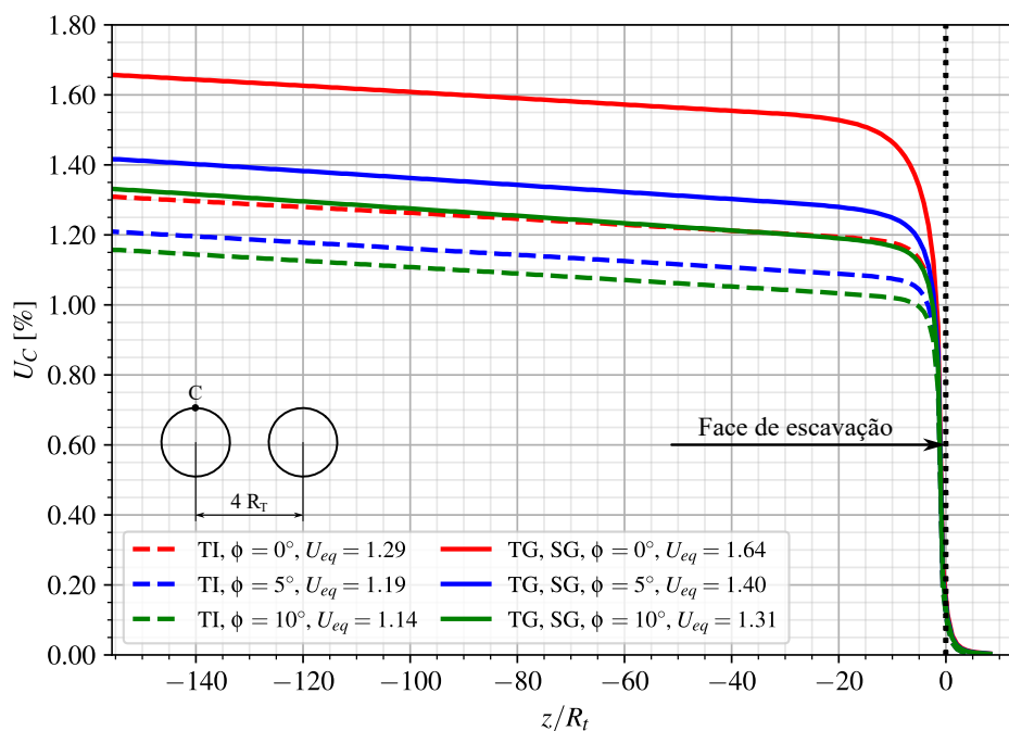
Figura 7.2 – Perfis de convergência - túnel isolado (TI) e túneis gêmeos (TG) sem galeria (SG) e sem revestimento (SR) no final da construção
