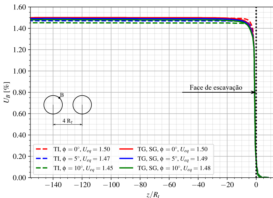
Figura A.12 – Perfis de convergência - Ponto B - túnel isolado (TI) e túneis gêmeos (TG) com revestimento viscoelástico (CRVE) no longo prazo
