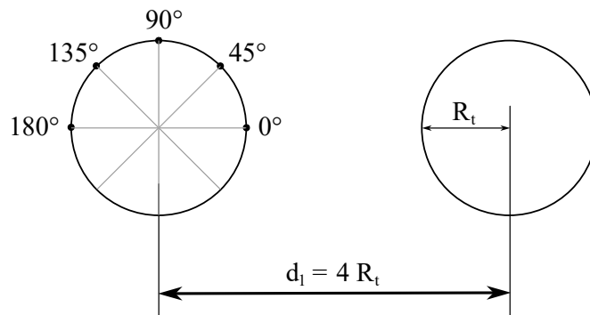
Figura 7.12 – Posições dos ângulos \theta no contorno da seção transversal do túnel
