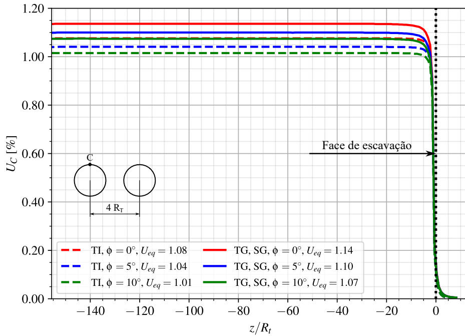
Figura 7.5 – Perfis de convergência - túnel isolado (TI) e túneis gêmeos (TG) sem galeria (SG), com revestimento elástico (CRE) no longo prazo
