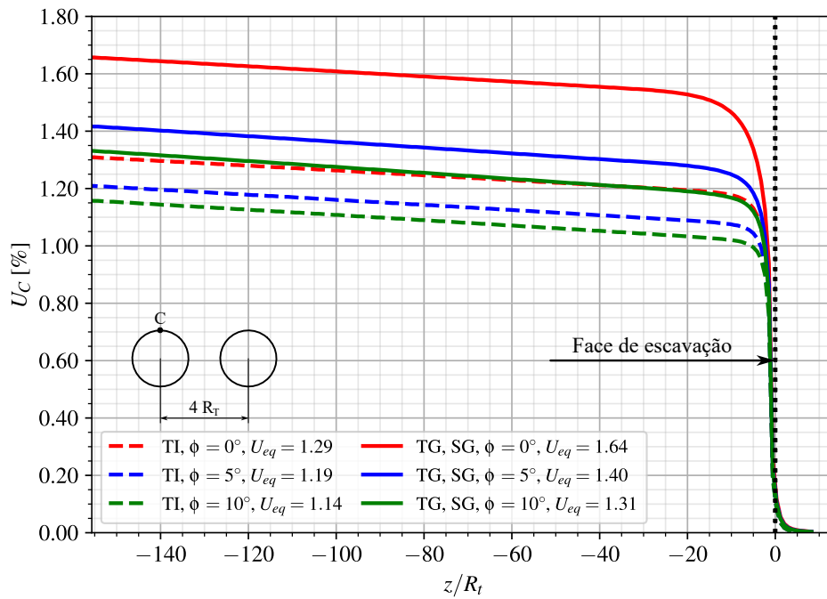
Figura 7.2 – Perfis de convergência - túnel isolado (TI) e túneis gêmeos (TG) sem galeria (SG), sem revestimento (SR) no final da construção
