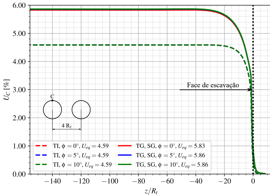
Figura 7.3 – Perfis de convergência - túnel isolado (TI) e túneis gêmeos (TG) sem galeria (SG), sem revestimento (SR) no longo prazo
