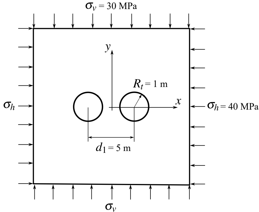
Figura 4.8 – Geometria e carregamento dos túneis gêmeos estudados por Ma et al. (2020))
