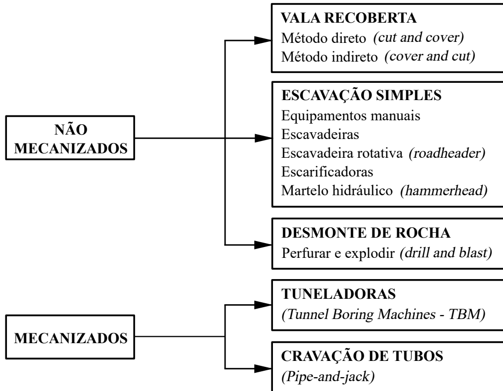
Figura 2.3 – Métodos de escavação de túneis (adaptado de ??)
