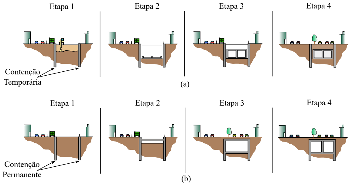
Figura 2.4 – Método de escavação vala recoberta. a) cut and cover e b) cover and cut (adaptado de ??)
