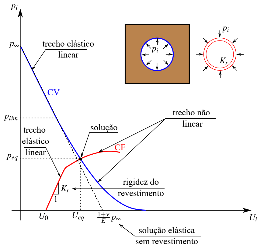
Figura 2.22 – Método convergência-confinamento (??)
