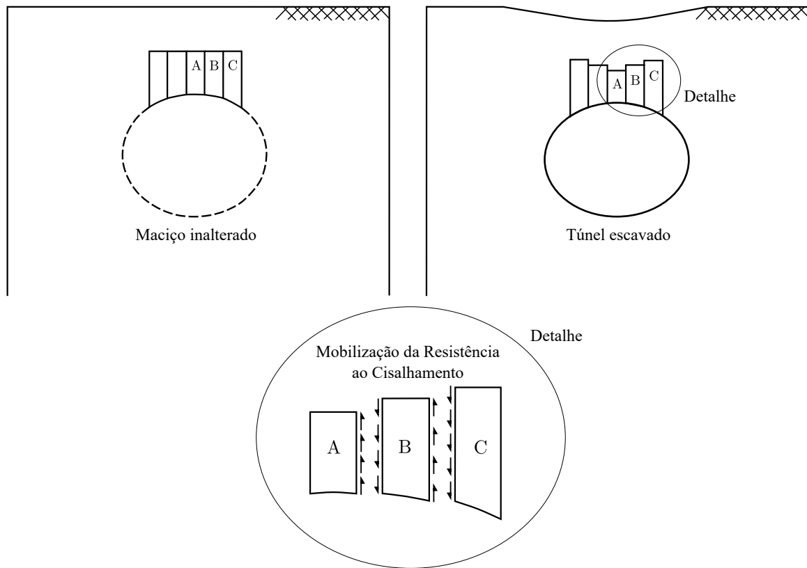
Figura 2.11 – Efeito arco: mobilização da resistência ao cisalhamento do maciço nos arredores da escavação (adaptado de ??)
