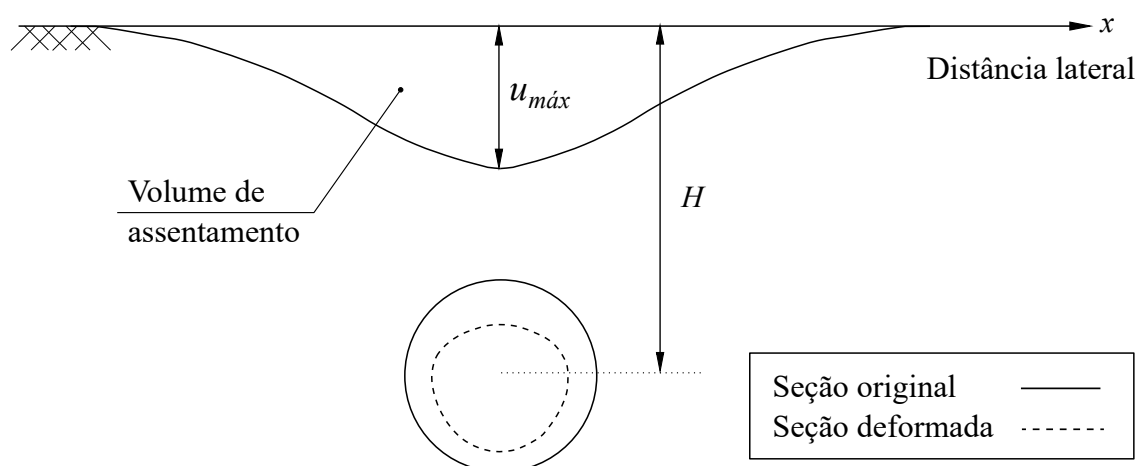
Figura 2.18 – Forma do assentamento superficial (adaptado de ??)
