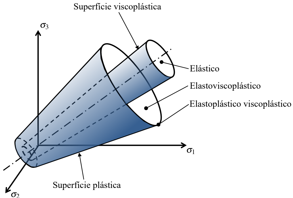
Figura 3.4 – Domínios e superfícies do modelo elastoplástico viscoplástico (adaptado de ??)
