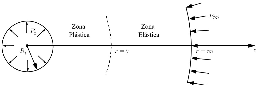
Figura 2.20 – Delimitação das regiões plástica e elástica (adaptado de ??)
