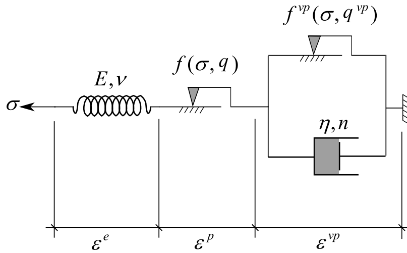
Figura 3.2 – Representação reológica do modelo elastoplástico viscoplástico (adaptado de ??)
