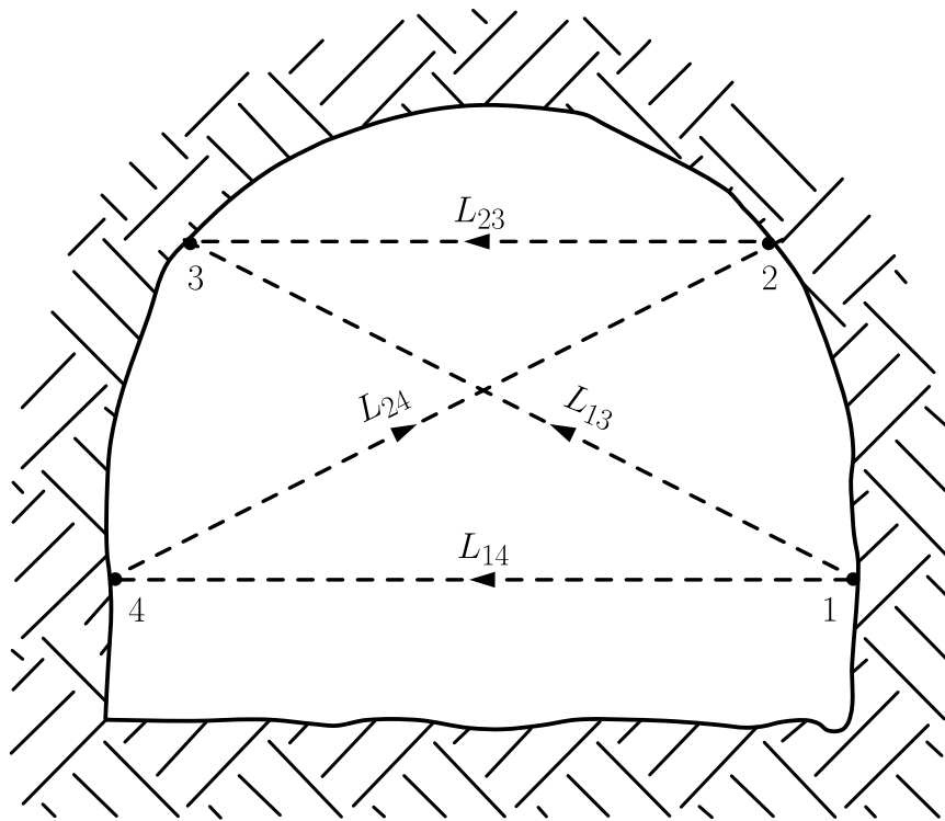
Figura 2.15 – Seção de medição de convergência em quatro direções (adaptado de ??)
