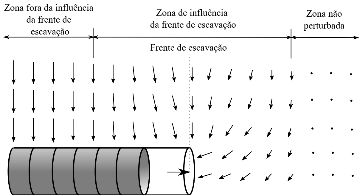
Figura 2.14 – Campo vetorial de deslocamentos no maciço durante a escavação de um túnel (adaptado de ??)
