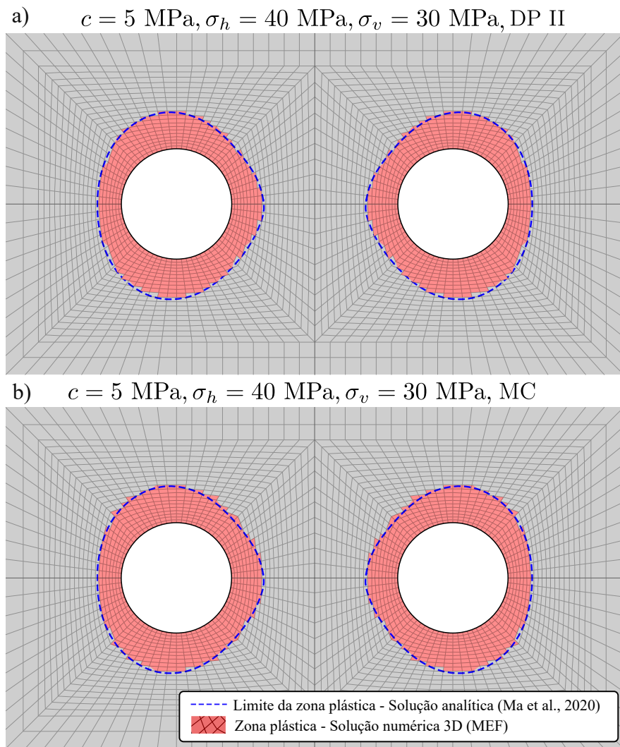
Figura 4.13 – Extensão da zona plástica obtida com as simulações numéricas do presente estudo e solução de tensão fornecida por ??). a) Drucker-Prager; b) Mohr-Coulomb
