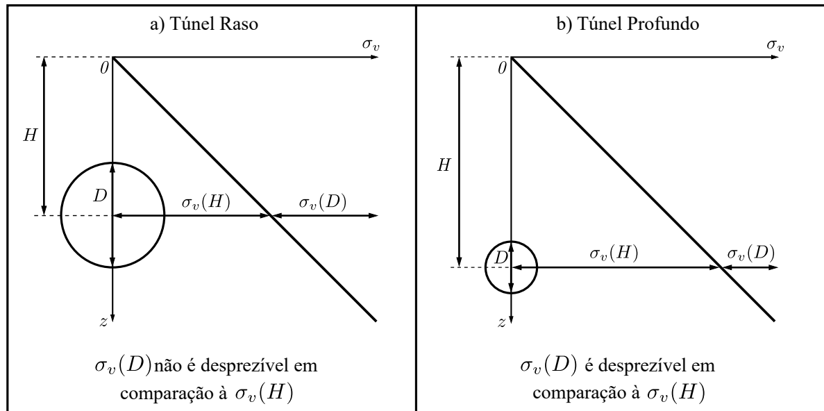
Figura 2.17 – Variação da tensão vertical (adaptado de ??)
