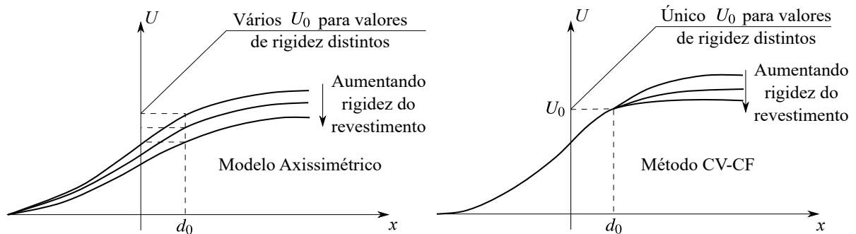
Figura 2.24 – Influência da rigidez do revestimento no perfil de convergências e no parâmetro U_0 (adaptado de ??)
