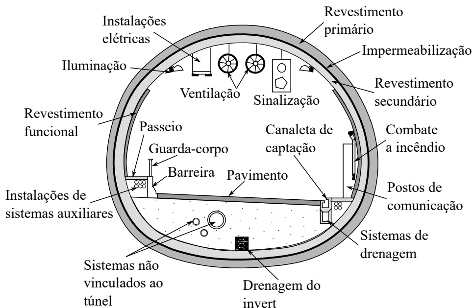
Figura 2.10 – Elementos de revestimento de túnel rodoviário (adaptado de ??)
