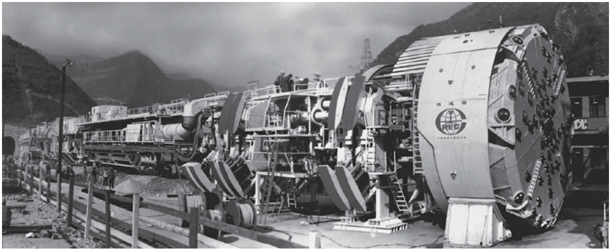
Figura 2.7 – Tuneladora com múltiplas garras (??)
