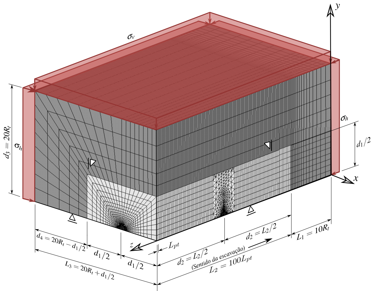
Figura 4.3 – Malha, dimensões e condições de contorno do domínio dos túneis gêmeos tridimensionais (adaptado de ??)
