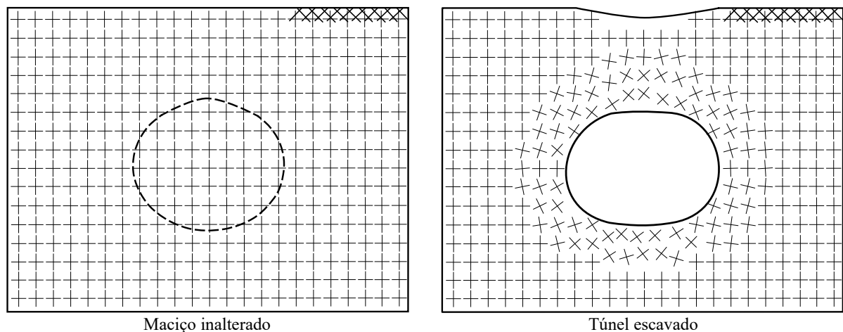
Figura 2.13 – Direções das tensões principais (adaptado de ??)
