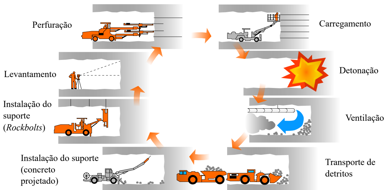
Figura 2.6 – Sequência executiva do método de construção por perfuração e detonação (adaptado de ??)
