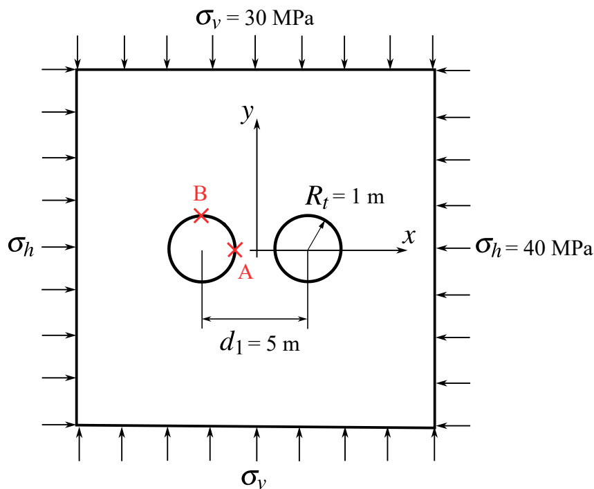
Figura 4.11 – Geometria e carregamento dos túneis gêmeos estudados por ??)
