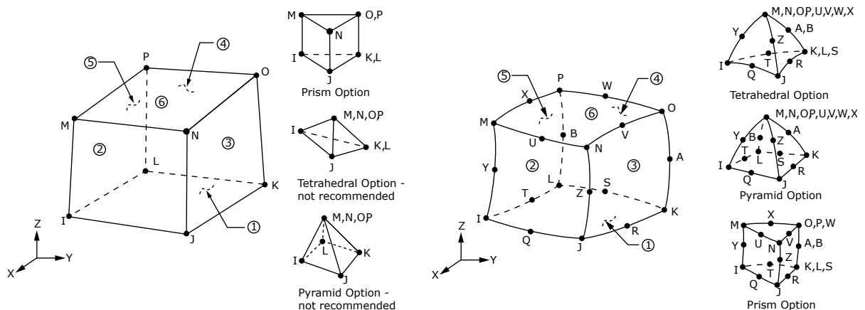
Figura 4.2 – Elementos SOLID 185 e SOLID 186 (??)
