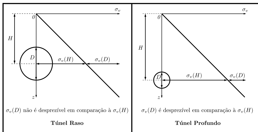
Figura 2.2 – Distinção entre túnel raso e profundo (fonte: adaptado de Benamar (fazer a citação))
