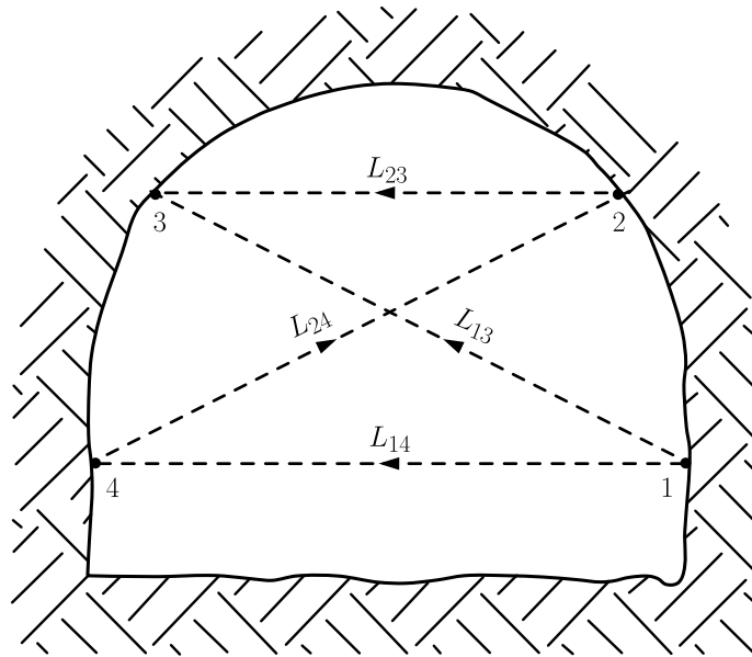
Figura 2.9 – Seção de medição de convergência em quatro direções (fonte: adaptado de Panet (1985) (fazer a citação))
