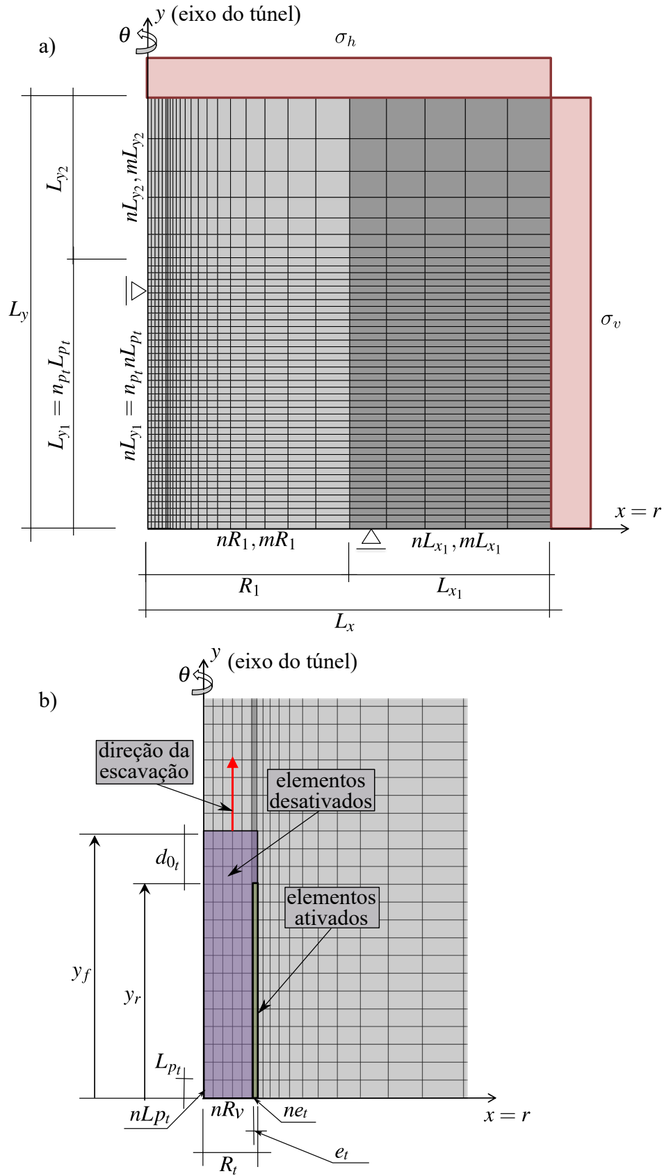
Figura 4.1 – a) Domínio, condições de contorno e parâmetros geométricos do modelo axisimétrico (b) Detalhe dos parâmetros que envolvem a escavação (adaptado de Quevedo (2021))
