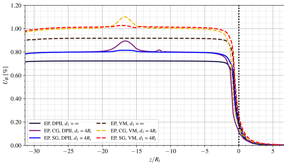
Figura 4.13 – Perfis de convergência dos túneis gêmeos para maciço elastoplástico e com revestimento elástico
