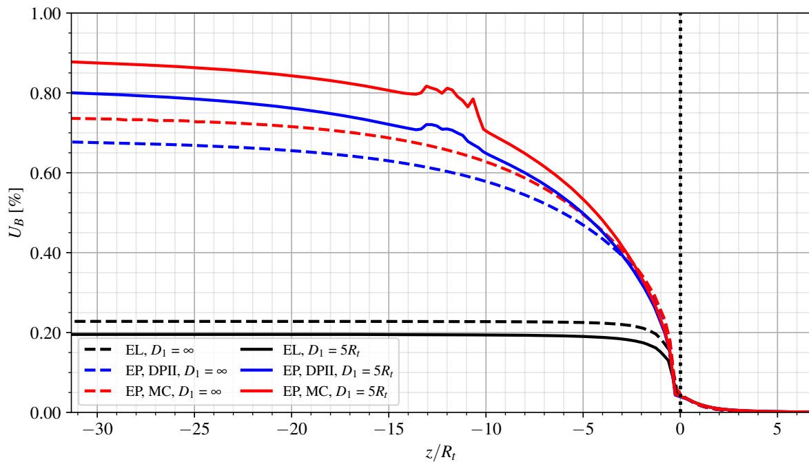
Figura 4.12 – Perfis de convergência no ponto B
