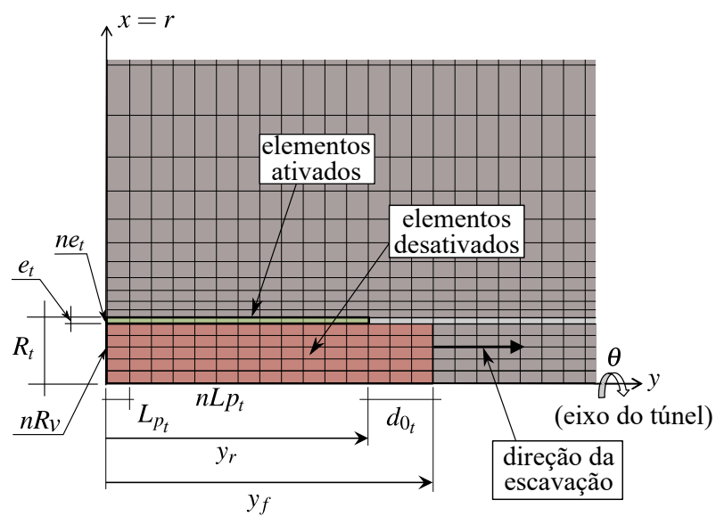
Figura 5.2 – Detalhe dos parâmetros que envolvem a escavação e colocação do revestimento
