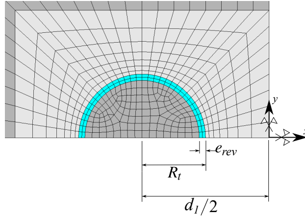
Figura 4.4 – Detalhes do túnel longitudinal (adaptado de Colombo (2023))
