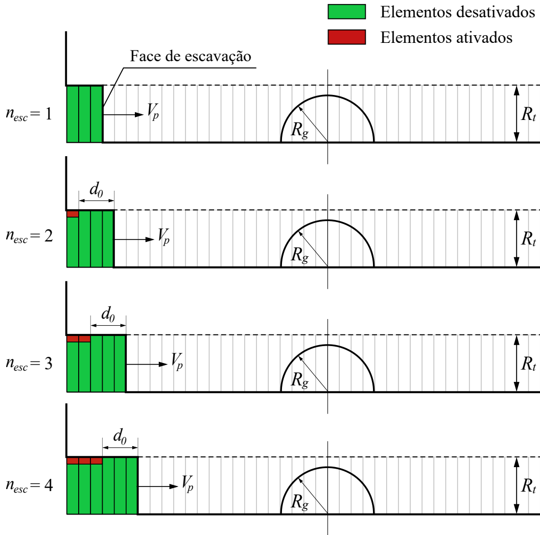
Figura 2.23 – Representação esquemática do processo de escavação (adaptado de Colombo (2023))
