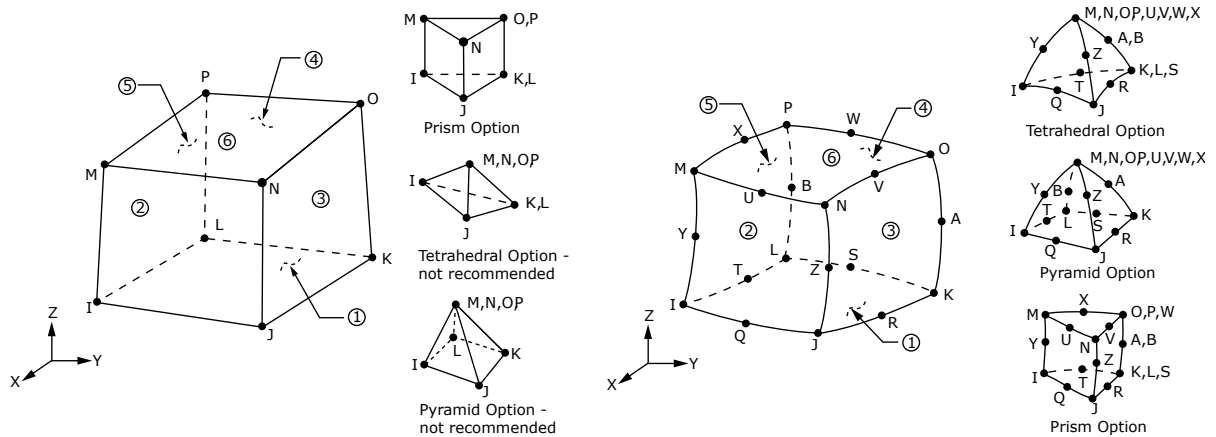
Figura 4.2 – Elementos SOLID 185 e SOLID 186 (ANSYS Inc, 2024)
