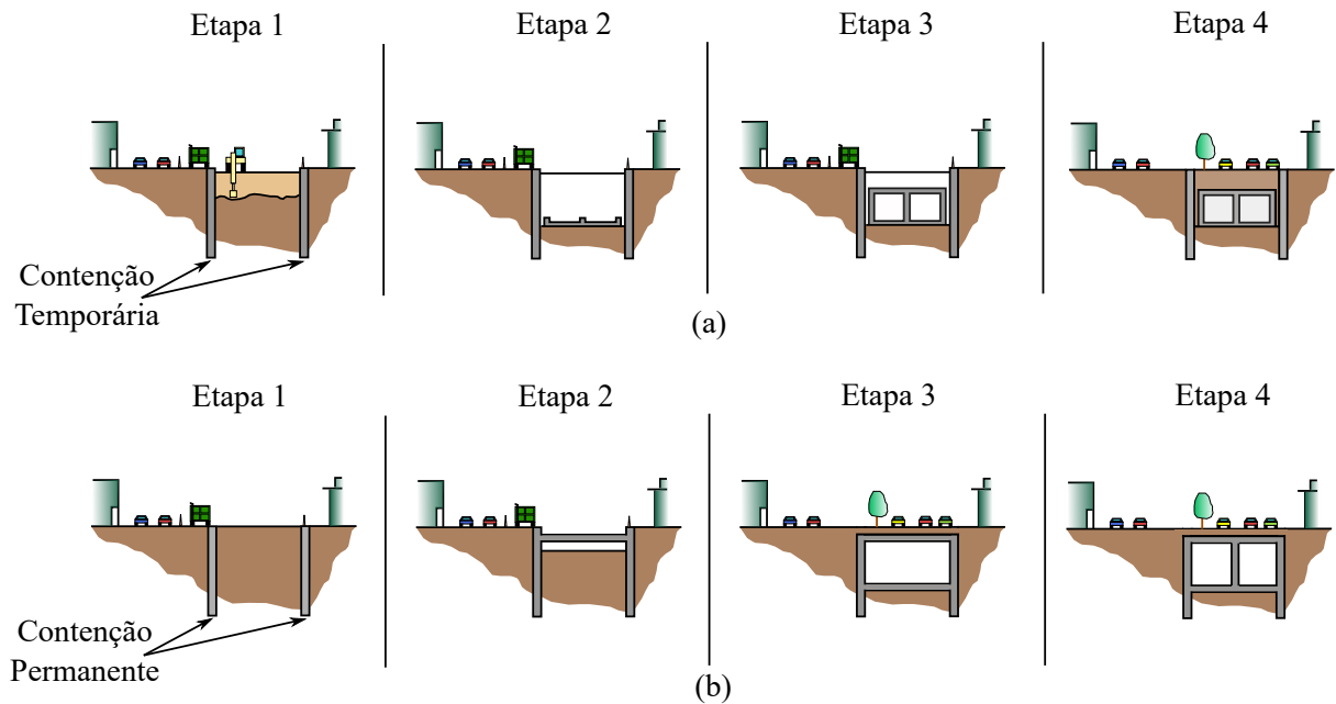
Figura 2.3 – Método de escavação vala recoberta. a) cut and cover e b) cover and cut (adaptado de ??)
