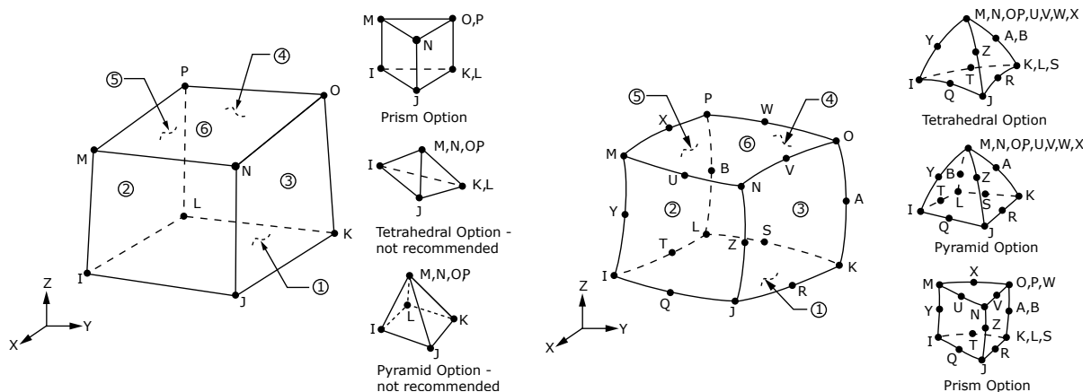
Figura 5.3 – Elementos SOLID185 e SOLID186 (ANSYS Inc, 2024)
