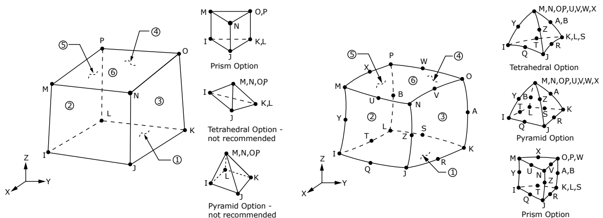
Figura 5.3 – Elementos SOLID185 e SOLID186 (ANSYS Inc, 2024)
