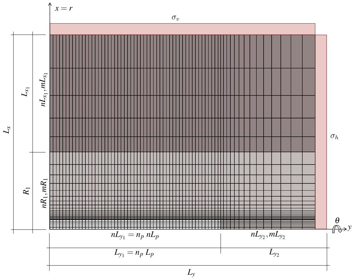
Figura 5.1 – Domínio, condições de contorno e parâmetros geométricos do modelo axissimétrico
