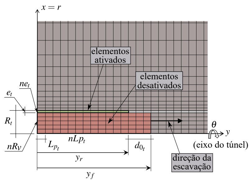
Figura 5.2 – Detalhe dos parâmetros que envolvem a escavação e colocação do revestimento
