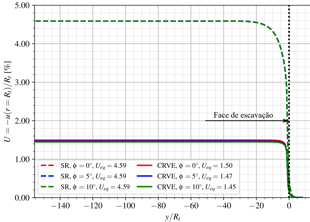
Figura 6.4 – Perfis de convergência no longo prazo - túnel isolado sem revestimento (SR) e com revestimento viscoelástico (CRVE)
