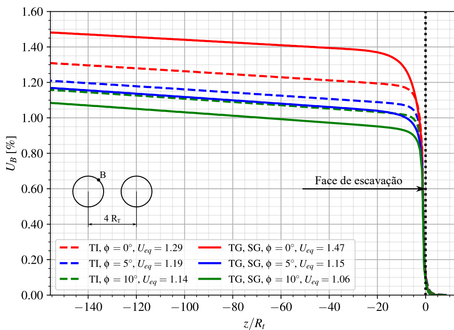
Figura A.3 – Perfis de convergência - Ponto B - túnel isolado (TI) e túneis gêmeos (TG) sem revestimento (SR) no final da construção
