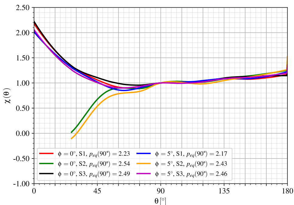
Figura 8.10 – Pressões no revestimento - túneis gêmeos com galeria transversal e revestimento elástico (CRE) no final da construção
