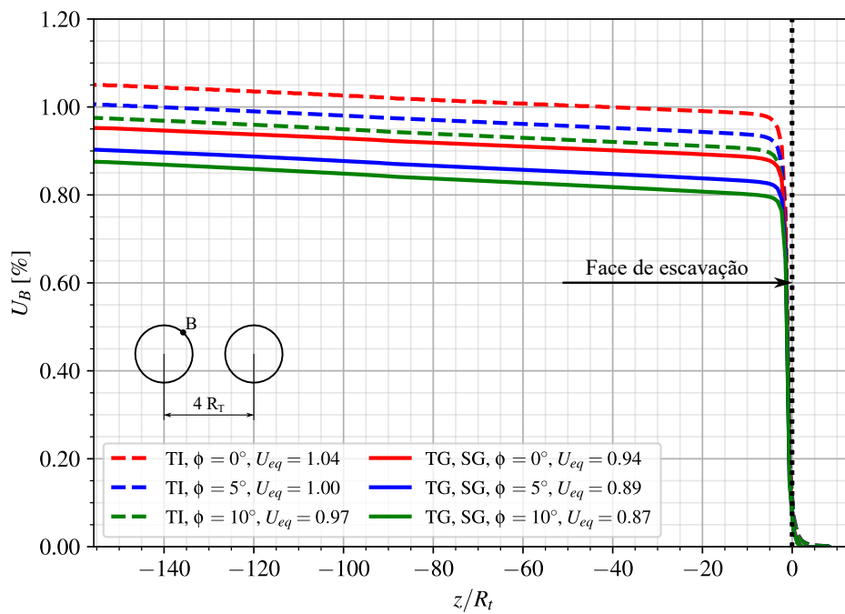
Figura A.11 – Perfis de convergência - Ponto B - túnel isolado (TI) e túneis gêmeos (TG) com revestimento viscoelástico (CRVE) no final da construção
