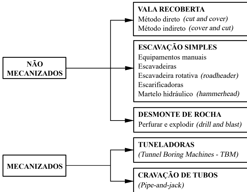
Figura 2.3 – Métodos de escavação de túneis ((QUEVEDO, 2021))
