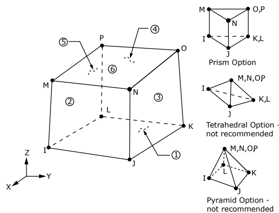
Figura 4.4 – Elemento SOLID185 (ANSYS Inc, 2024)
