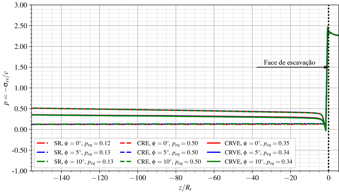
Figura 6.6 – Pressões no revestimento - túnel isolado sem revestimento (SR), com revestimento elástico (CRE) e viscoelástico (CRVE) no final da construção
