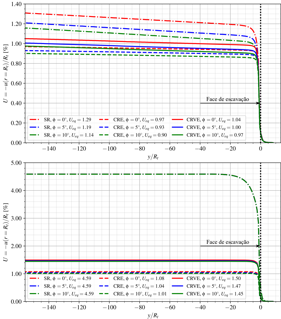
Figura 6.5 – Perfis de convergência - túnel isolado sem revestimento (SR), com revestimento elástico (CRE) e viscoelástico (CRVE). a) Final da construção; b) Longo prazo
