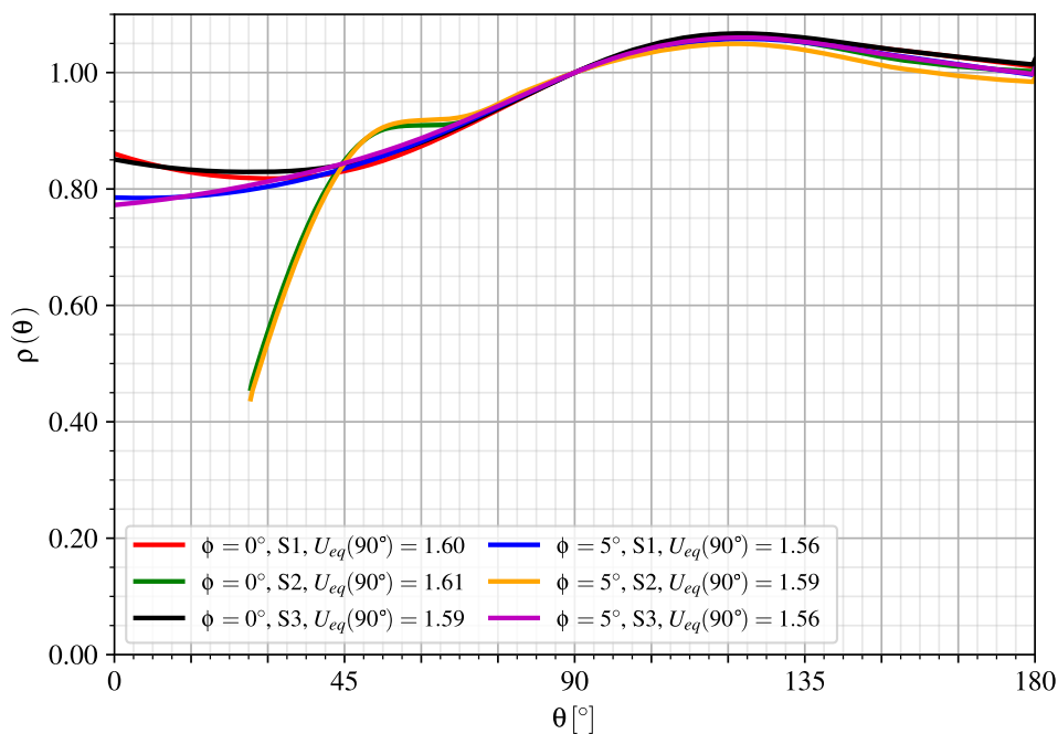
Figura 8.9 – Deformada da seção - túneis gêmeos com galeria transversal e revestimento viscoelástico (CRVE) no longo prazo
