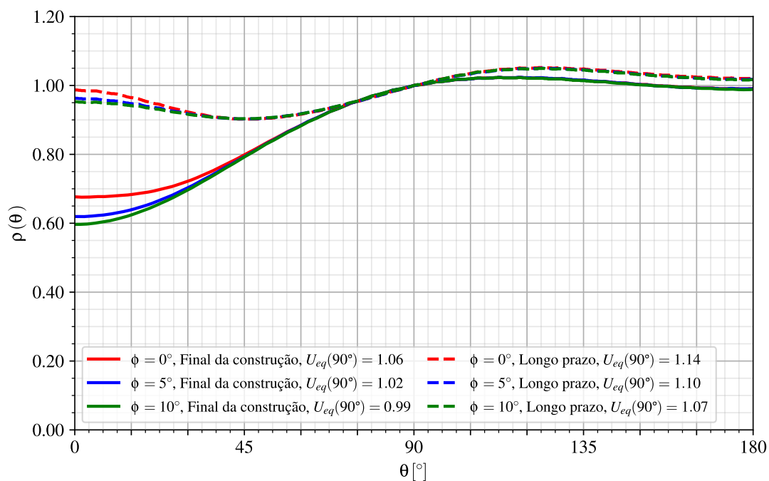
Figura 7.13 – Anisotropia das deformações - túneis gêmeos sem galeria com revestimento elástico (CRE)
