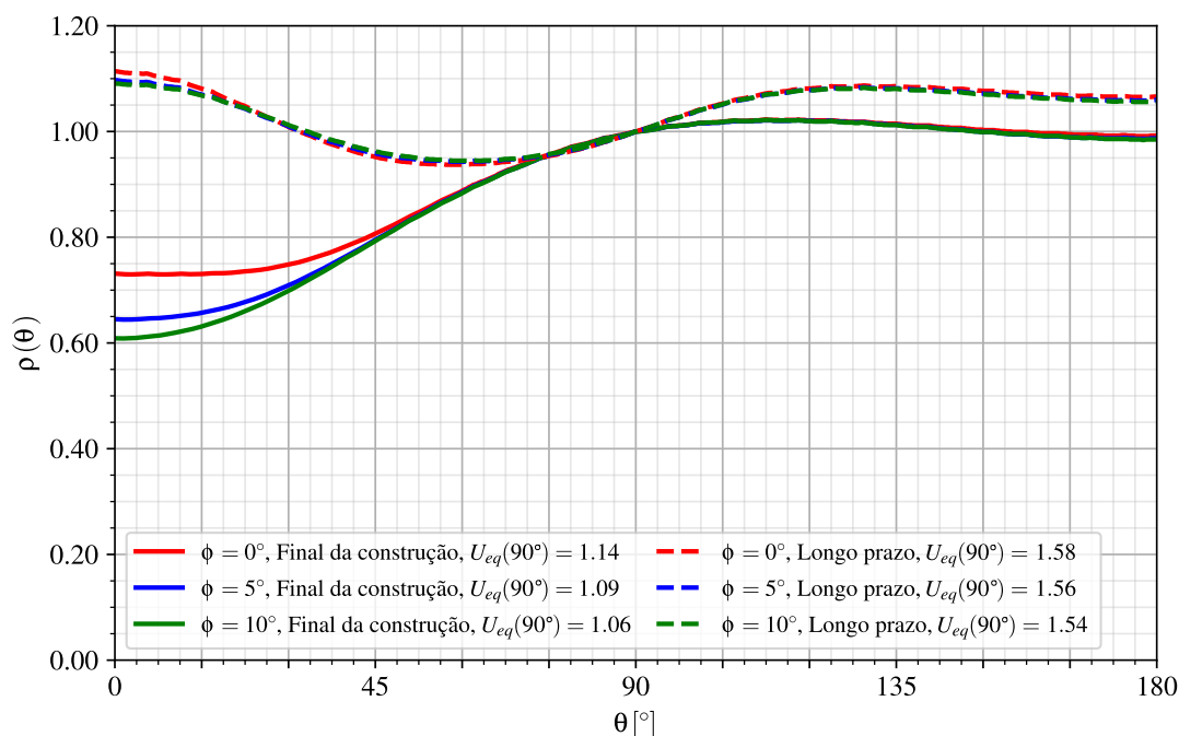
Figura 7.14 – Anisotropia das deformações - túneis gêmeos sem galeria com revestimento viscoelástico (CRVE)
