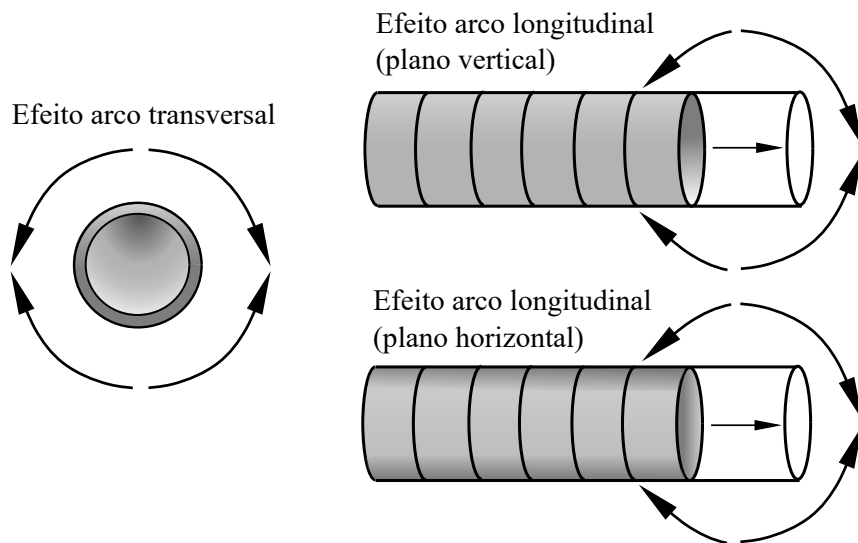
Figura 2.13 – Efeito arco em diferentes planos que interceptam o túnel (adaptado de França (2006))
