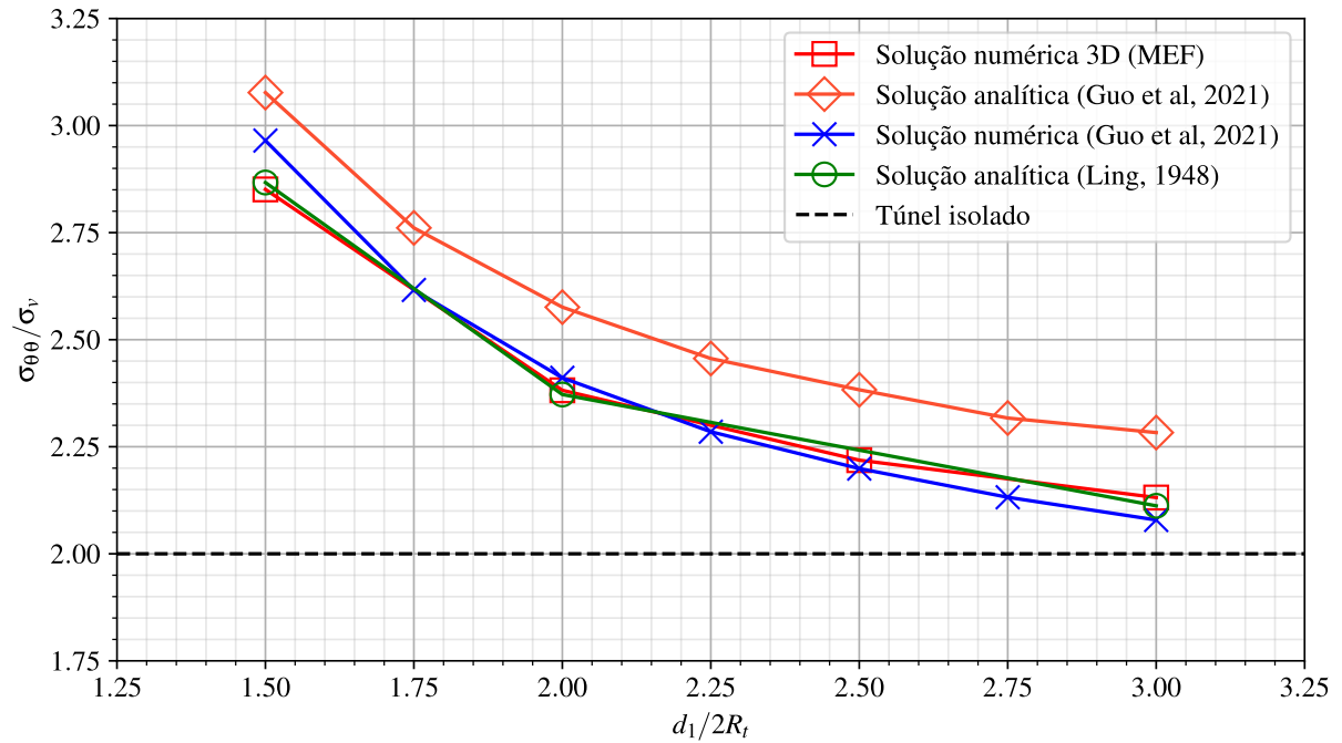
Figura 5.4 – Fator de concentração de tensão tangencial na parede lateral do túnel (ponto A) em função da distância entre os túneis gêmeos
