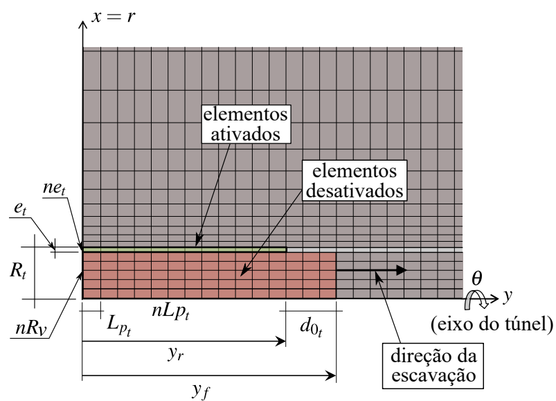
Figura 4.2 – Detalhe dos parâmetros que envolvem a escavação e colocação do revestimento
