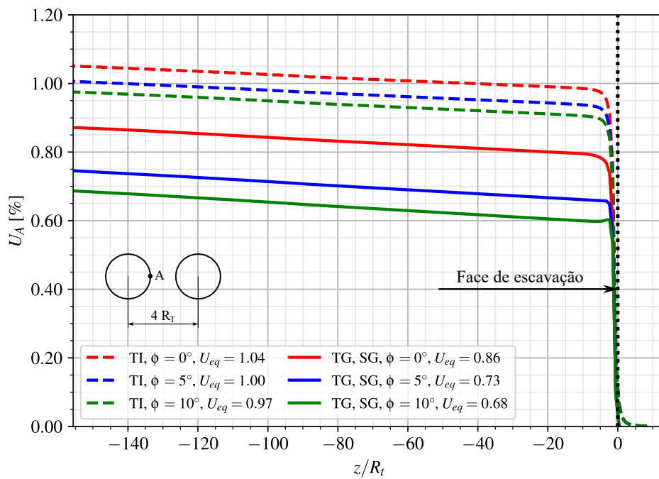
Figura A.9 – Perfis de convergência - Ponto A - túnel isolado (TI) e túneis gêmeos (TG) com revestimento viscoelástico (CRVE) no final da construção
