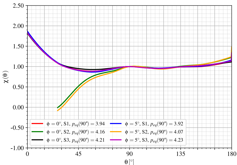
Figura 8.11 – Pressões no revestimento - túneis gêmeos com galeria transversal e revestimento elástico (CRE) no longo prazo
