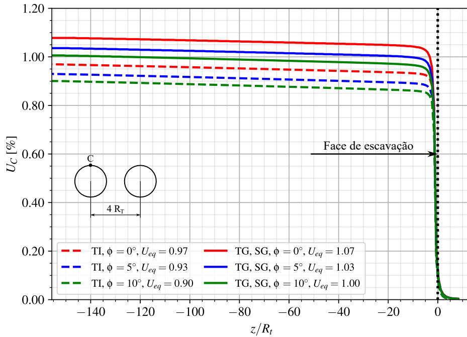
Figura 7.4 – Perfis de convergência - túnel isolado (TI) e túneis gêmeos (TG) sem galeria (SG), com revestimento elástico (CRE) no final da construção
