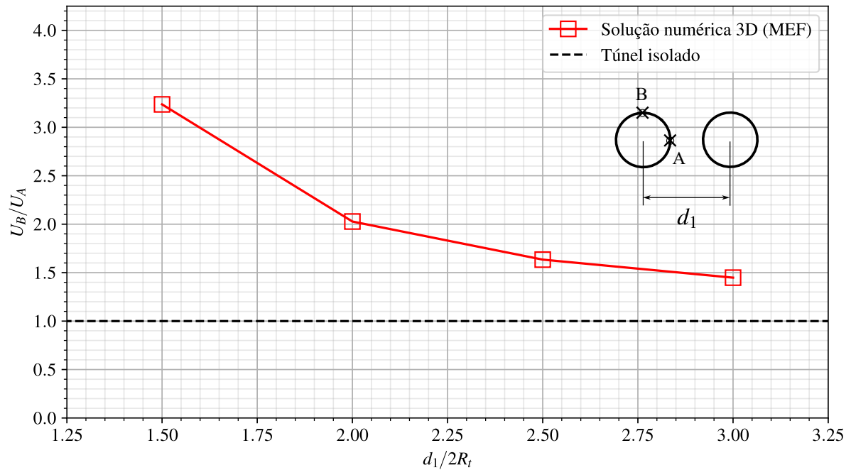
Figura 5.3 – Ilustração da anisotropia de deformação da parede do túnel induzida pela proximidade de túneis gêmeos
