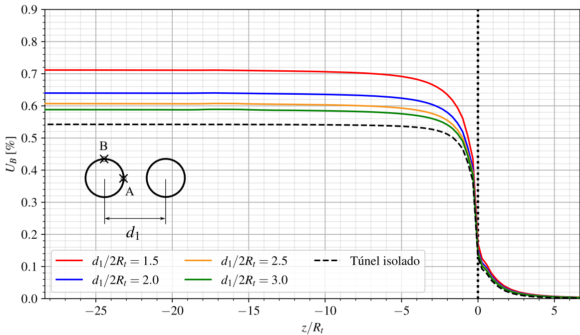
Figura 5.2 – Perfis de convergência no teto do túnel (ponto B)
