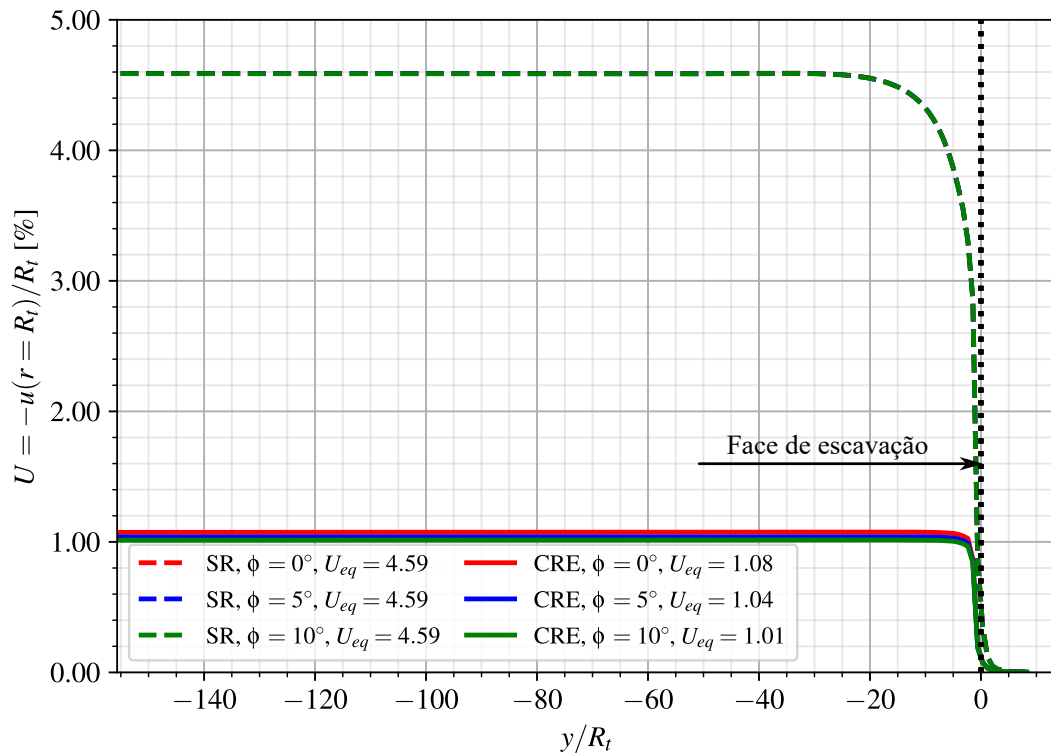
Figura 6.2 – Perfis de convergência no longo prazo - túnel isolado sem revestimento (SR) e com revestimento elástico (CRE)
