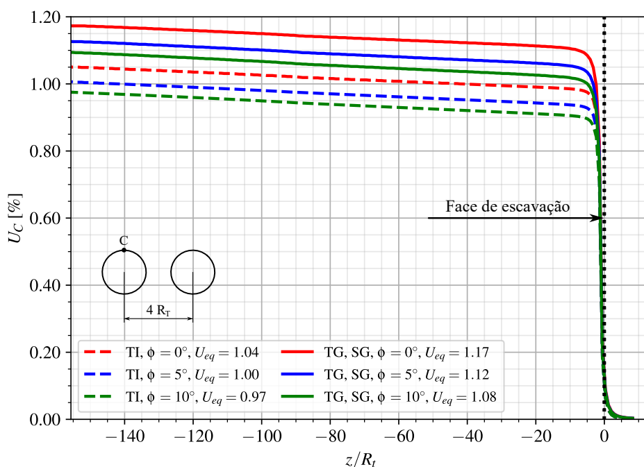
Figura 7.6 – Perfis de convergência - túnel isolado (TI) e túneis gêmeos (TG) sem galeria (SG), com revestimento viscoelástico (CRVE) no final da construção
