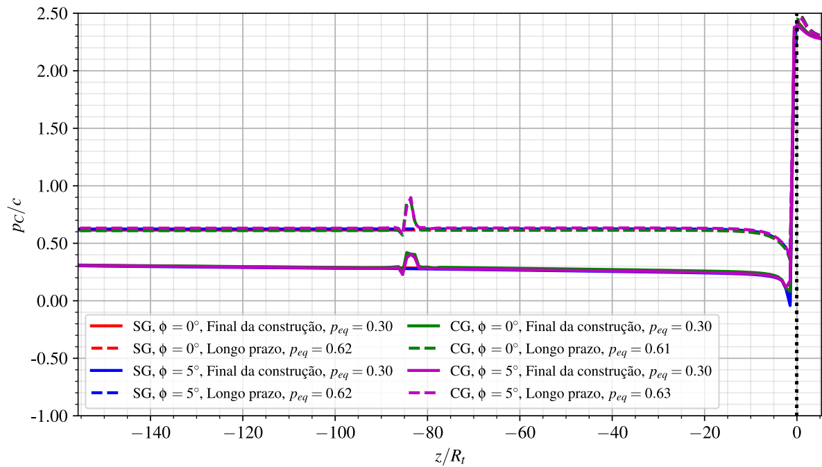
Figura 8.4 – Pressões no revestimento - túneis gêmeos sem galeria (SG) e com galeria (CG) com revestimento viscoelástico (CRVE)
