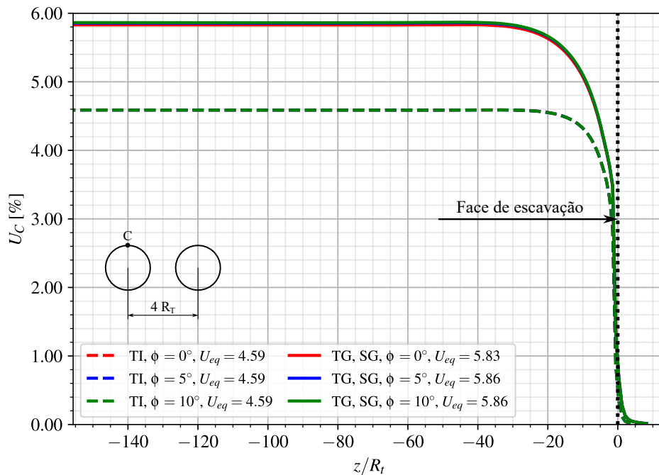
Figura 7.3 – Perfis de convergência - túnel isolado (TI) e túneis gêmeos (TG) sem galeria (SG) e sem revestimento (SR) no longo prazo
