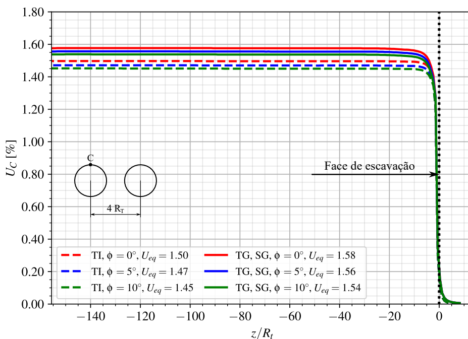
Figura 7.7 – Perfis de convergência - túnel isolado (TI) e túneis gêmeos (TG) sem galeria (SG), com revestimento viscoelástico (CRVE) no longo prazo
