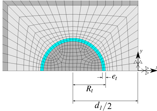
Figura 4.7 – Detalhe da malha de elementos finitos na seção transversal do túnel longitudinal (adaptado de Colombo (2023))
