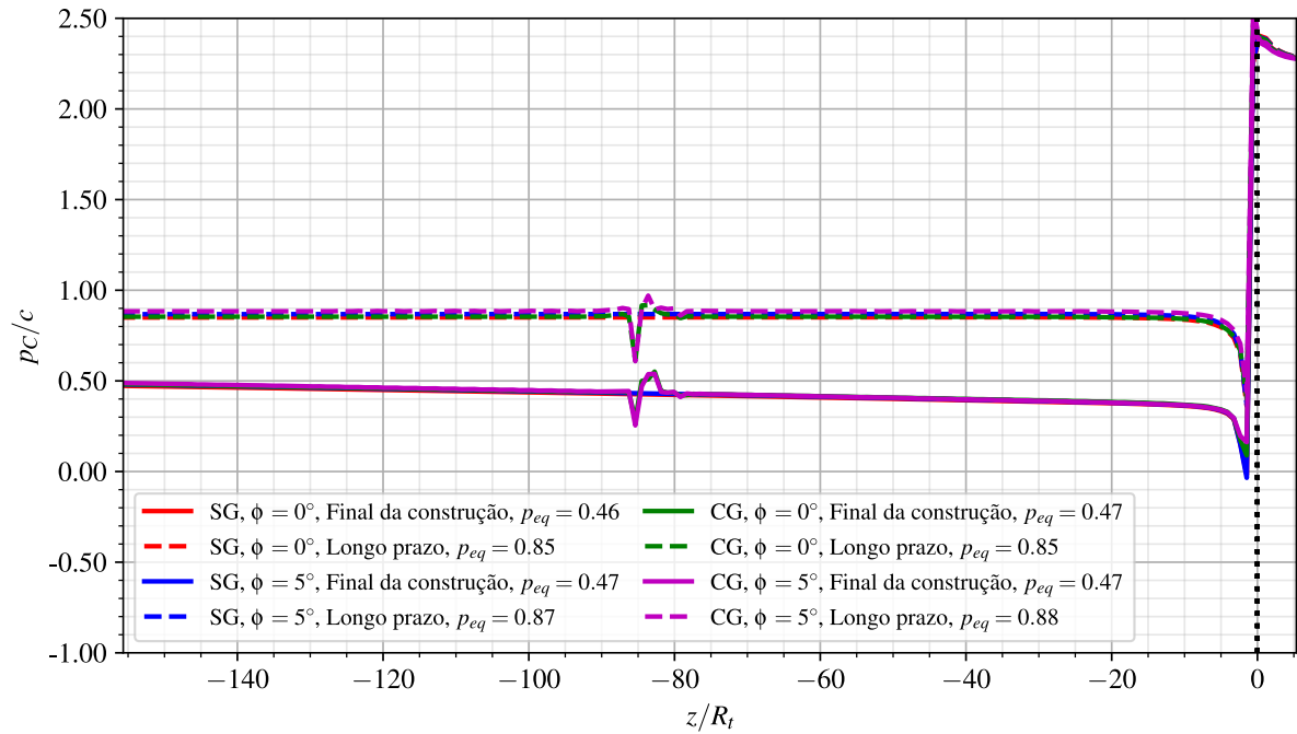
Figura 8.3 – Pressões no revestimento - túneis gêmeos sem galeria (SG) e com galeria (CG) com revestimento elástico (CRE)
