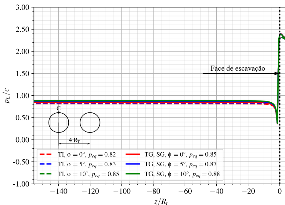
Figura 7.9 – Pressões no revestimento - túnel isolado (TI) e túneis gêmeos (TG) sem galeria (SG) com revestimento elástico (CRE) no longo prazo
