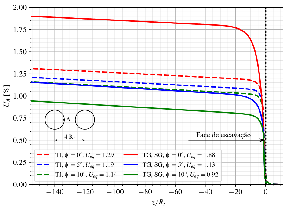
Figura A.1 – Perfis de convergência - Ponto A - túnel isolado (TI) e túneis gêmeos (TG) sem revestimento (SR) no final da construção
