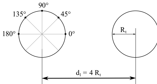
Figura 7.12 – Posições dos ângulos \theta no contorno da seção transversal do túnel
