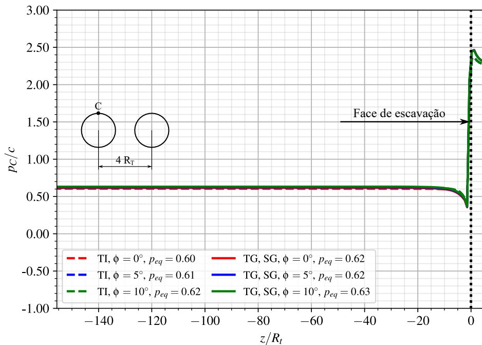
Figura 7.11 – Pressões no revestimento - túnel isolado (TI) e túneis gêmeos (TG) sem galeria (SG) com revestimento viscoelástico (CRVE) no longo prazo
