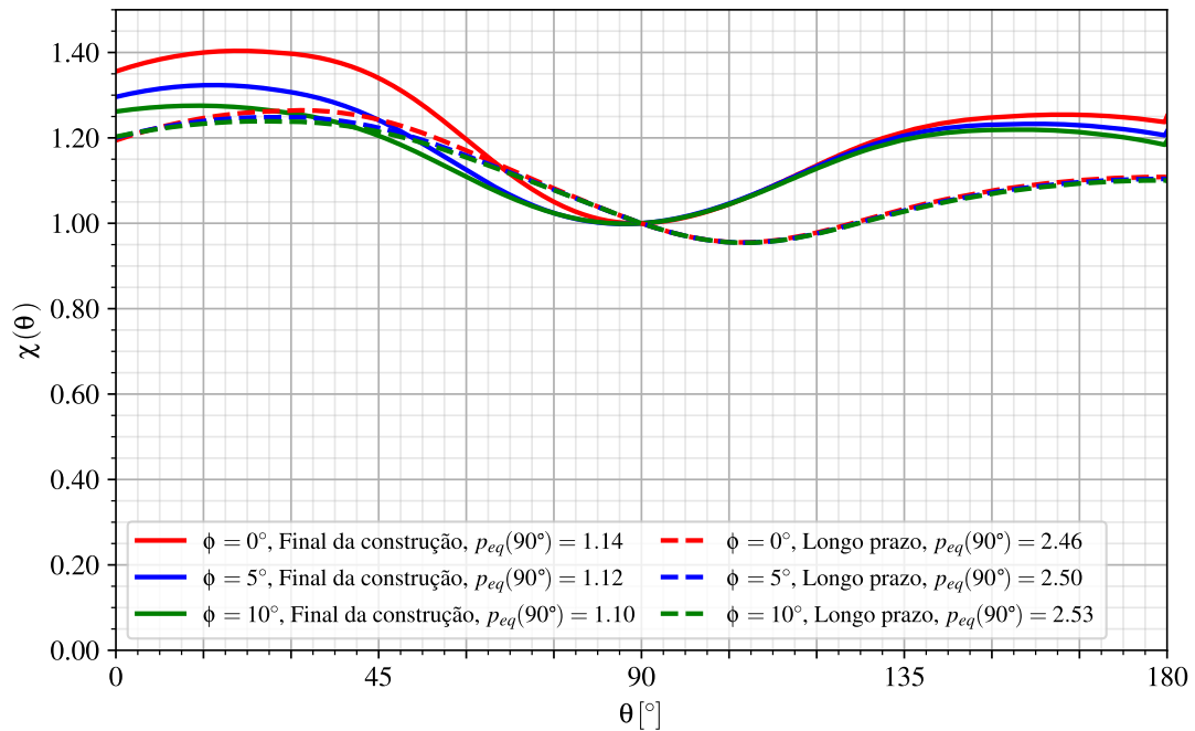
Figura 7.16 – Anisotropia das pressões no revestimento - túneis gêmeos sem galeria com revestimento viscoelástico (CRVE)
