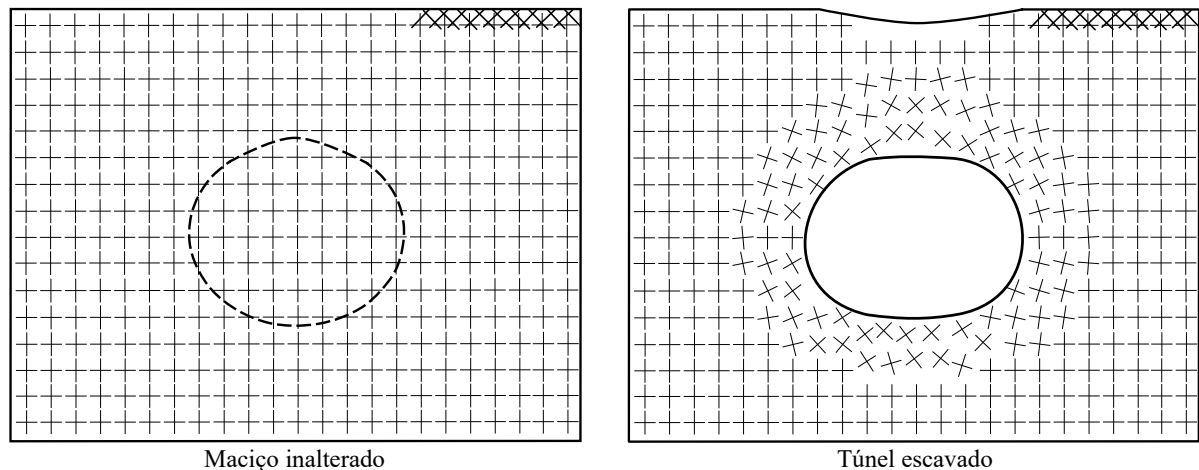
Figura 2.12 – Direções das tensões principais (adaptado de França (2006))
