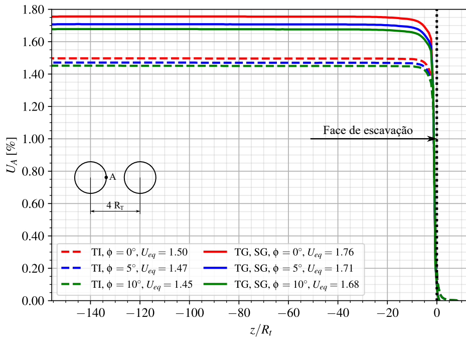
Figura A.10 – Perfis de convergência - Ponto A - túnel isolado (TI) e túneis gêmeos (TG) com revestimento viscoelástico (CRVE) no longo prazo
