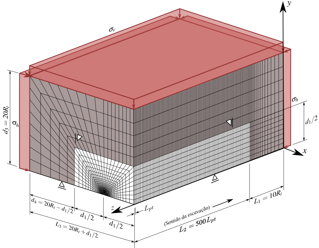
Figura 4.6 – Malha, dimensões e condições de contorno do domínio dos túneis gêmeos sem galeria (adaptado de Colombo (2023))
