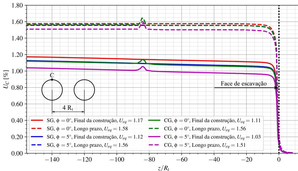
Figura 8.2 – Perfis de convergência - túneis gêmeos sem galeria (SG) e com galeria (CG) com revestimento viscoelástico (CRVE)
