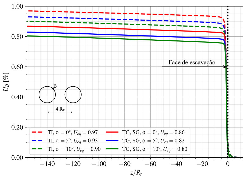
Figura A.7 – Perfis de convergência - Ponto B - túnel isolado (TI) e túneis gêmeos (TG) com revestimento elástico (CRE) no final da construção
