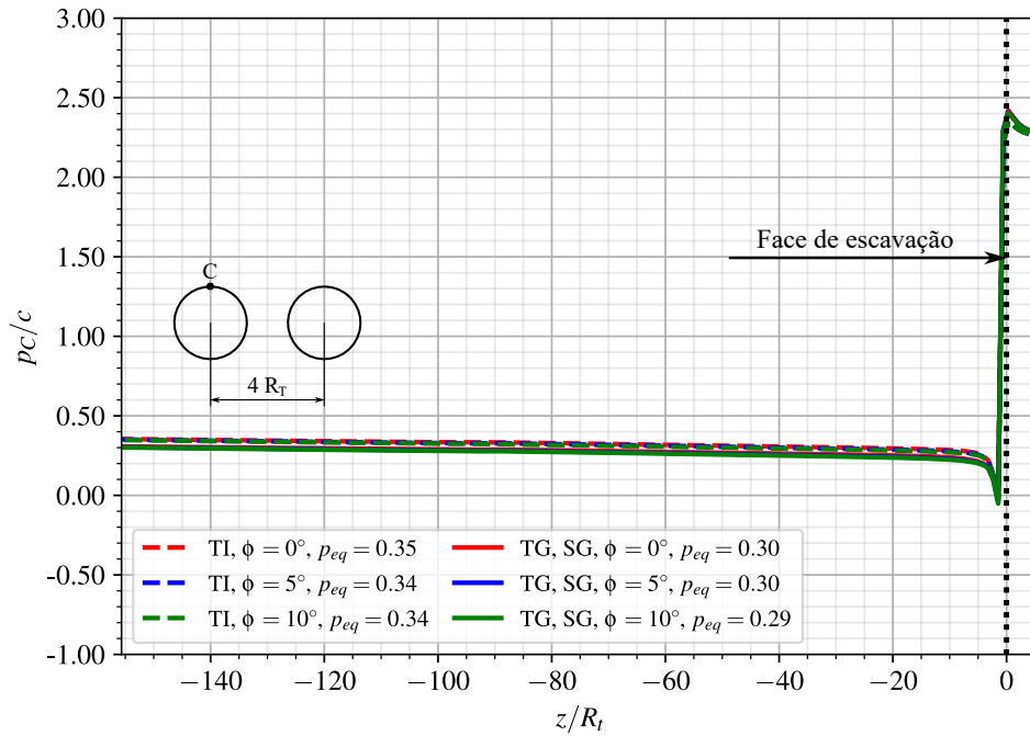
Figura 7.10 – Pressões no revestimento - túnel isolado (TI) e túneis gêmeos (TG) sem galeria (SG) com revestimento viscoelástico (CRVE) no final da construção
