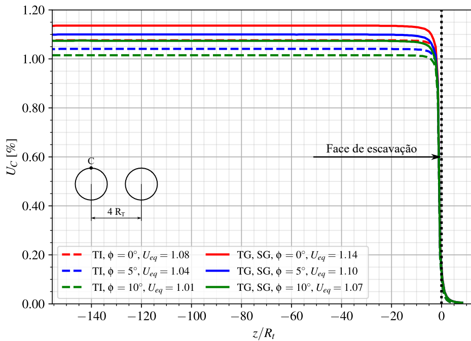
Figura 7.5 – Perfis de convergência - túnel isolado (TI) e túneis gêmeos (TG) sem galeria (SG), com revestimento elástico (CRE) no longo prazo
