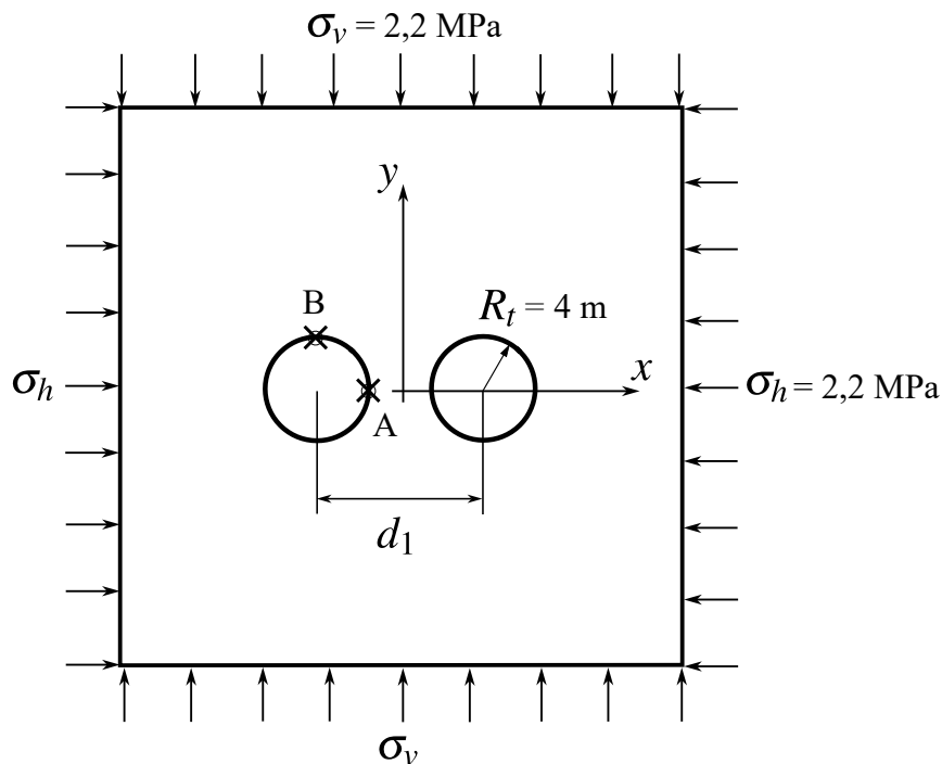
Figura 5.1 – Geometria e carregamento dos túneis gêmeos estudados por Guo et al. (2021))
