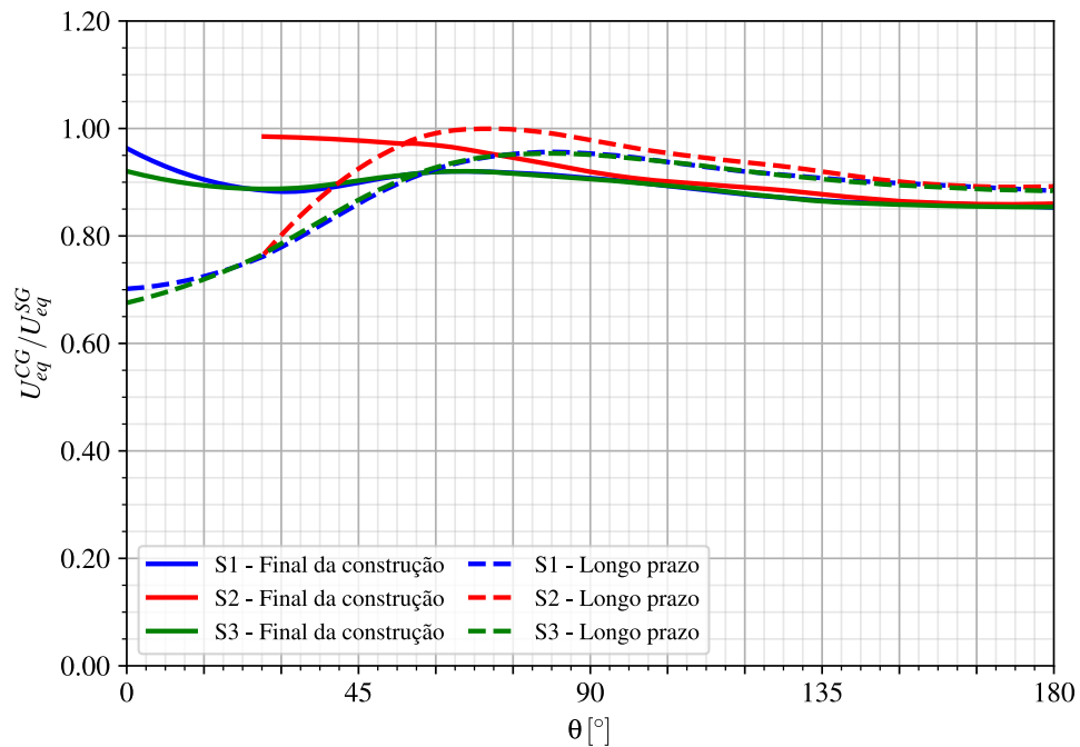
Figura 8.15 – Razão entre túneis gêmeos com galeria e sem galeria, com revestimento elástico (CRE) e \phi = 5^\circ
