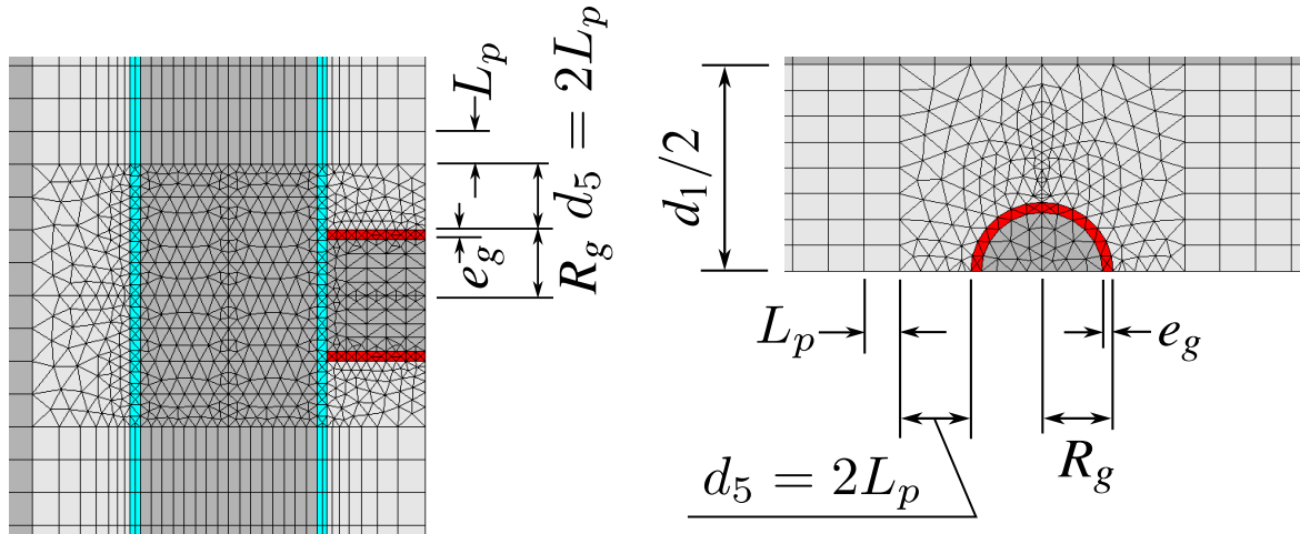
Figura 4.8 – Detalhamento da galeria transversal. Esquerda: vista da região de encontro entre o túnel longitudinal e a galeria no plano de simetria y = 0 ; Direita: detalhe da malha de elementos finitos na seção transversal da galeria. Adaptado de Colombo (2023)
