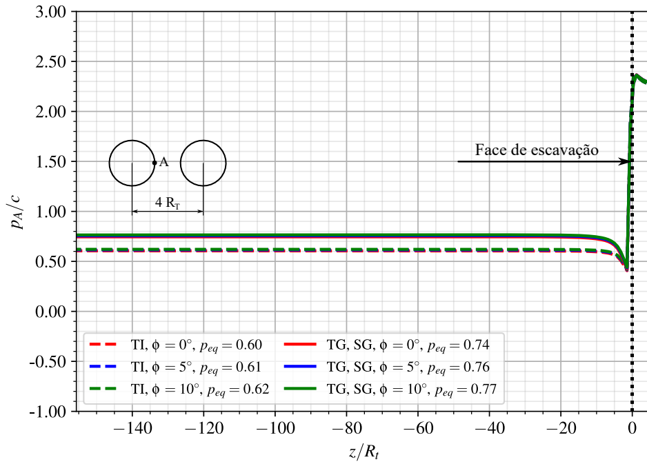
Figura A.22 – Perfis de convergência - Ponto A - túnel isolado (TI) e túneis gêmeos (TG) com revestimento viscoelástico (CRVE) no longo prazo
