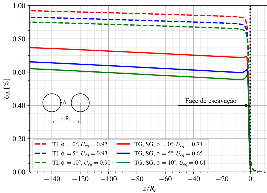
Figura A.5 – Perfis de convergência - Ponto A - túnel isolado (TI) e túneis gêmeos (TG) com revestimento elástico (CRE) no final da construção
