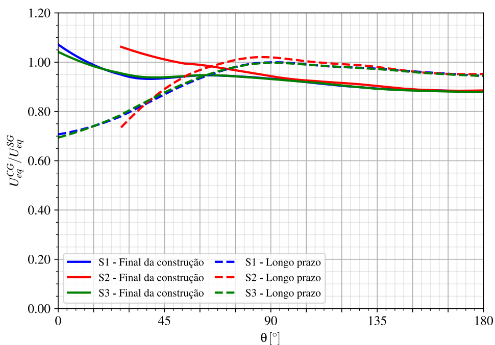
Figura 8.17 – Razão entre túneis gêmeos com galeria e sem galeria, com revestimento viscoelástico (CRVE) e \phi = 5^\circ
