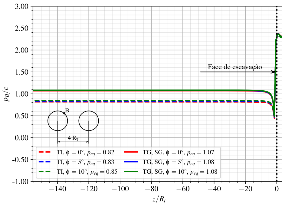
Figura A.20 – Perfis de convergência - Ponto B - túnel isolado (TI) e túneis gêmeos (TG) com revestimento elástico (CRE) no longo prazo
