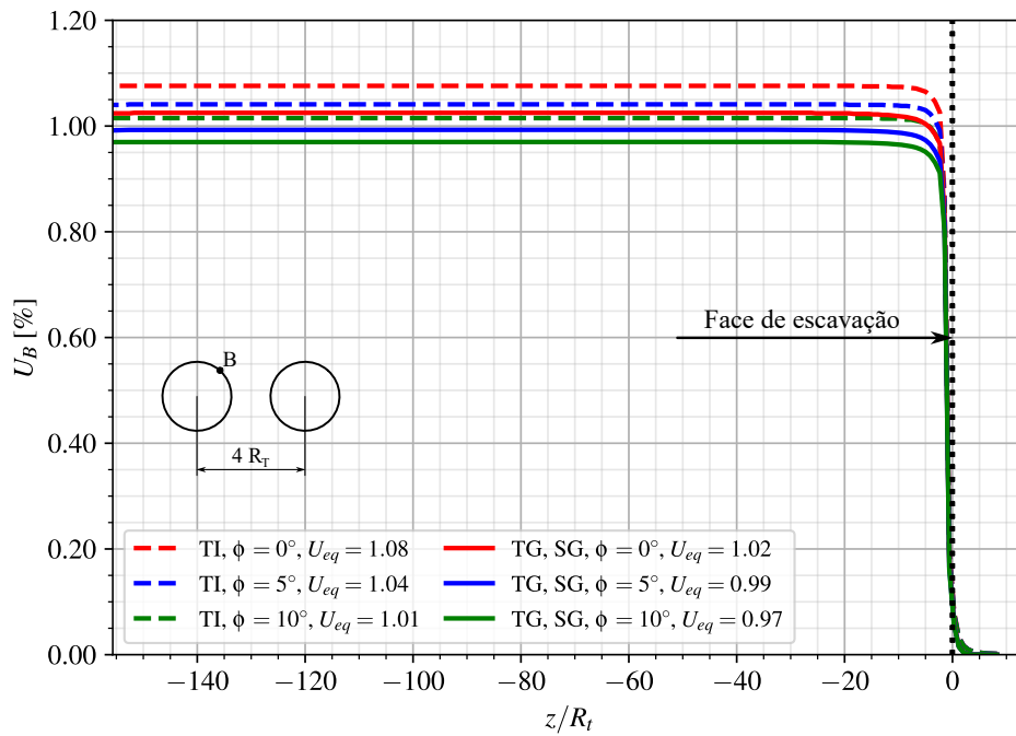
Figura A.8 – Perfis de convergência - Ponto B - túnel isolado (TI) e túneis gêmeos (TG) com revestimento elástico (CRE) no longo prazo
