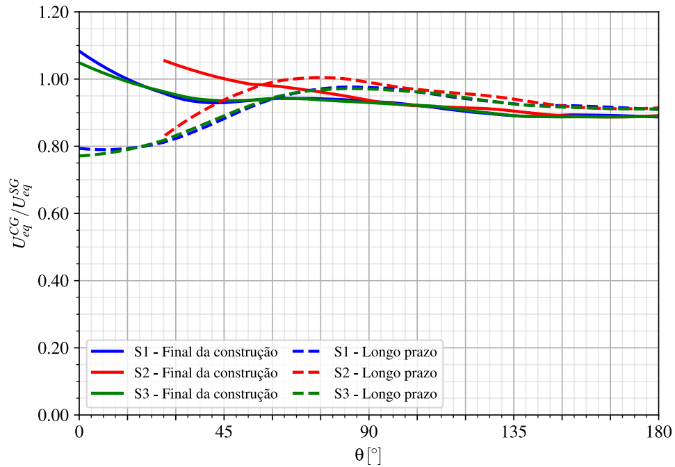
Figura 8.14 – Razão entre túneis gêmeos com galeria e sem galeria, com revestimento elástico (CRE) e \phi = 0^\circ
