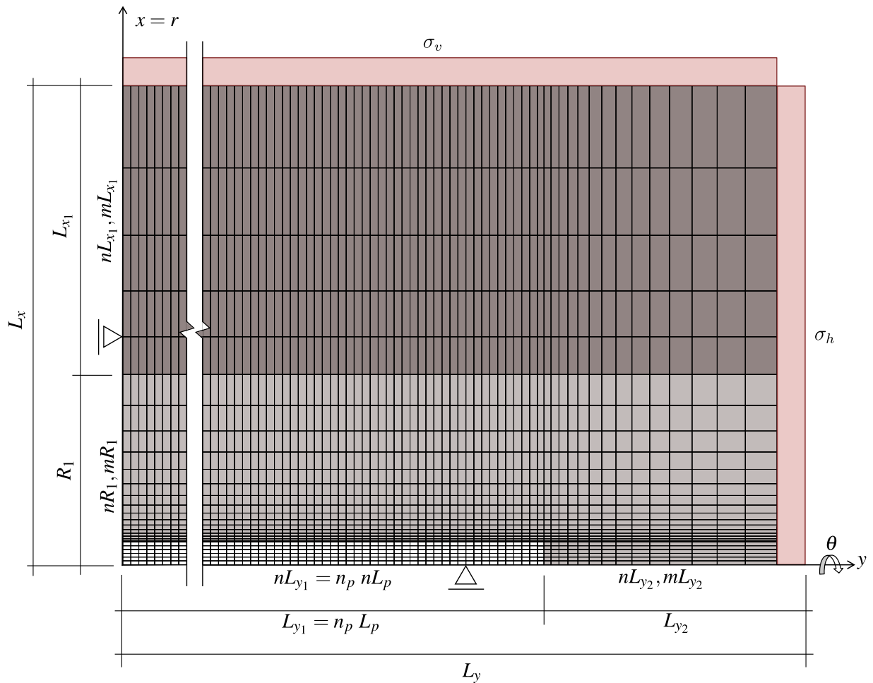
Figura 4.1 – Discretização do domínio, condições de contorno e parâmetros geométricos do modelo axissimétrico
