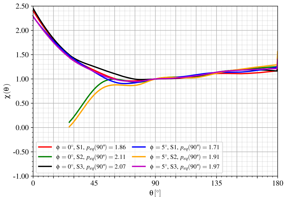
Figura 8.12 – Pressões no revestimento - túneis gêmeos com galeria transversal e revestimento viscoelástico (CRVE) no final da construção
