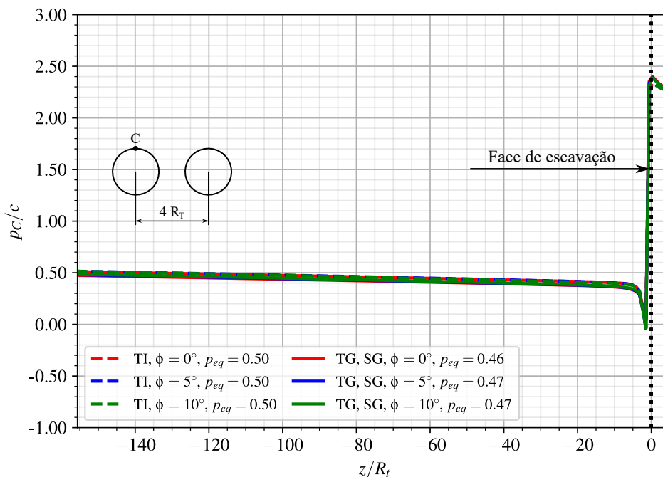
Figura 7.8 – Pressões no revestimento - túnel isolado (TI) e túneis gêmeos (TG) sem galeria (SG) com revestimento elástico (CRE) no final da construção
