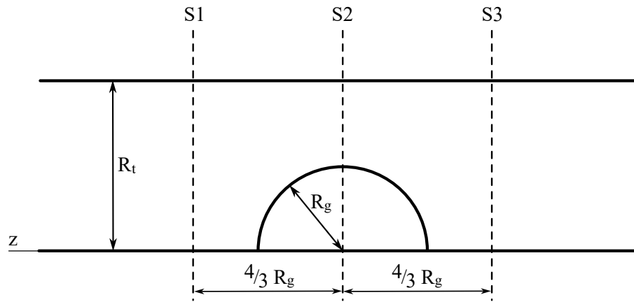
Figura 8.5 – Esquema de representação das seções de análise
