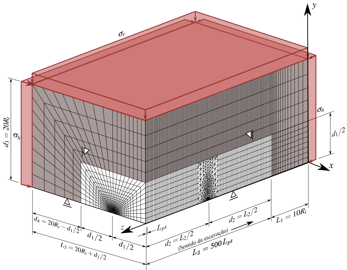
Figura 4.5 – Malha, dimensões e condições de contorno do domínio dos túneis gêmeos com galeria (adaptado de Colombo (2023))
