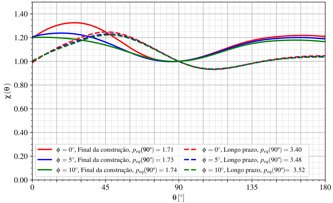
Figura 7.15 – Anisotropia das pressões no revestimento - túneis gêmeos sem galeria com revestimento elástico (CRE)
