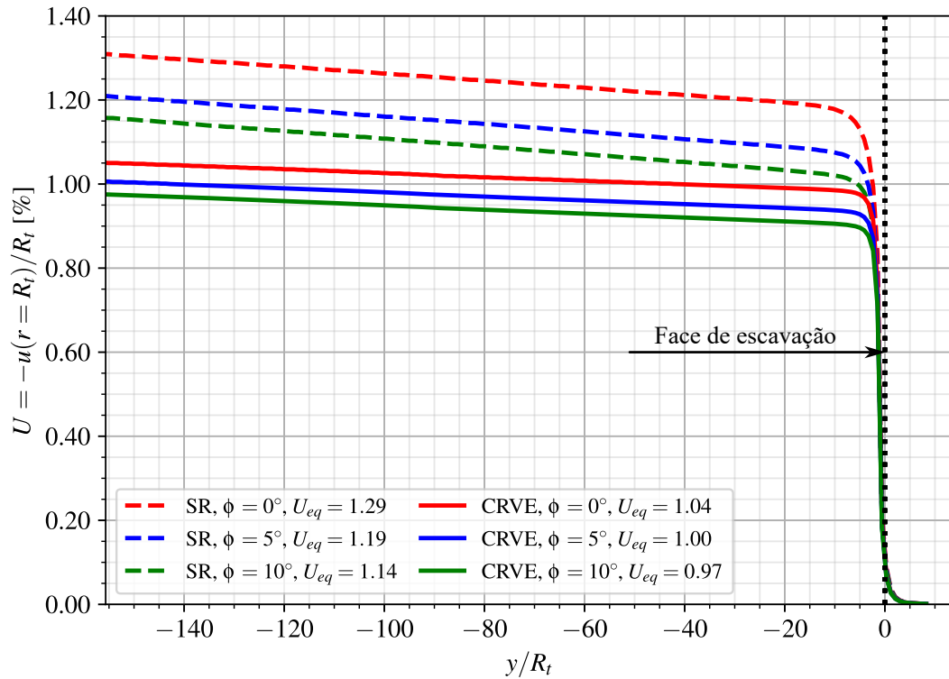
Figura 6.3 – Perfis de convergência ao final da construção - túnel isolado sem revestimento (SR) e com revestimento viscoelástico (CRVE)
