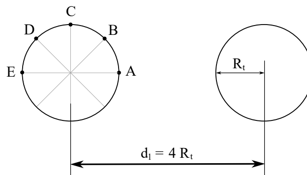
Figura 7.1 – Representação dos pontos de análise dos túneis gêmeos
