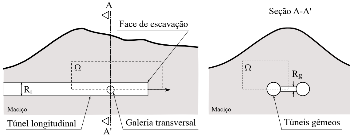
Figura 4.3 – Representação esquemática do domínio \Omega para a problemática de túneis gêmeos com galeria
