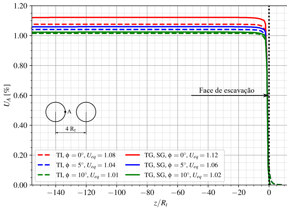
Figura A.6 – Perfis de convergência - Ponto A - túnel isolado (TI) e túneis gêmeos (TG) com revestimento elástico (CRE) no longo prazo
