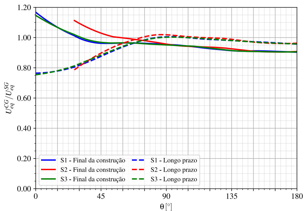
Figura 8.16 – Razão entre túneis gêmeos com galeria e sem galeria, com revestimento viscoelástico (CRVE) e \phi = 0^\circ
