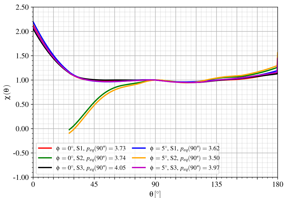
Figura 8.13 – Pressões no revestimento - túneis gêmeos com galeria transversal e revestimento viscoelástico (CRVE) no longo prazo
