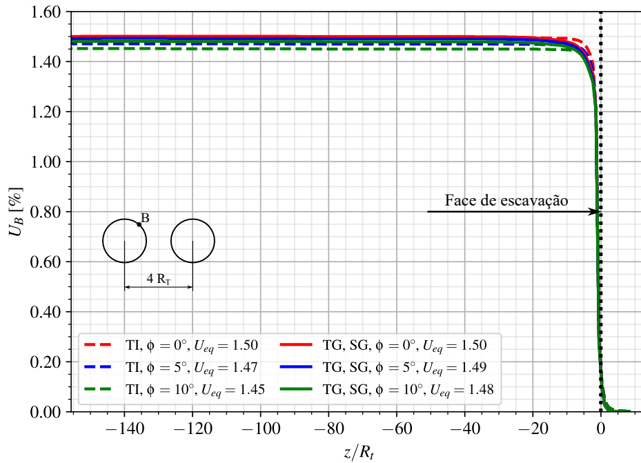
Figura A.12 – Perfis de convergência - Ponto B - túnel isolado (TI) e túneis gêmeos (TG) com revestimento viscoelástico (CRVE) no longo prazo
