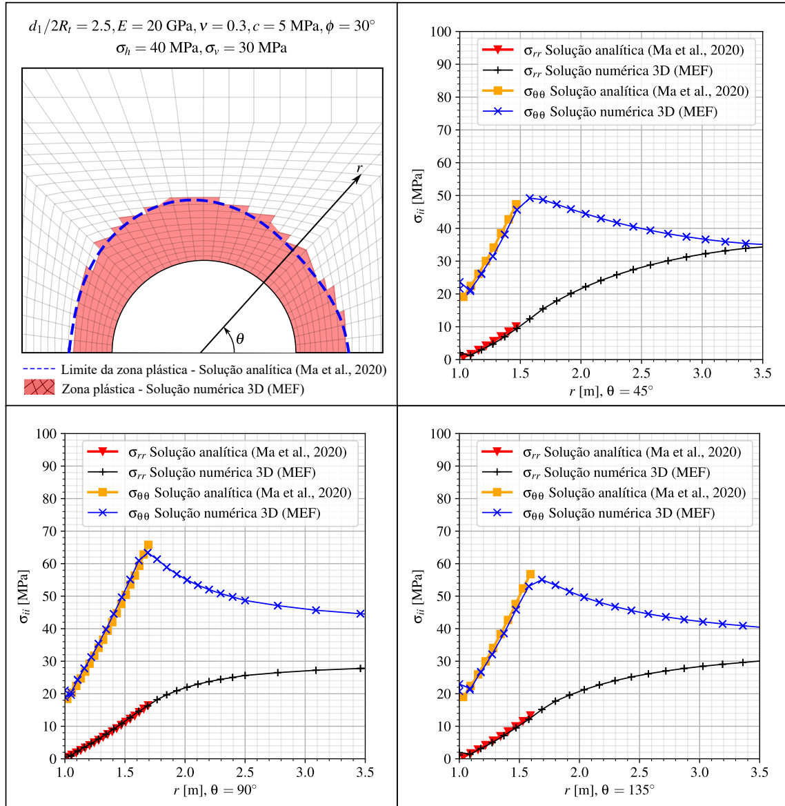
Figura 5.8 – Distribuição dos componentes de tensão radial e ortorradial ao longo de diferentes direções radiais: comparação entre simulações numérica e analítica - critério Mohr-Coulomb
