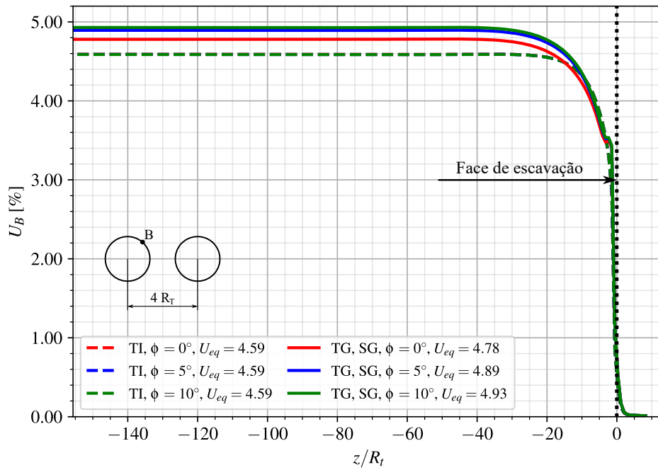
Figura A.4 – Perfis de convergência - Ponto B - túnel isolado (TI) e túneis gêmeos (TG) sem revestimento (SR) no longo prazo
