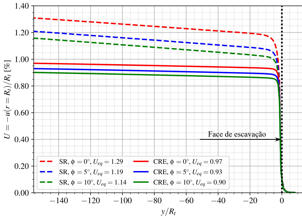
Figura 6.1 – Perfis de convergência ao final da construção - túnel isolado sem revestimento (SR) e com revestimento elástico (CRE)
