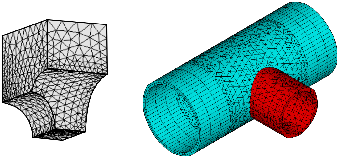
Figura 4.9 – Esquerda: vista isométrica da zona de transição no maciço; Direita: vista isométrica da zona de intersecção do revestimento túnel/galeria. Adaptado de Colombo (2023)
