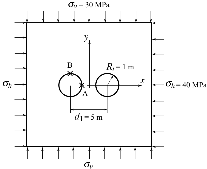
Figura 5.5 – Geometria e carregamento dos túneis gêmeos estudados por Ma et al. (2020))
