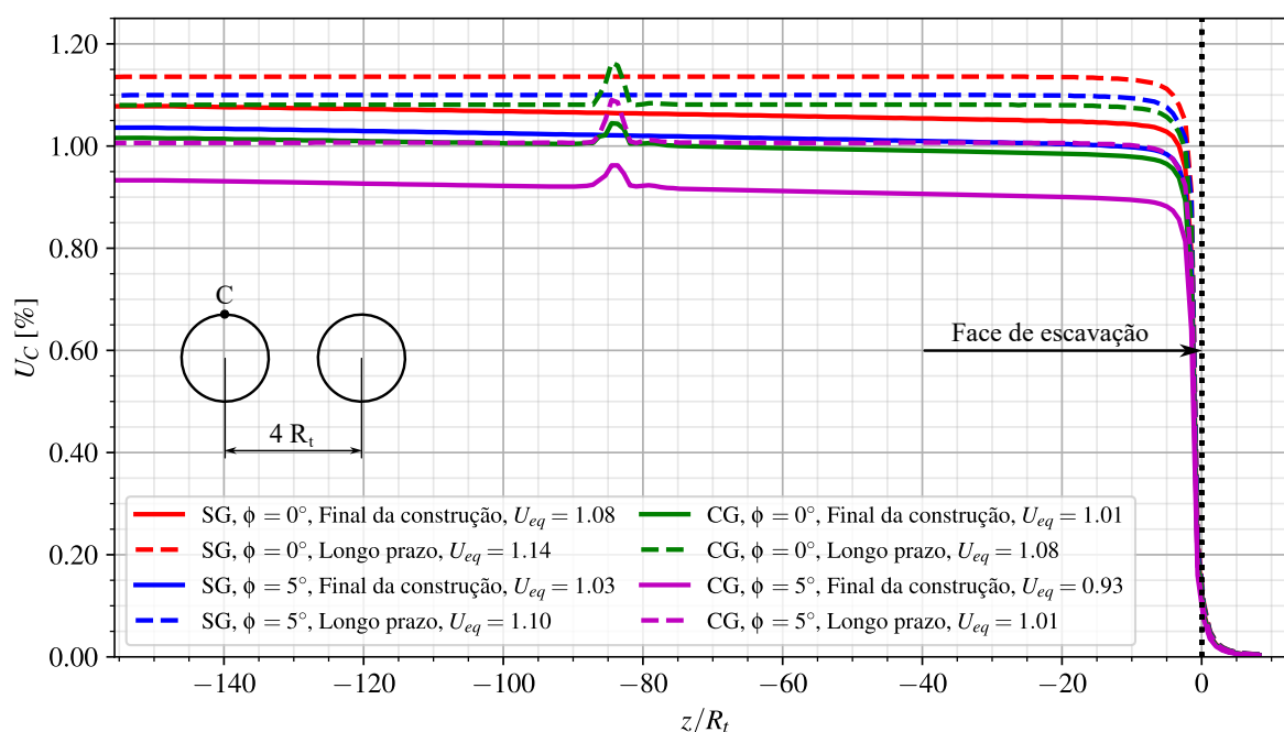
Figura 8.1 – Perfis de convergência - túneis gêmeos sem galeria (SG) e com galeria (CG) com revestimento elástico (CRE)
