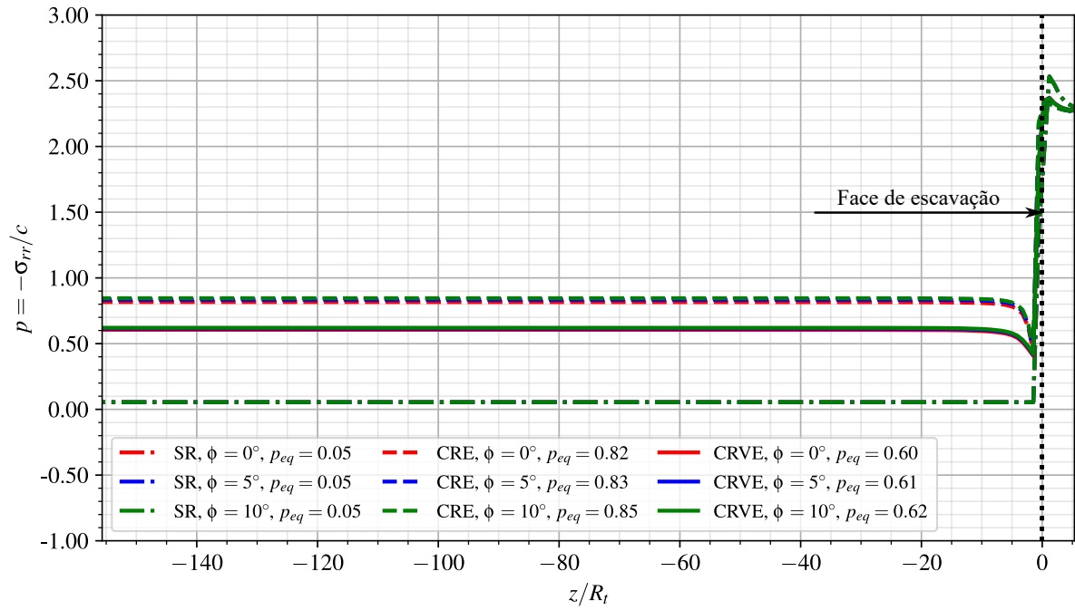
Figura 6.7 – Pressões no revestimento - túnel isolado sem revestimento (SR), com revestimento elástico (CRE) e viscoelástico (CRVE) no longo prazo
