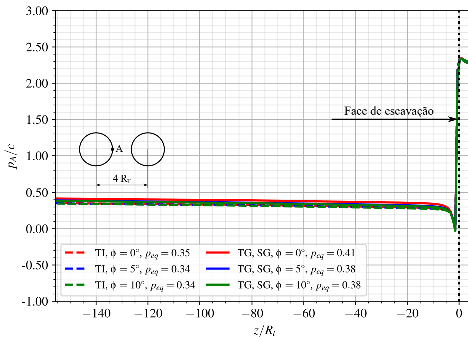
Figura A.21 – Perfis de convergência - Ponto A - túnel isolado (TI) e túneis gêmeos (TG) com revestimento viscoelástico (CRVE) no final da construção
