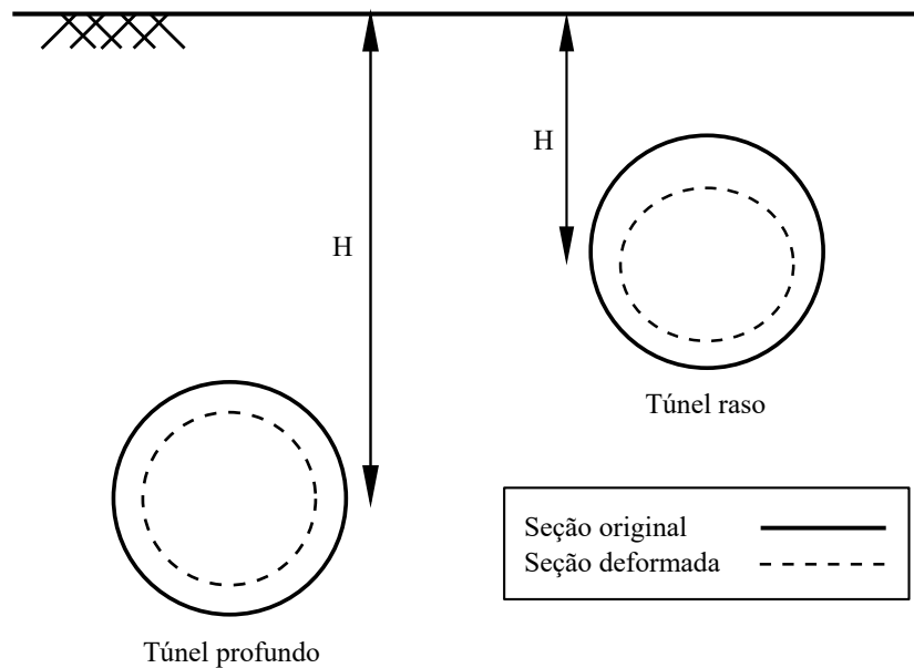
Figura 2.1 – Diferença no formato da seção transversal (adaptado de Jensen, Bernaud e Filho (2019))
