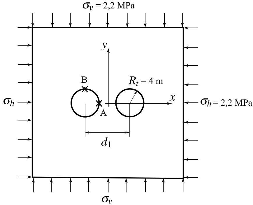
Figura 4.7 – Geometria e carregamento dos túneis gêmeos estudados por Guo, Liu e Zhu (2021))
