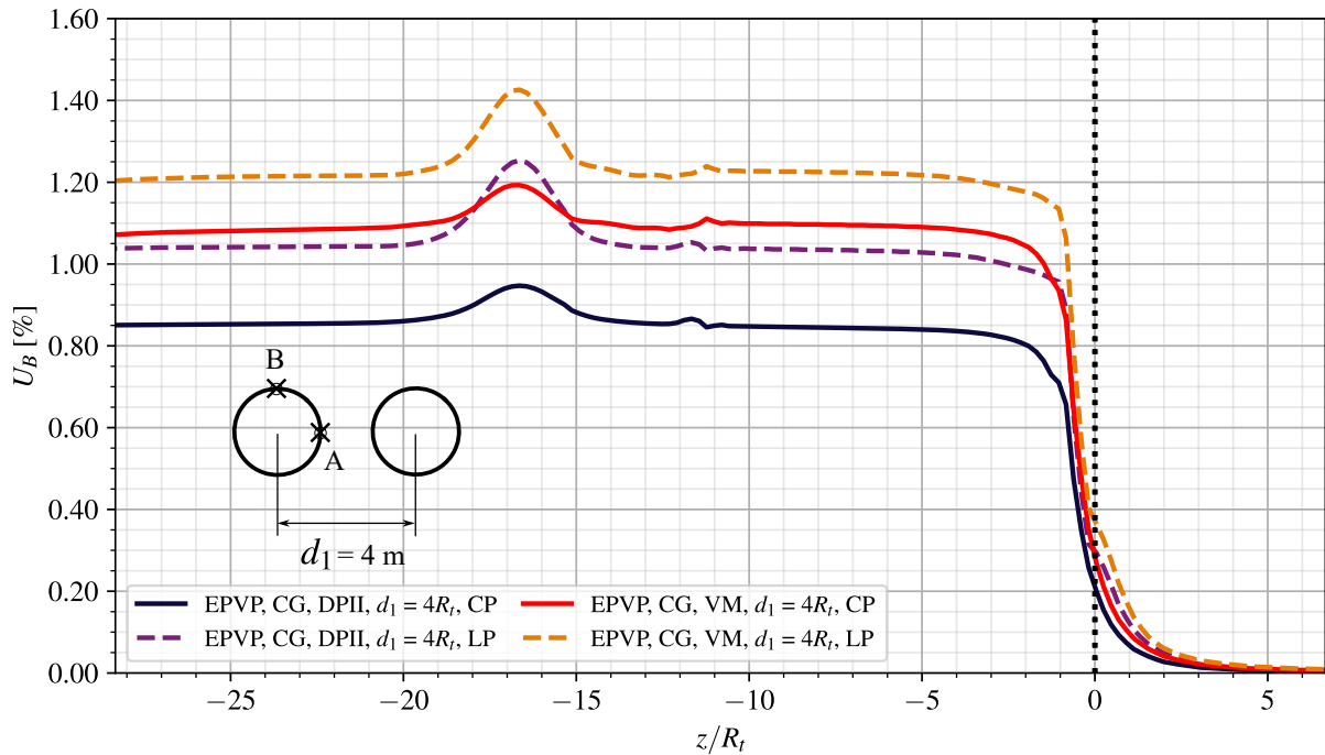
Figura 4.18 – Perfil de convergência dos túneis gêmeos para maciço elastoplástico e sem revestimento, considerando curto e longo prazo
