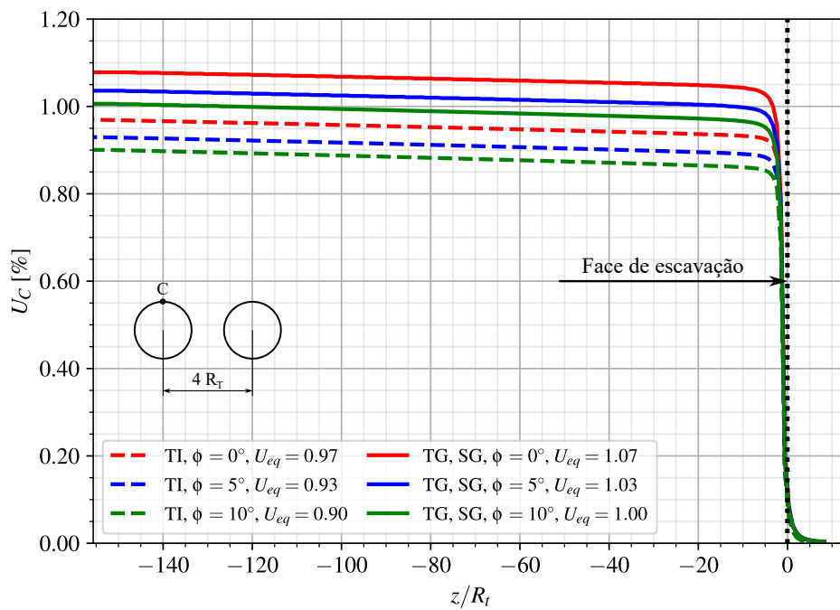
Figura 7.4 – Perfis de convergência - túnel isolado (TI) e túneis gêmeos (TG) sem galeria (SG), com revestimento elástico (CRE) no final da construção
