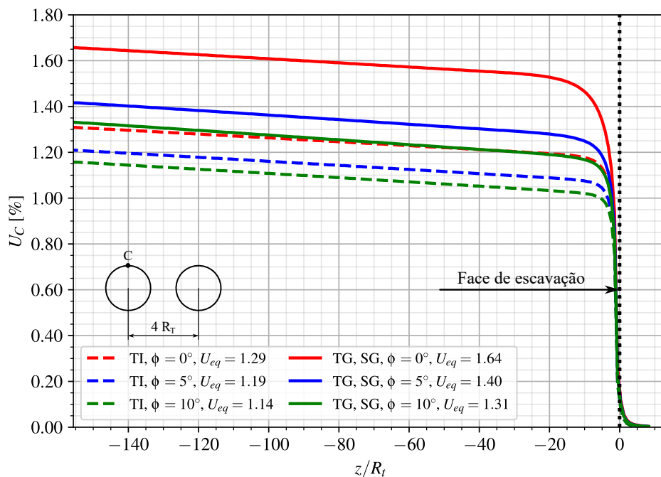
Figura 7.2 – Perfis de convergência - túnel isolado (TI) e túneis gêmeos (TG) sem galeria (SG), sem revestimento (SR) no final da construção
