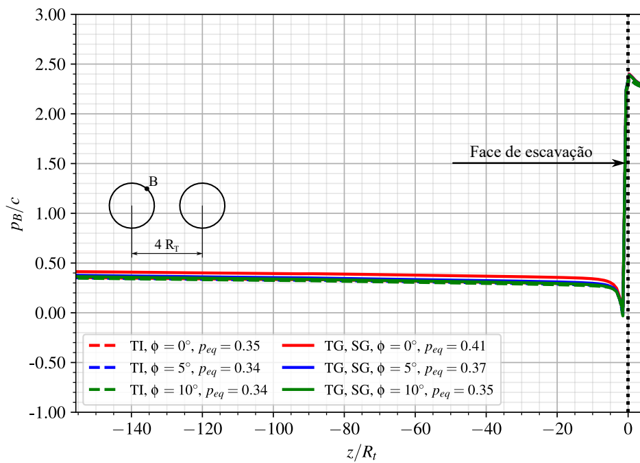
Figura A.23 – Perfis de convergência - Ponto B - túnel isolado (TI) e túneis gêmeos (TG) com revestimento viscoelástico (CRVE) no final da construção
