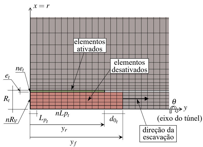
Figura 4.2 – Detalhe dos parâmetros que envolvem a escavação e colocação do revestimento
