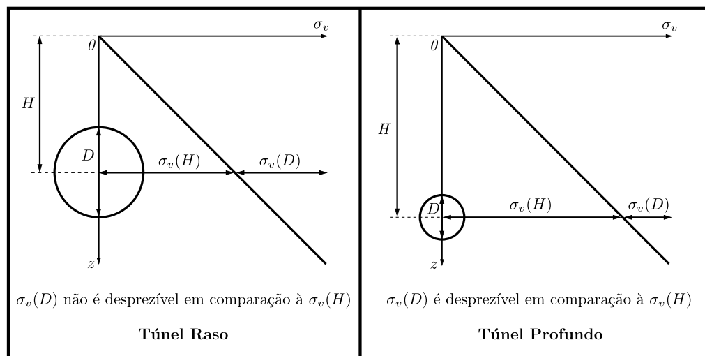
Figura 2.2 – Distinção entre túnel raso e profundo (fonte: adaptado de Benamar (fazer a citação))
