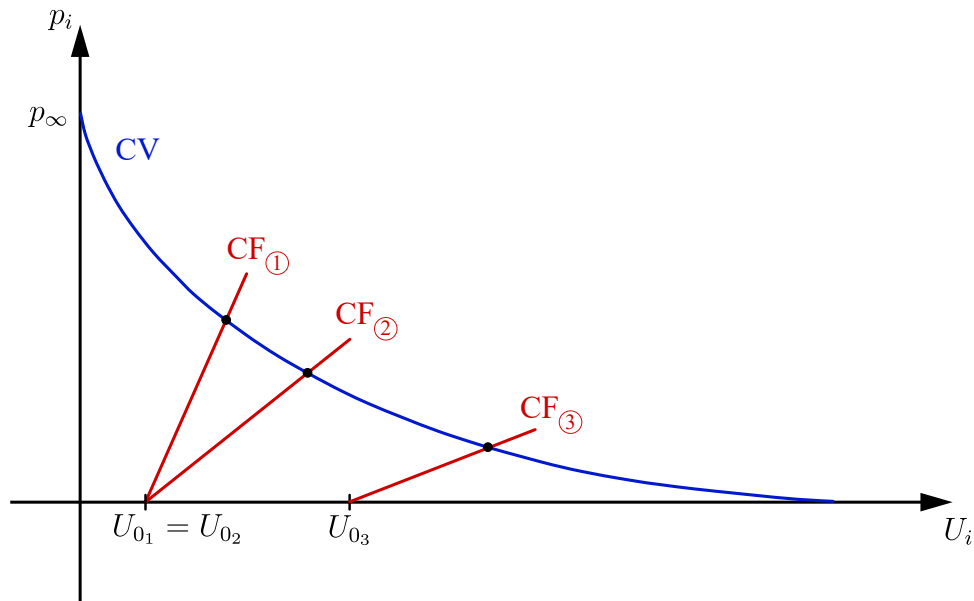
Figura 2.18 – Curvas características do maciço (CV) e do revestimento (CF)
