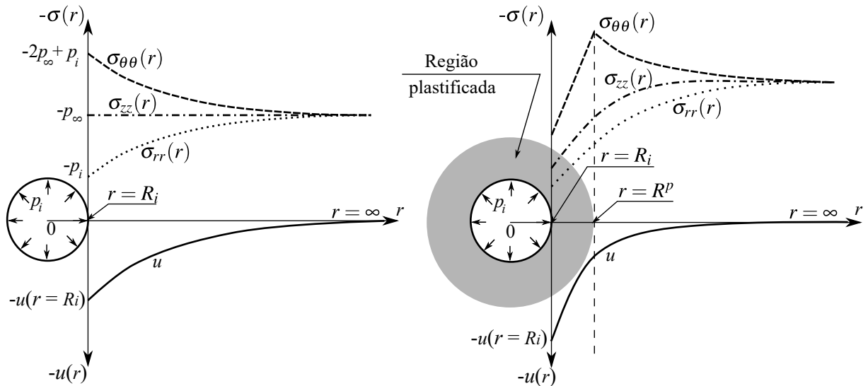
Figura 2.16 – Deslocamentos e tensões no entorno de um maciço submetido à pressão geostática-hidrostática p_\infty e pressão interna p_i no interior da seção do túnel. Elasticidade (esquerda) e elastoplasticidade (direita). (QUEVEDO, 2021)
