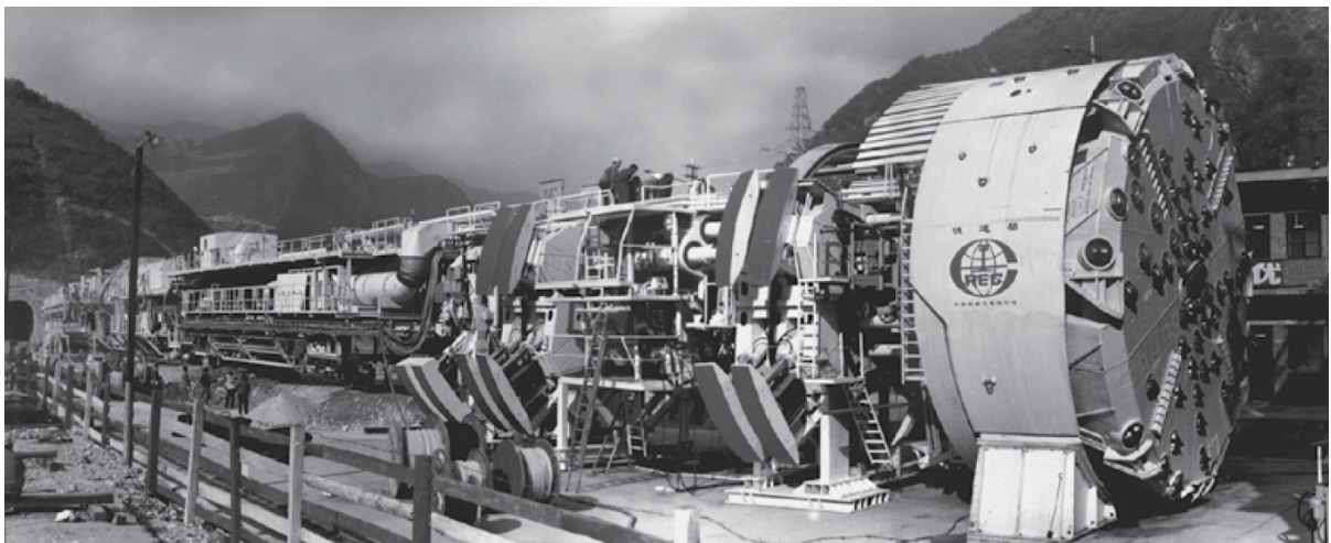
Figura 2.6 – Tuneladora com múltiplas garras (CHAPMAN; METJE; STÄRK, 2018)
