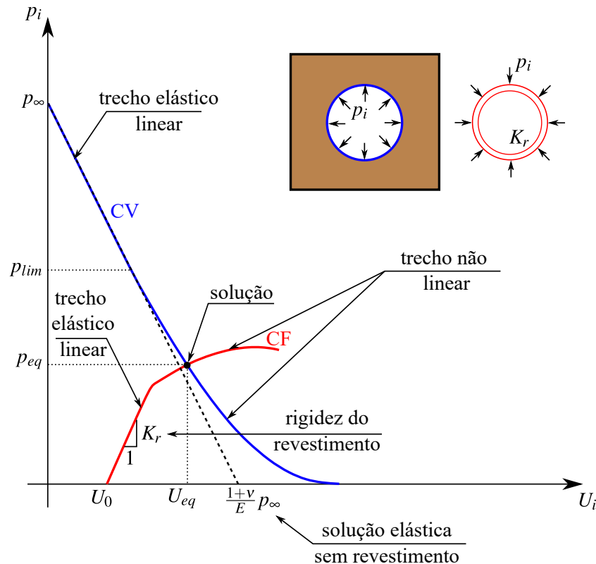
Figura 2.17 – Método convergência-confinamento (QUEVEDO, 2021)
