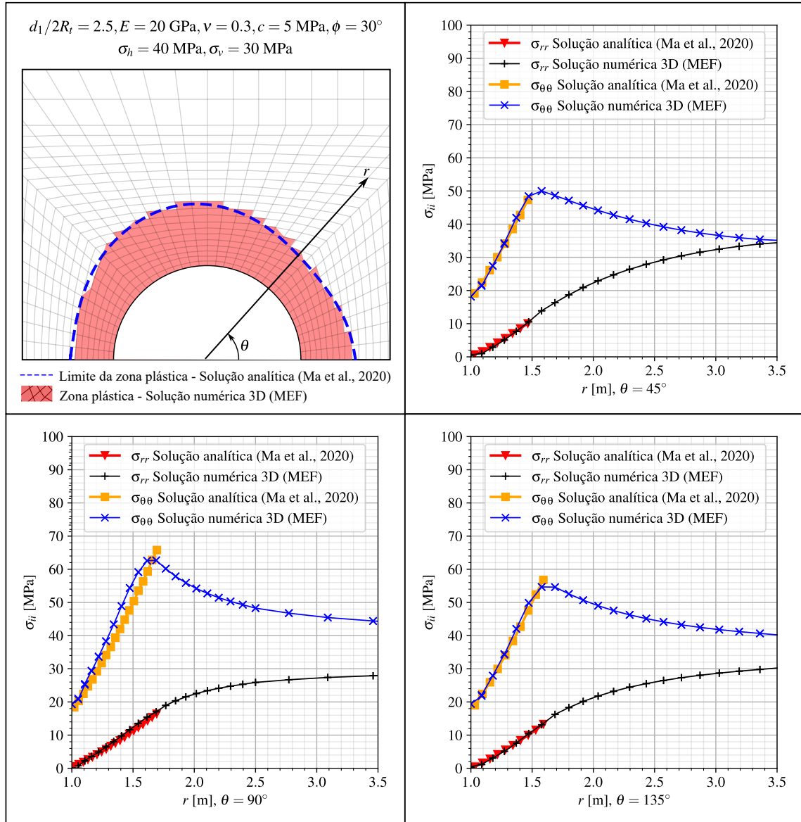
Figura 4.8 – Distribuição dos componentes de tensão radial e ortorradial ao longo de diferentes direções radiais: comparação entre simulações numérica e analítica - critério Drucker-Prager
