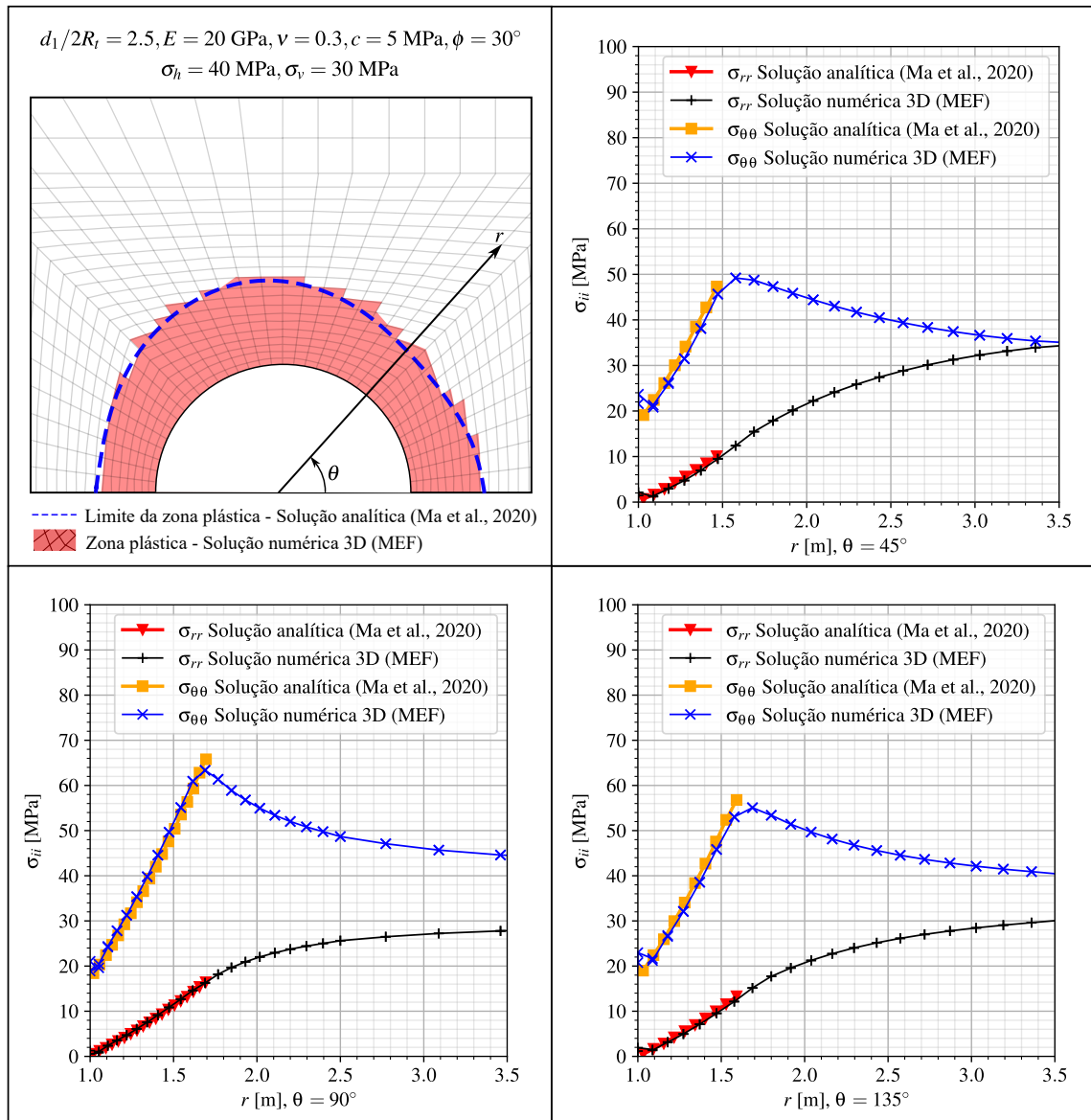
Figura 4.9 – Distribuição dos componentes de tensão radial e ortorradial ao longo de diferentes direções radiais: comparação entre simulações numérica e analítica - critério Mohr-Coulomb
