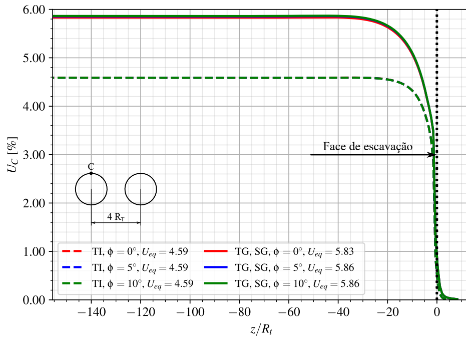
Figura 7.3 – Perfis de convergência - túnel isolado (TI) e túneis gêmeos (TG) sem galeria (SG) e sem revestimento (SR) no longo prazo
