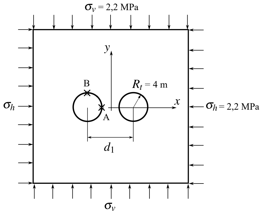
Figura 4.1 – Geometria e carregamento dos túneis gêmeos estudados por Guo et al. (2021))
