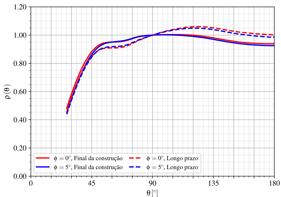
Figura 8.8 – Deformada da seção - túneis gêmeos com galeria com revestimento viscoelástico (CRVE) na seção 2
