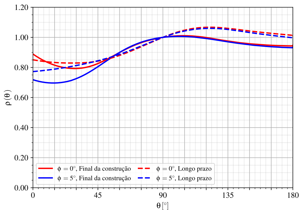
Figura 8.9 – Deformada da seção - túneis gêmeos com galeria com revestimento viscoelástico (CRVE) na seção 3
