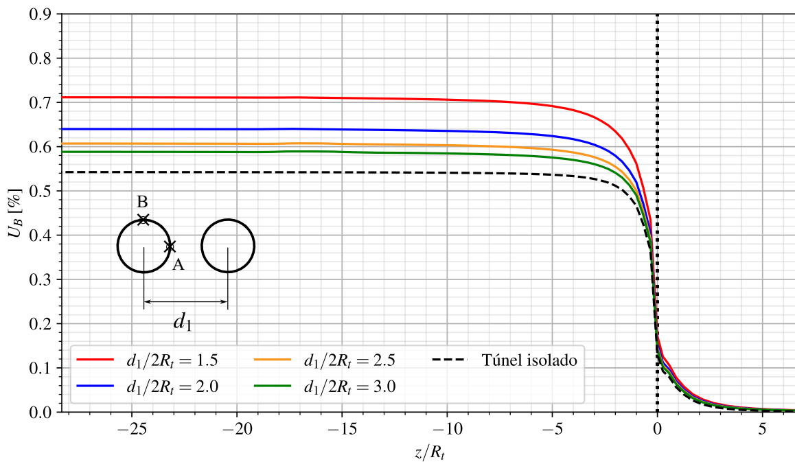
Figura 4.2 – Perfis de convergência no teto do túnel (ponto B)
