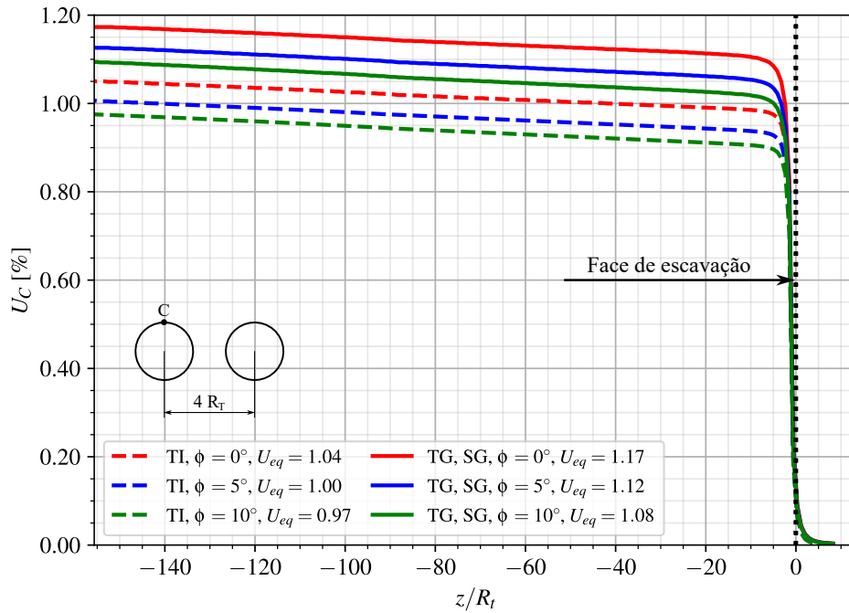
Figura 7.6 – Perfis de convergência - túnel isolado (TI) e túneis gêmeos (TG) sem galeria (SG), com revestimento viscoelástico (CRVE) no final da construção
