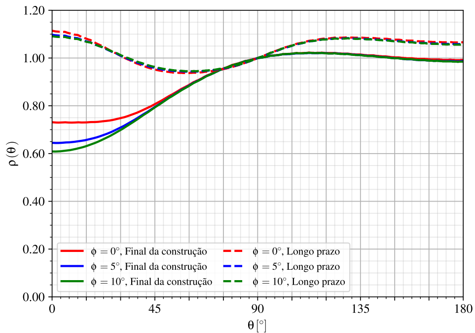
Figura 7.13 – Deformada da seção - túneis gêmeos sem galeria com revestimento viscoelástico (CRVE)
