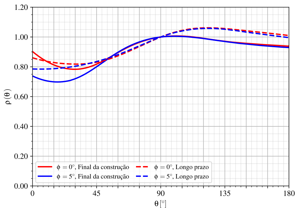
Figura 8.7 – Deformada da seção - túneis gêmeos com galeria com revestimento viscoelástico (CRVE) na seção 1
