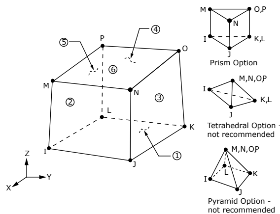
Figura 5.3 – Elemento SOLID185 (ANSYS Inc, 2024)
