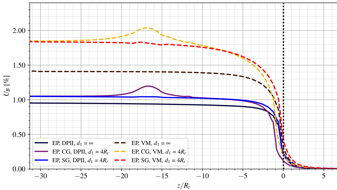
Figura 4.14 – Perfil de convergência dos túneis gêmeos para maciço elastoplástico e sem revestimento
