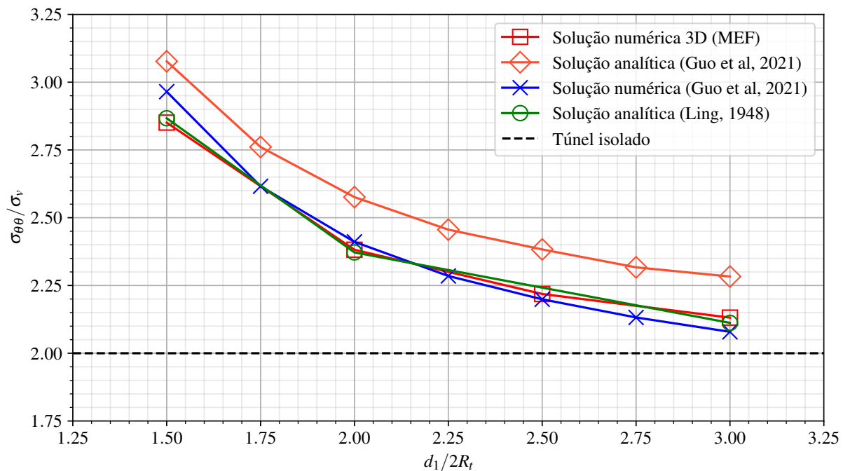
Figura 4.10 – Fator de concentração de tensão tangencial no ponto A versus distância dos túneis gêmeos d_1/2R_t
