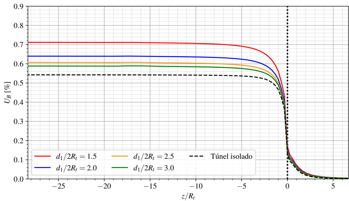
Figura 4.8 – Perfis de convergência no ponto B
