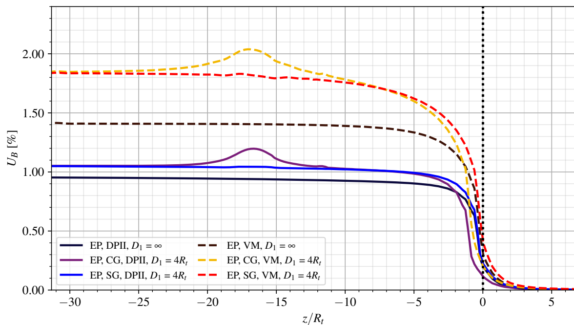
Figura 4.14 – Perfis de convergência dos túneis gêmeos para maciço elastoplástico e sem revestimento
