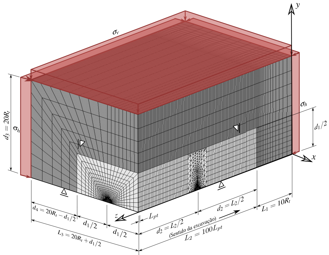
Figura 4.3 – Malha, dimensões e condições de contorno do domínio dos túneis gemêos tridimensionais. (adaptado de Colombo (2023))
