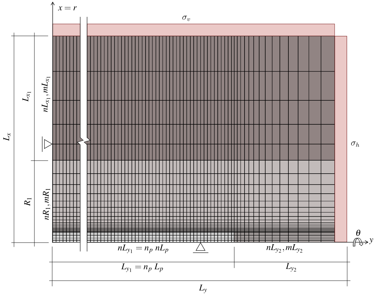
Figura 4.1 – Domínio, condições de contorno e parâmetros geométricos do modelo axissimétrico
