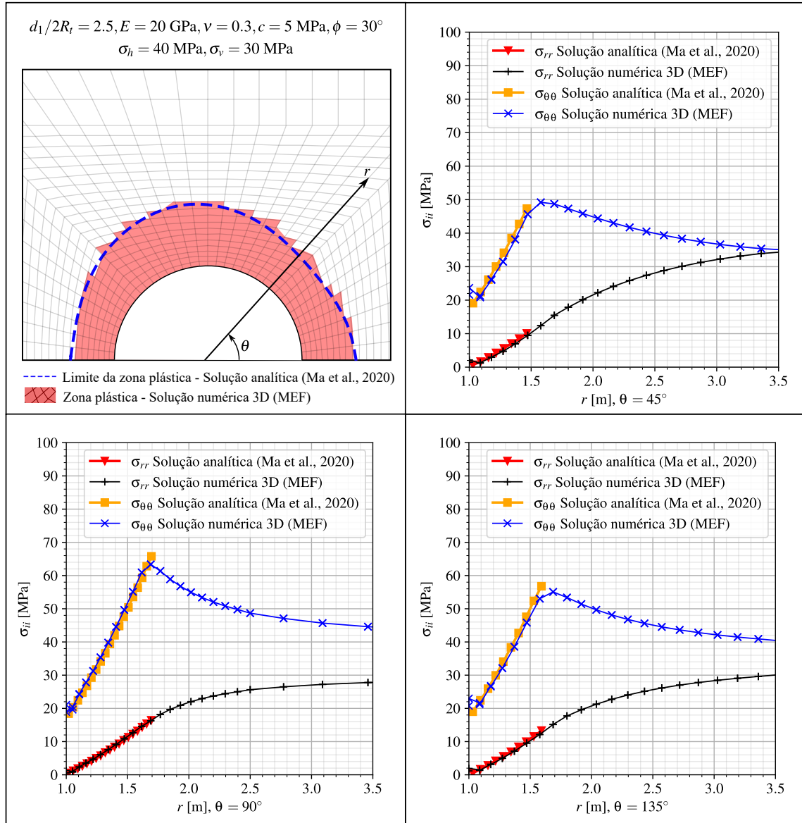
Figura 5.9 – Distribuição dos componentes de tensão radial e ortorradial ao longo de diferentes direções radiais: comparação entre simulações numérica e analítica - critério Mohr-Coulomb
