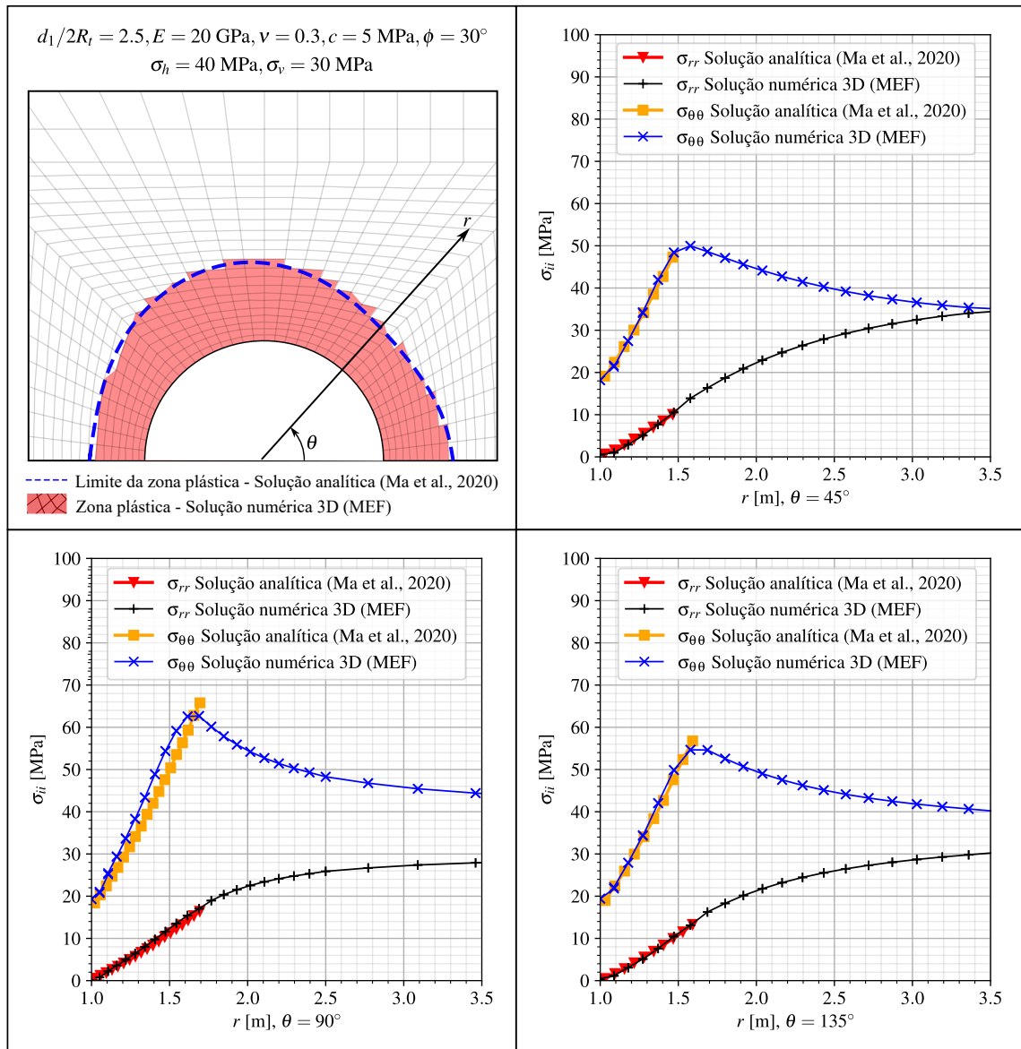
Figura 5.8 – Distribuição dos componentes de tensão radial e ortorradial ao longo de diferentes direções radiais: comparação entre simulações numérica e analítica - critério Drucker-Prager
