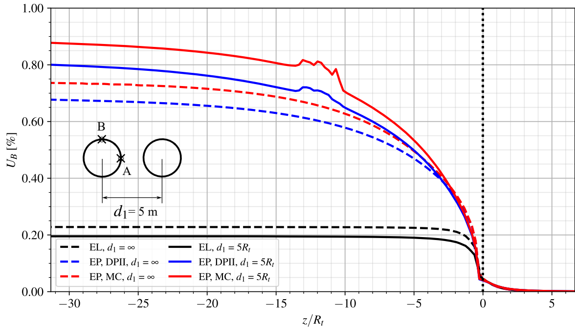
Figura 5.6 – Perfis de convergência no teto do túnel (ponto B)
