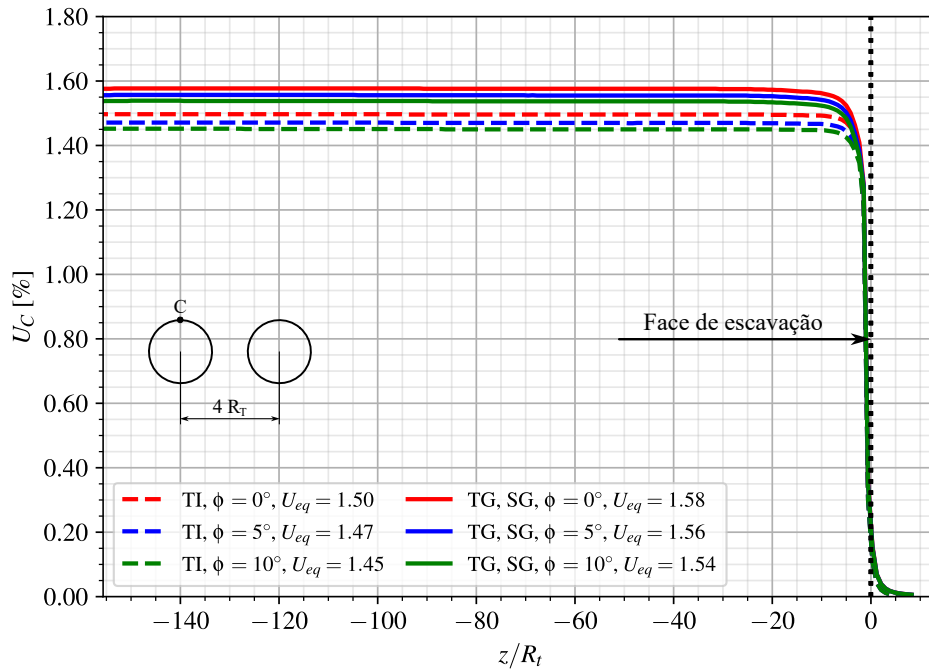
Figura 7.7 – Perfis de convergência - túnel isolado (TI) e túneis gêmeos (TG) sem galeria (SG), com revestimento viscoelástico (CRVE) no longo prazo
