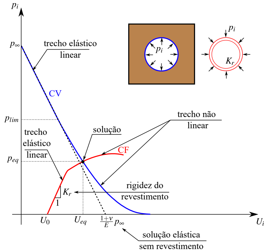
Figura 2.12 – Método convergência-confinamento (fonte: Quevedo (2021) (fazer a citação))
