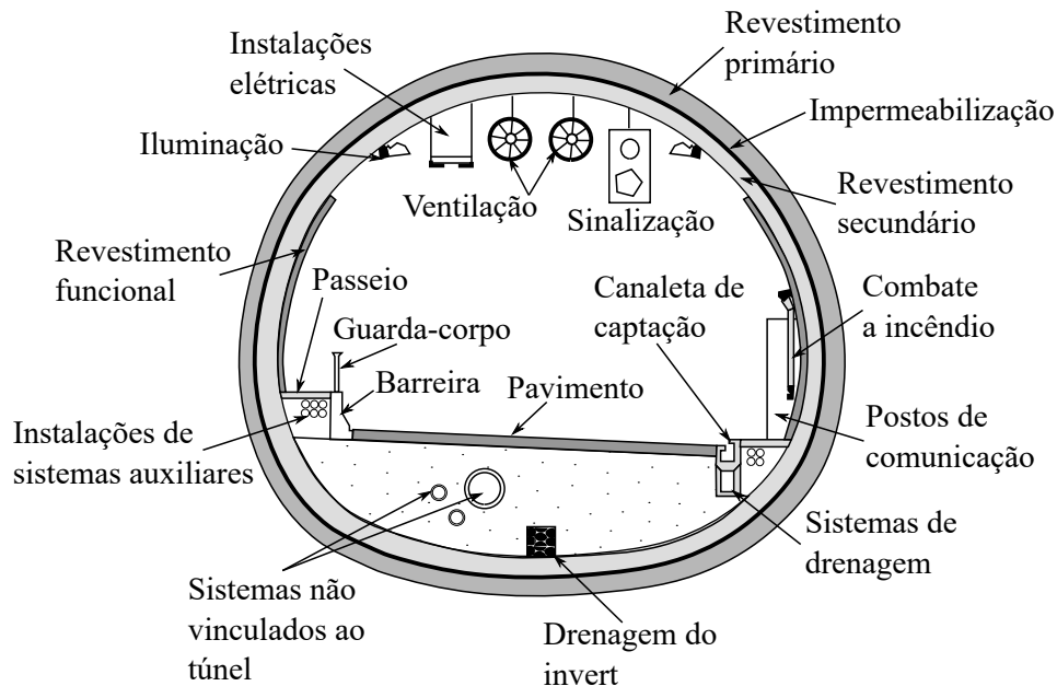
Figura 2.5 – Elementos de revestimento de túnel rodoviário (fonte: Quevedo (2021) ou adaptado de DAER? (fazer a citação))
