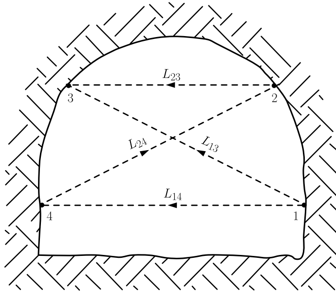
Figura 2.11 – Seção de medição de convergência em quatro direções (fonte: adaptado de Panet (1985) (fazer a citação))
