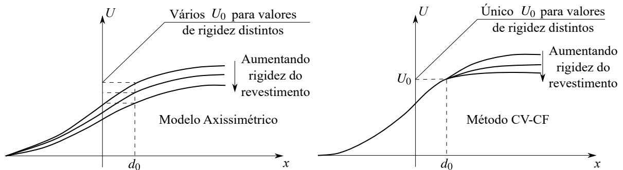
Figura 2.20 – Influência da rigidez do revestimento no perfil de convergências e no parâmetro U_0 (adaptado de Bernaud e Rousset (1992))
