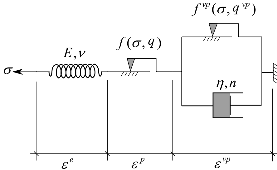
Figura 3.1 – Representação reológica do modelo elastoplástico viscoplástico (adaptado de Rousset (1988))
