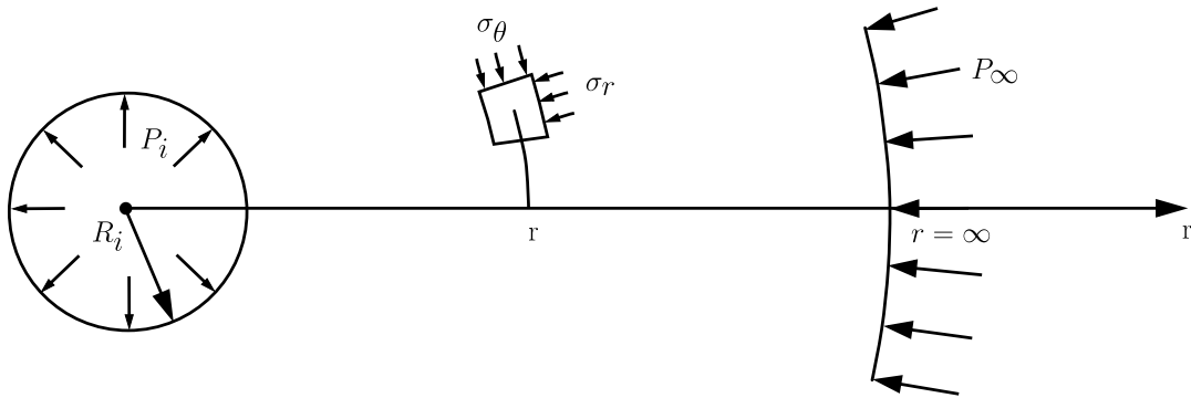
Figura 2.15 – Geometria e carregamento do túnel (adaptado de Bernaud (1991))
