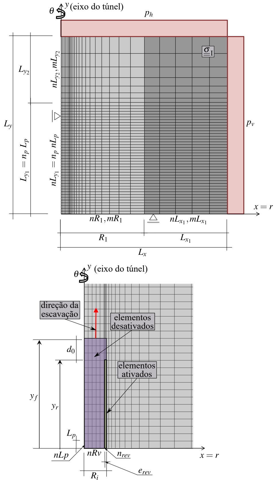
Figura 4.1 – Domínio, condições de contorno e parâmetros geométricos do modelo axissimétrico (QUEVEDO, 2021)
