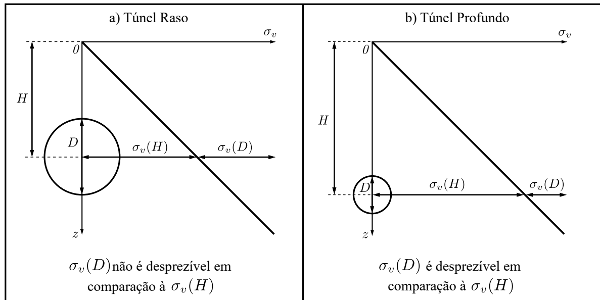
Figura 2.14 – Variação da tensão vertical (adaptado de Benamar (1996))
