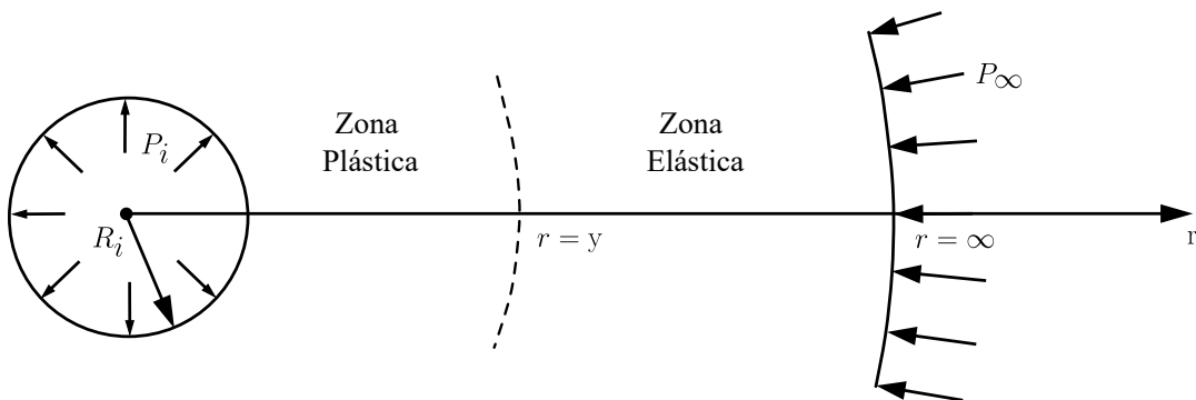
Figura 2.16 – Delimitação das regiões plástica e elástica (adaptado de Bernaud (1991))
