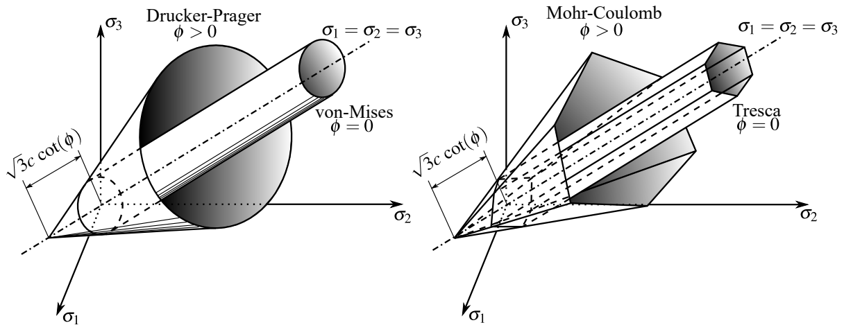
Figura 3.2 – Funções de escoamento de Drucker-Prager e Mohr-Coulomb (adaptado de Zienkiewicz e Corneau (1974))
