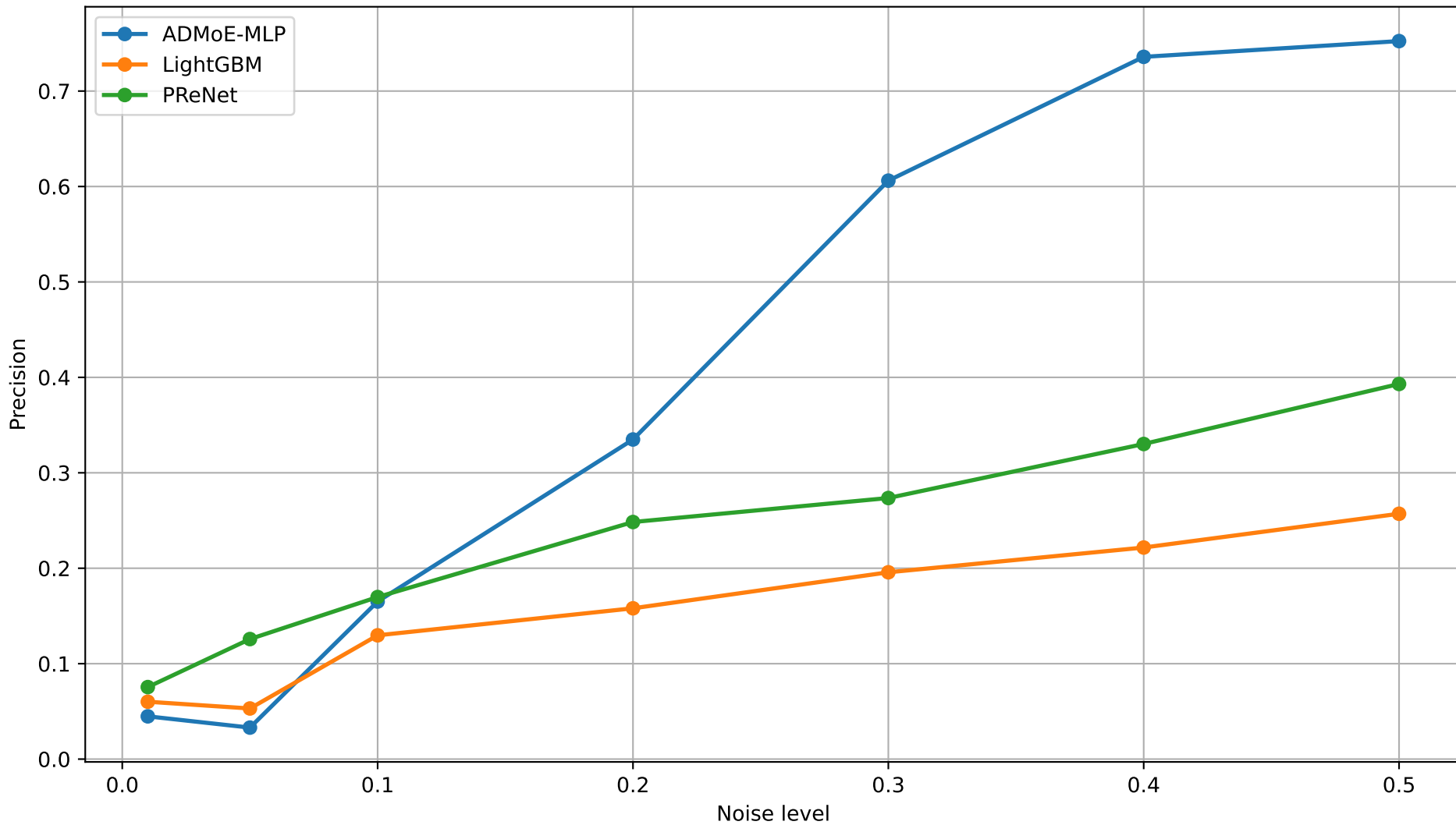
Precision vs Noise Level - imdb
