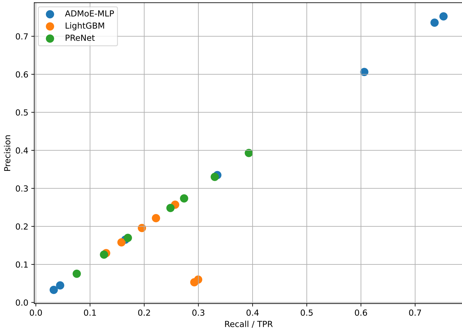
Precision vs Recall - imdb
