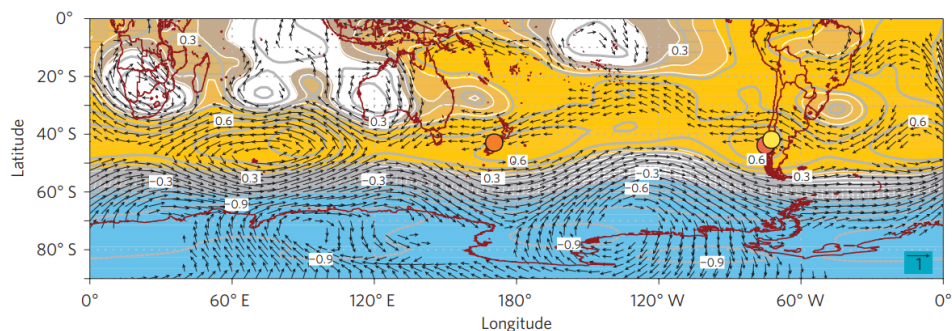
Figura 4: Regresión entre el índice de la AAO y la presión atmosférica (líneas) y vientos de los oestes (vectores). Fuente: Villalba et al. ([47])
