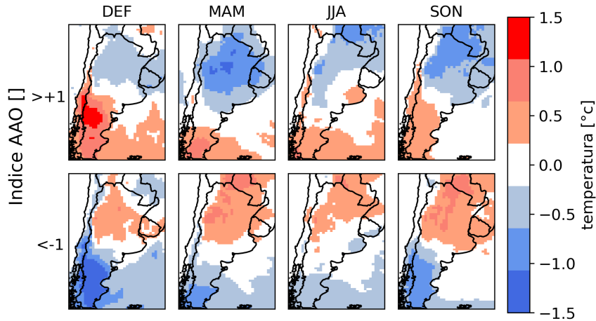
Figura 14: Mapas de anomalías de temperatura del aire por estación del año y por fase de la AAO
