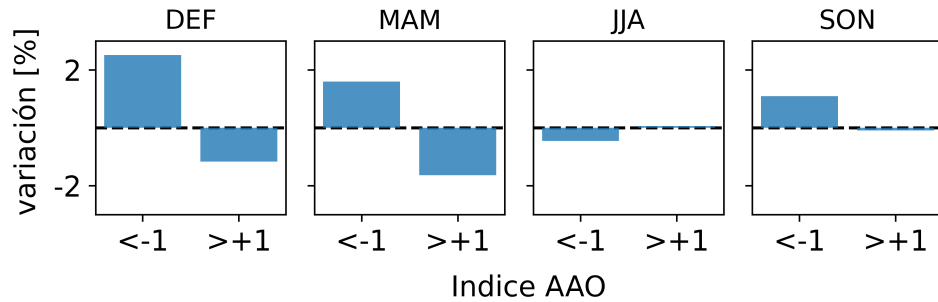
Figura 13: Anomalías percentuales de demanda eléctrica por estación del año y por fase de la AAO
