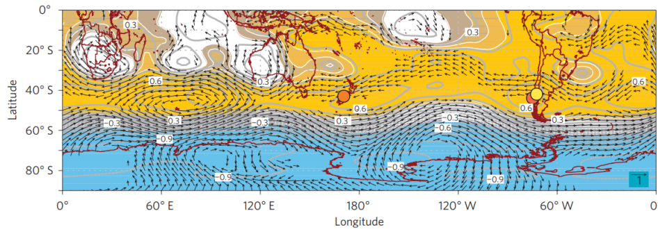
Figura 4: Regresión entre el índice de la AAO y la presión atmosférica (líneas) y vientos de los oestes (vectores). Fuente: Villalba et al. ([?])
