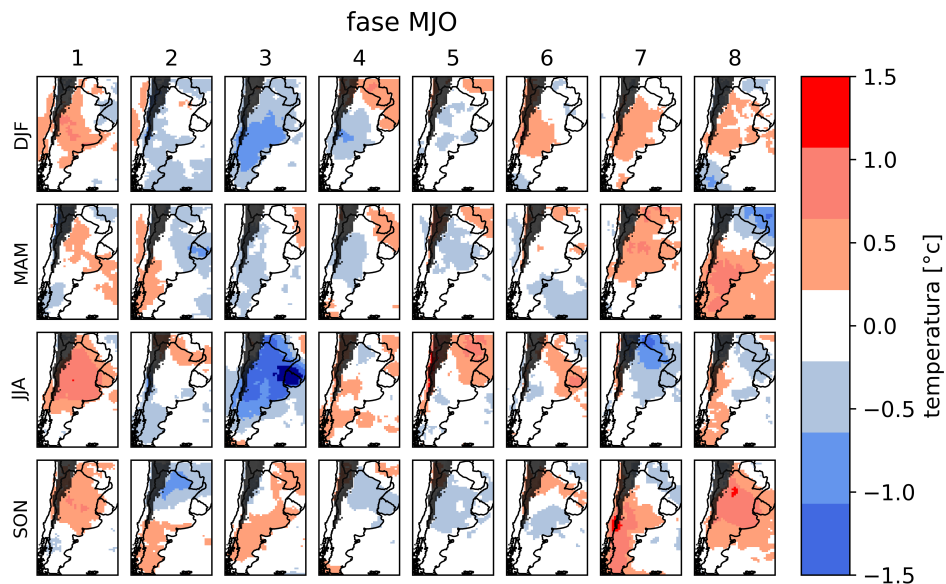
Figura 12: Mapas de anomalías de temperatura del aire por estación del año y por fase de la MJO
