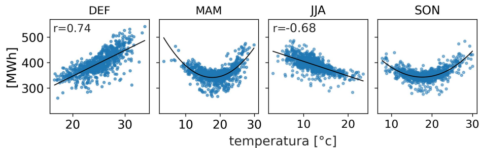
Figura 10: Diagramas de dispersión entre demanda eléctrica y temperatura del aire
