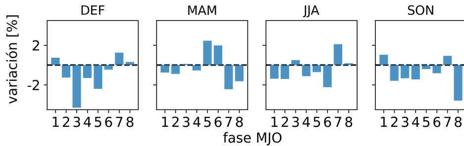
Figura 11: Anomalías porcentuales de demanda eléctrica por estación del año y por fase de la MJO
