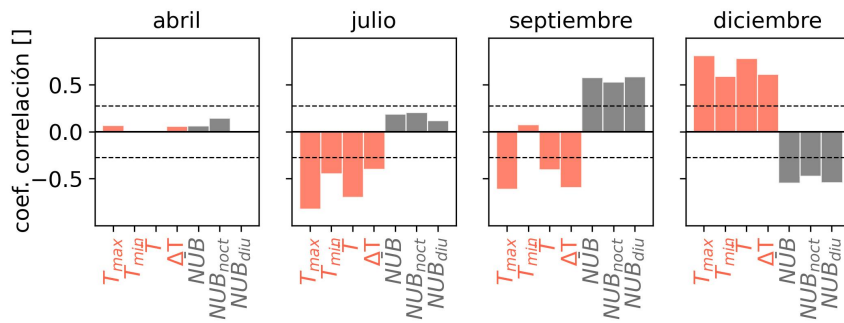
Figura 9: Coeficientes de correlación entre empuntamiento diario de la demanda eléctrica y parámetros meteorológicos
