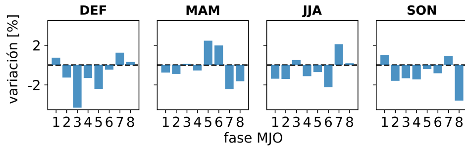
Figura 7: Anomalías porcentuales de demanda eléctrica por estación del año y por fase de la MJO
