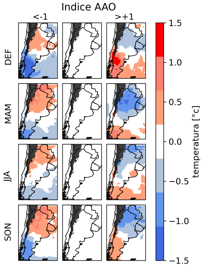
Figura 10: Mapas de anomalías de temperatura del aire por estación del año y por fase de la AAO
