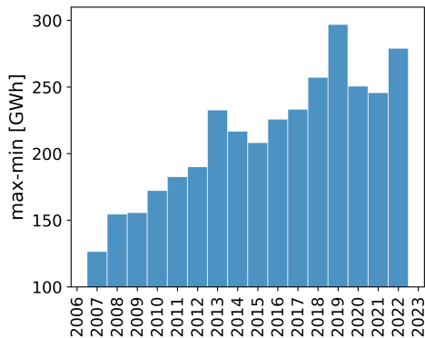
Figura 8: Diferencia anual entre máximo y mínimo absolutos de demanda diaria
