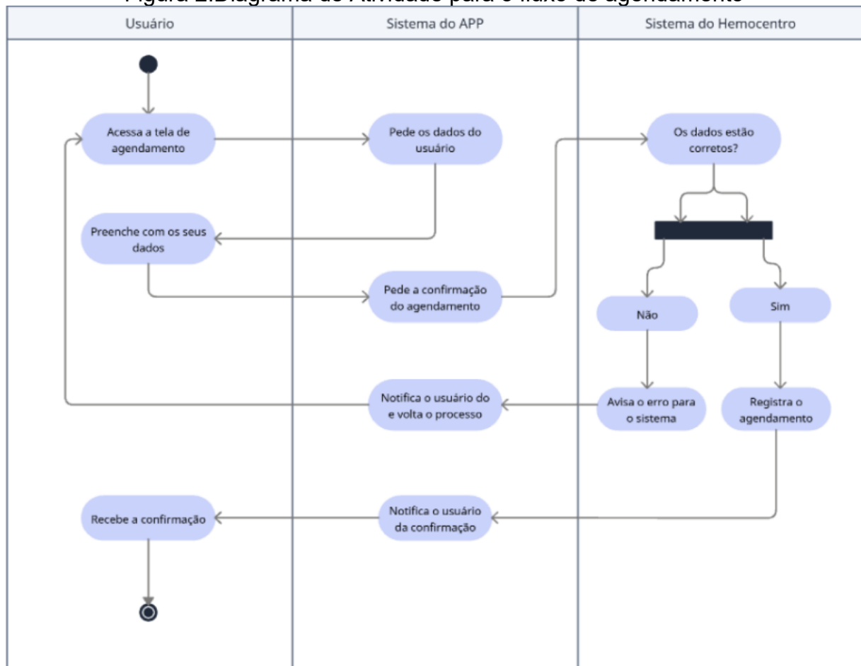
Figura 2:Diagrama de Atividade para o fluxo de agendamento
