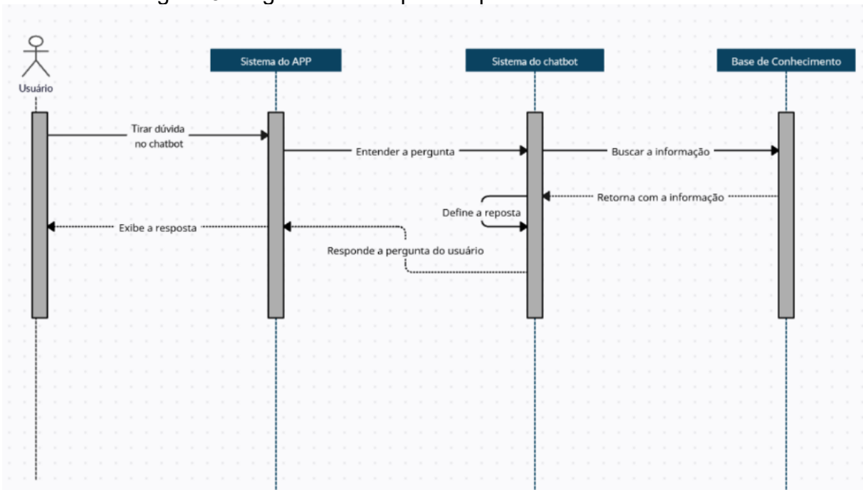
Figura 3: Diagrama de Sequência para consulta no chatbot
