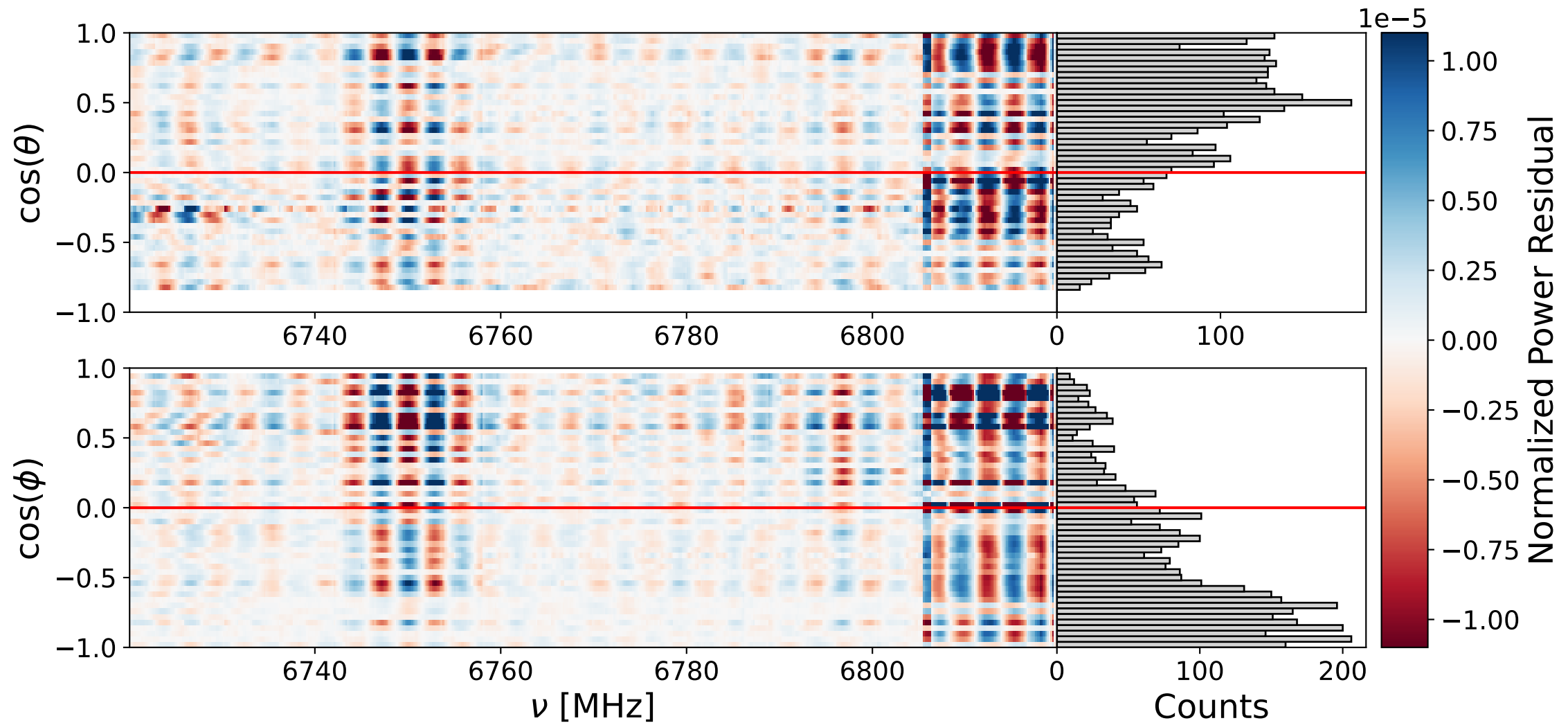
Bank 2 ann: 6720-6820 MHz
