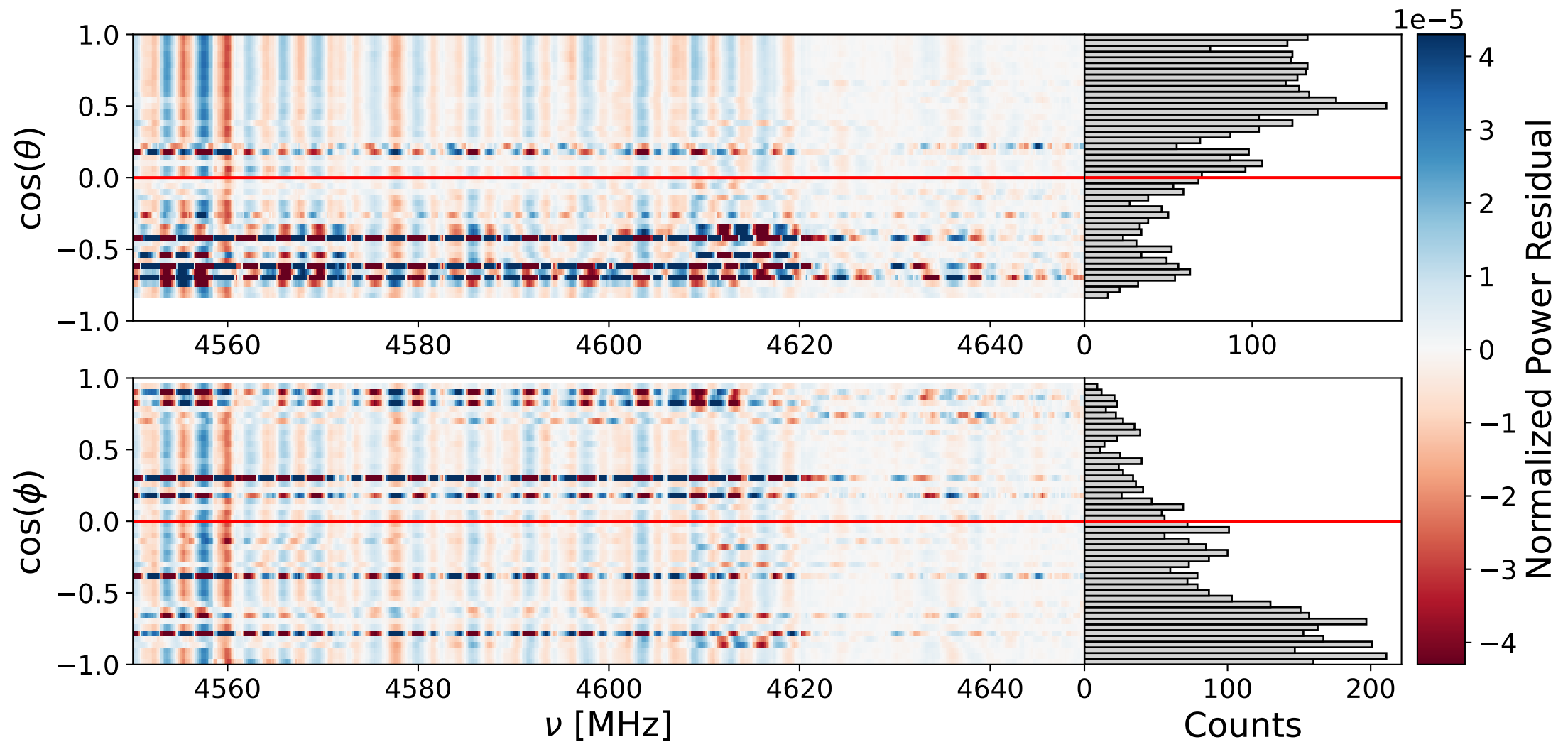
Bank 0 ann: 4550-4650 MHz
