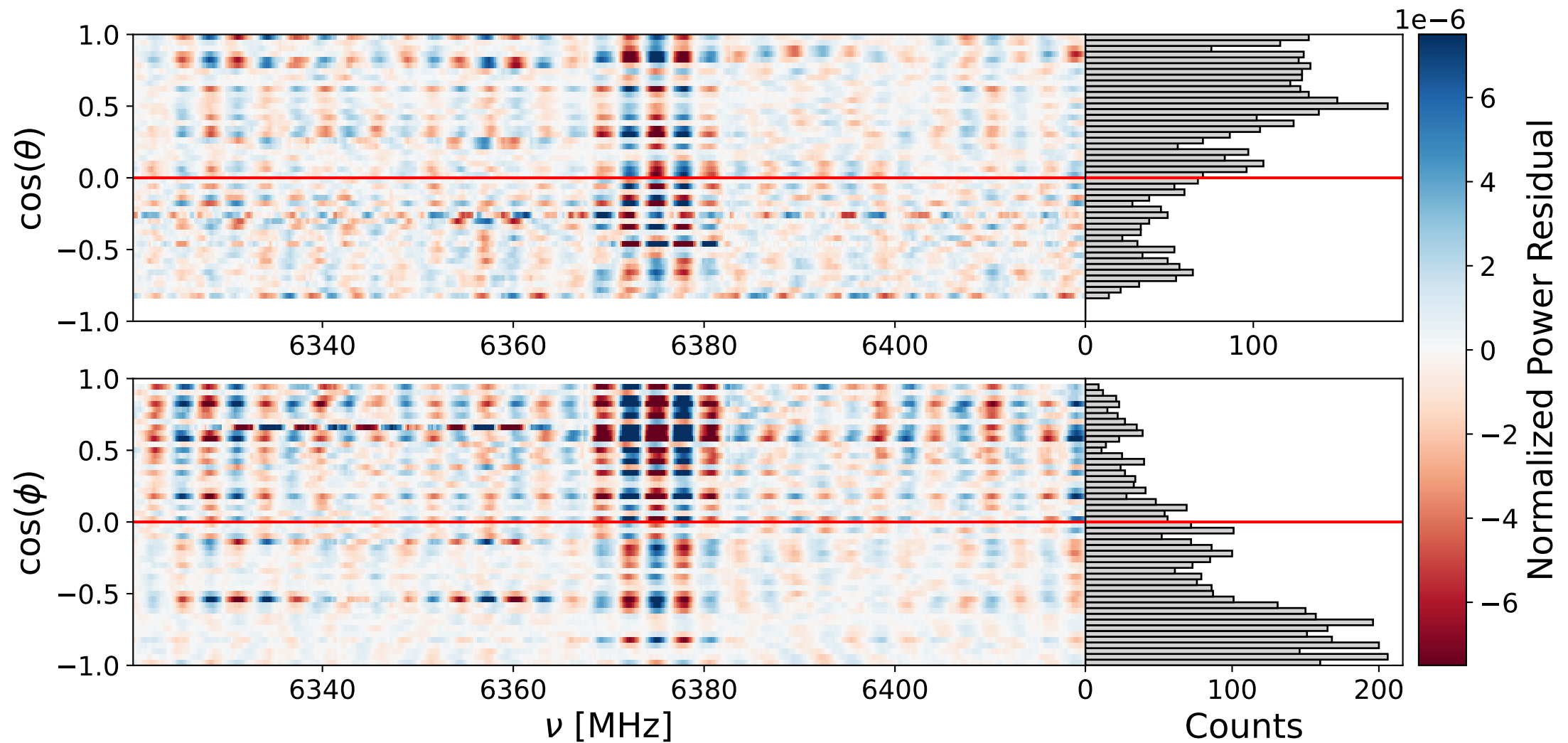
Bank 2 ann: 6320-6420 MHz
