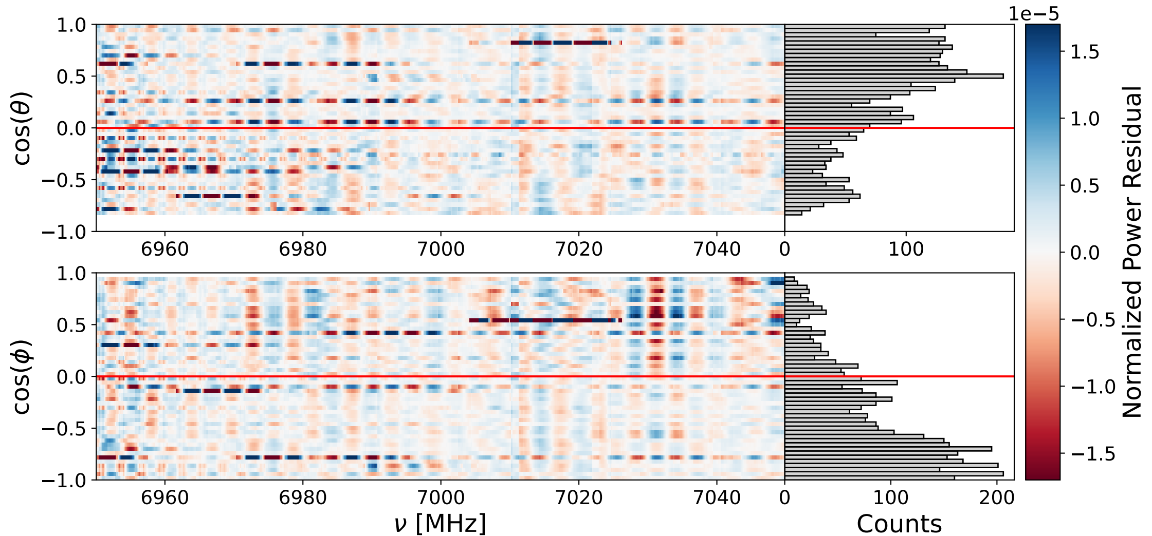
Bank 3 ann: 6950-7050 MHz
