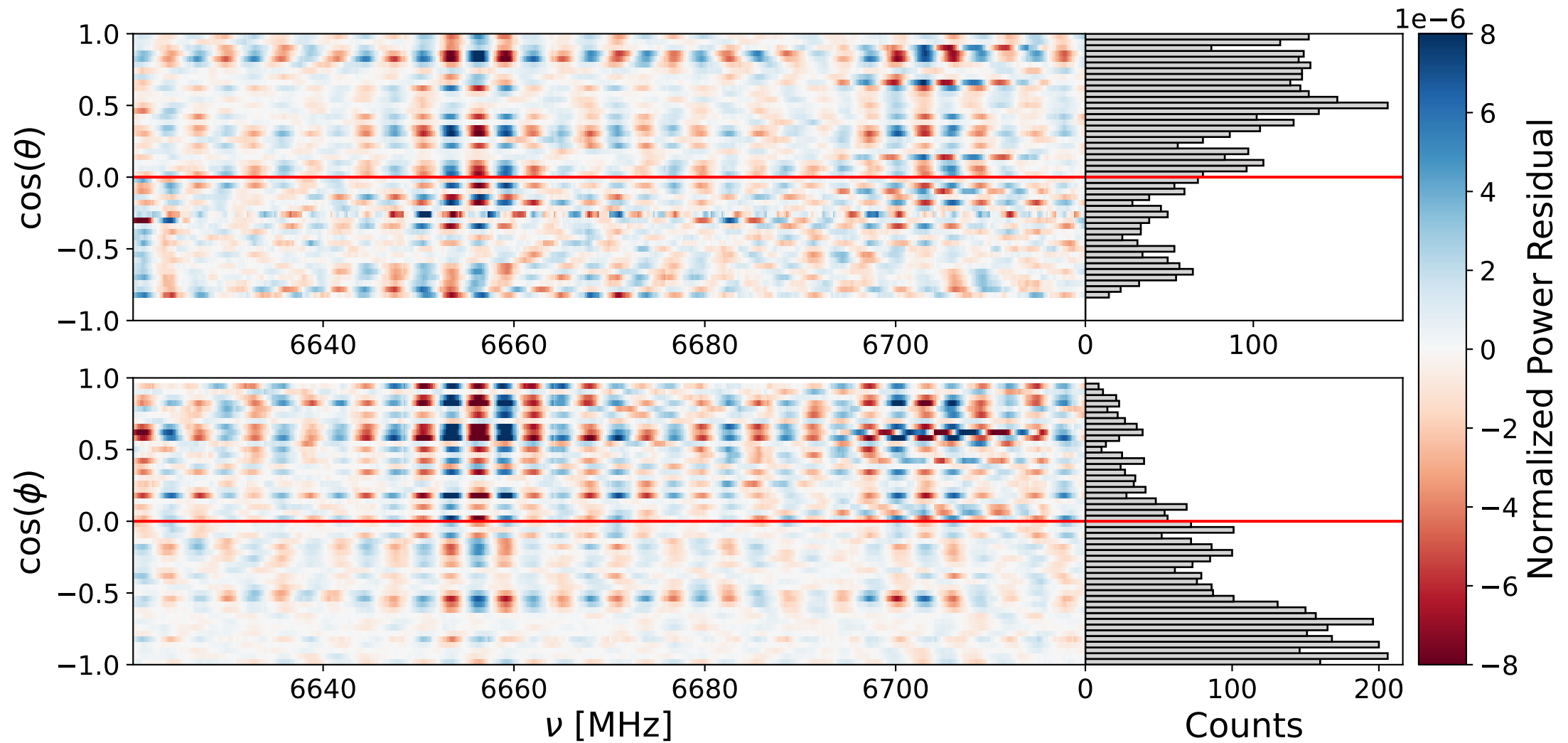
Bank 2 ann: 6620-6720 MHz
