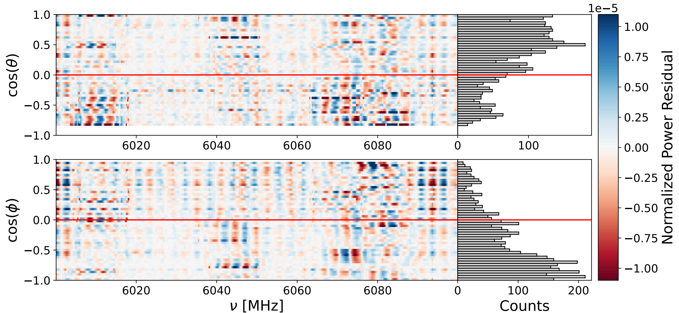
Bank 1 ann: 6000-6100 MHz
