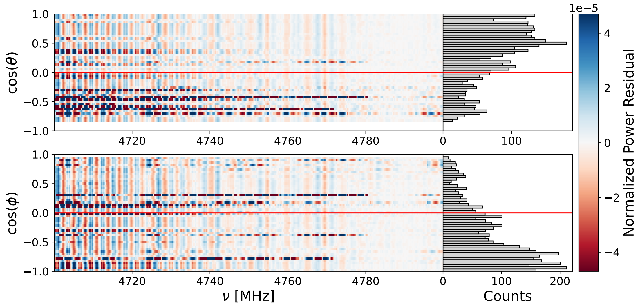
Bank 1 ann: 4700-4800 MHz
