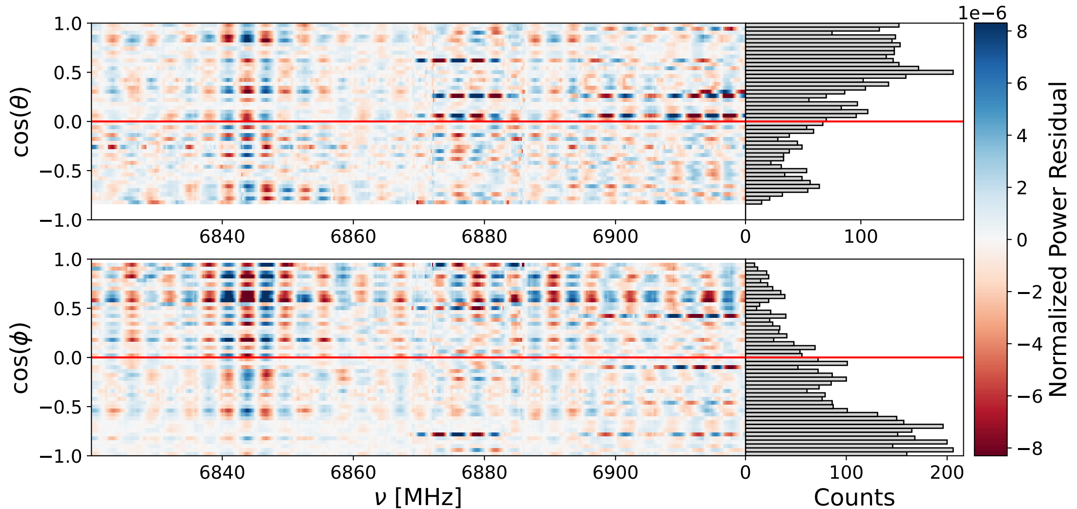
Bank 2 ann: 6820-6920 MHz
