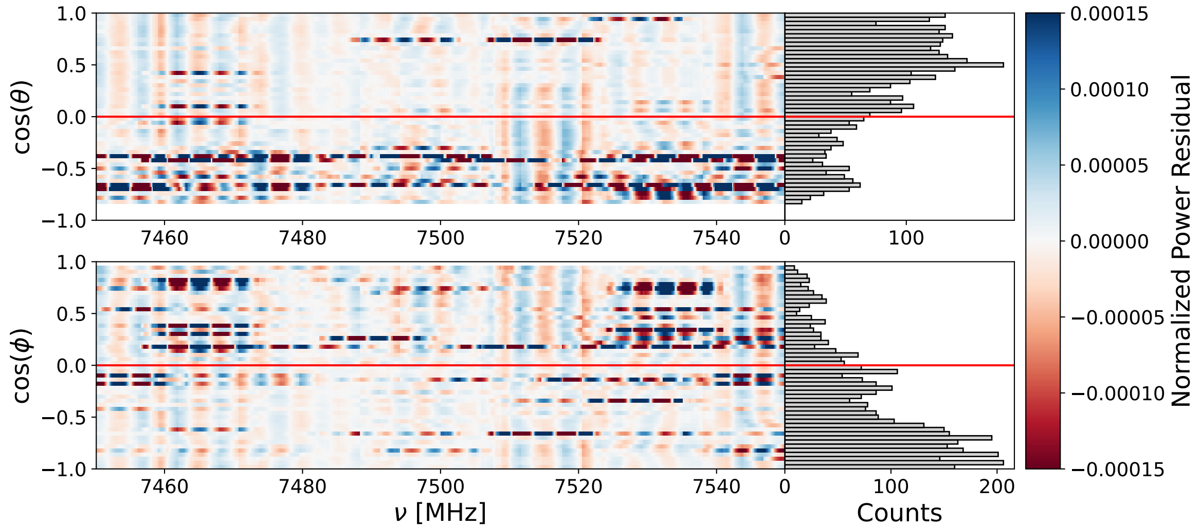
Bank 3 ann: 7450-7550 MHz
