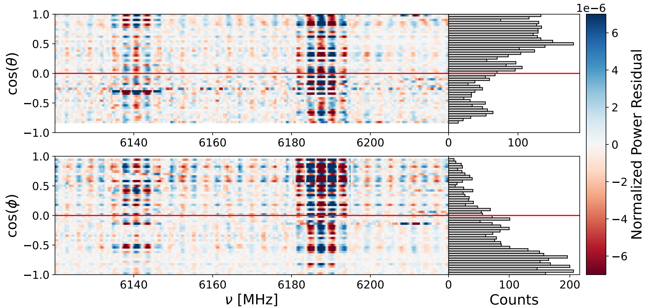
Bank 2 ann: 6120-6220 MHz
