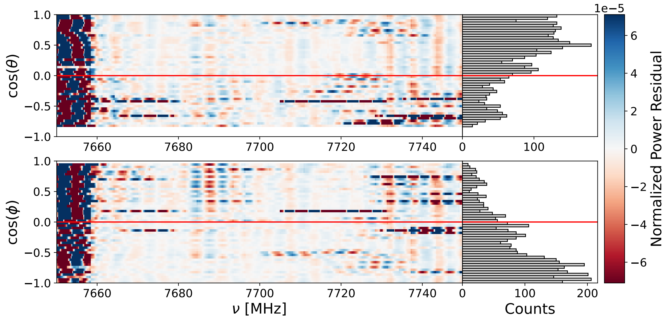
Bank 3 ann: 7650-7750 MHz
