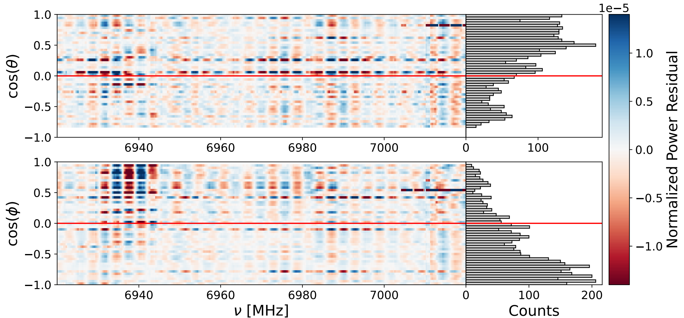
Bank 2 ann: 6920-7020 MHz
