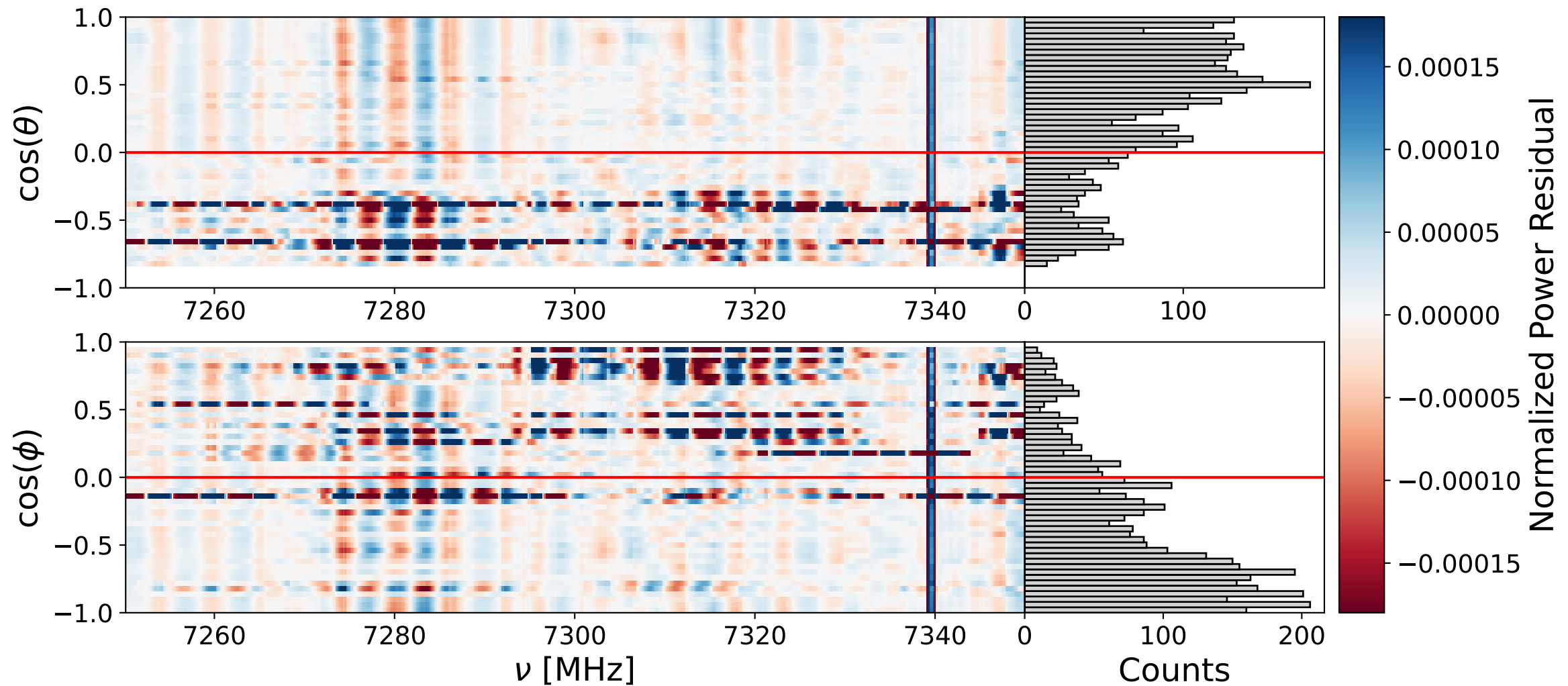
Bank 3 ann: 7250-7350 MHz
