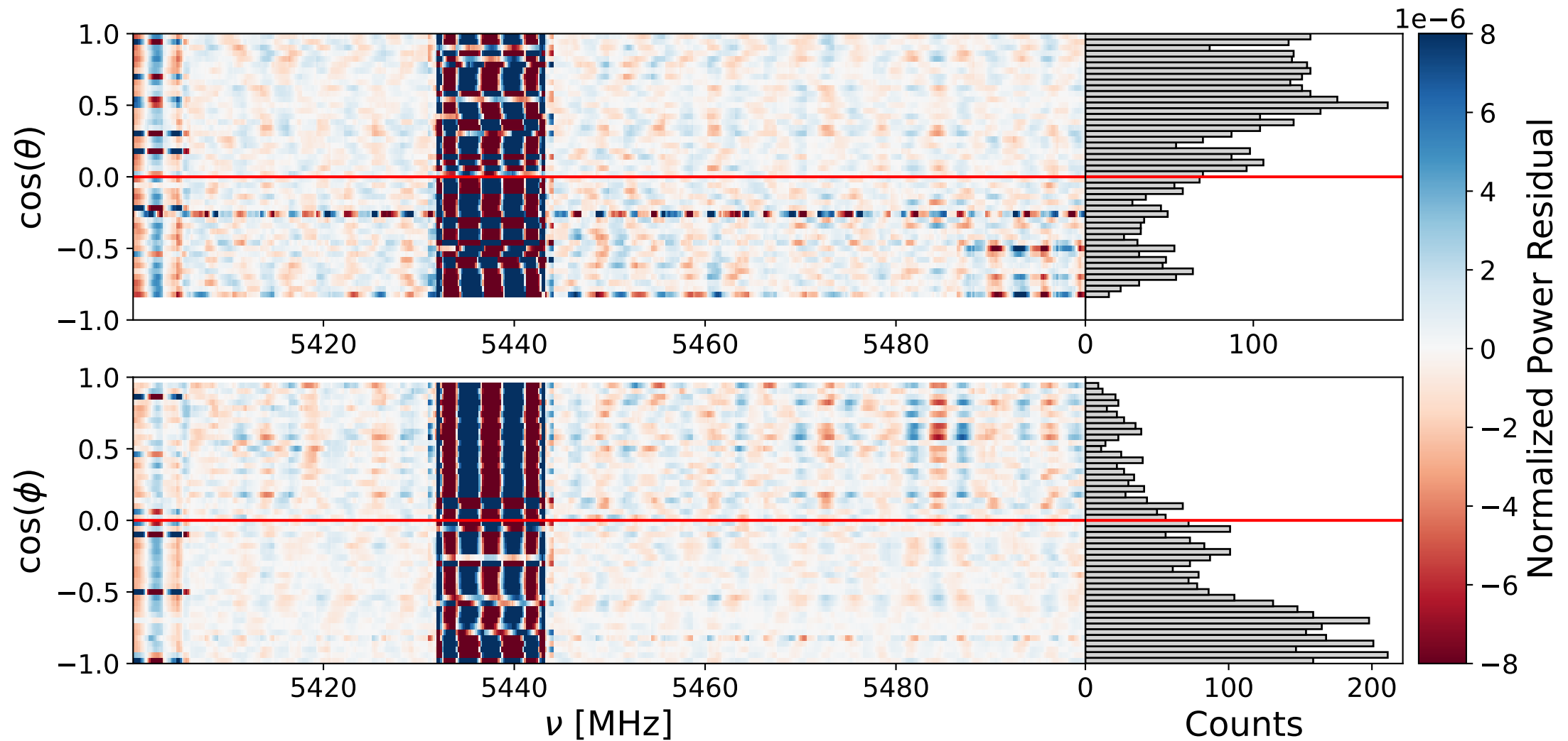
Bank 1 ann: 5400-5500 MHz
