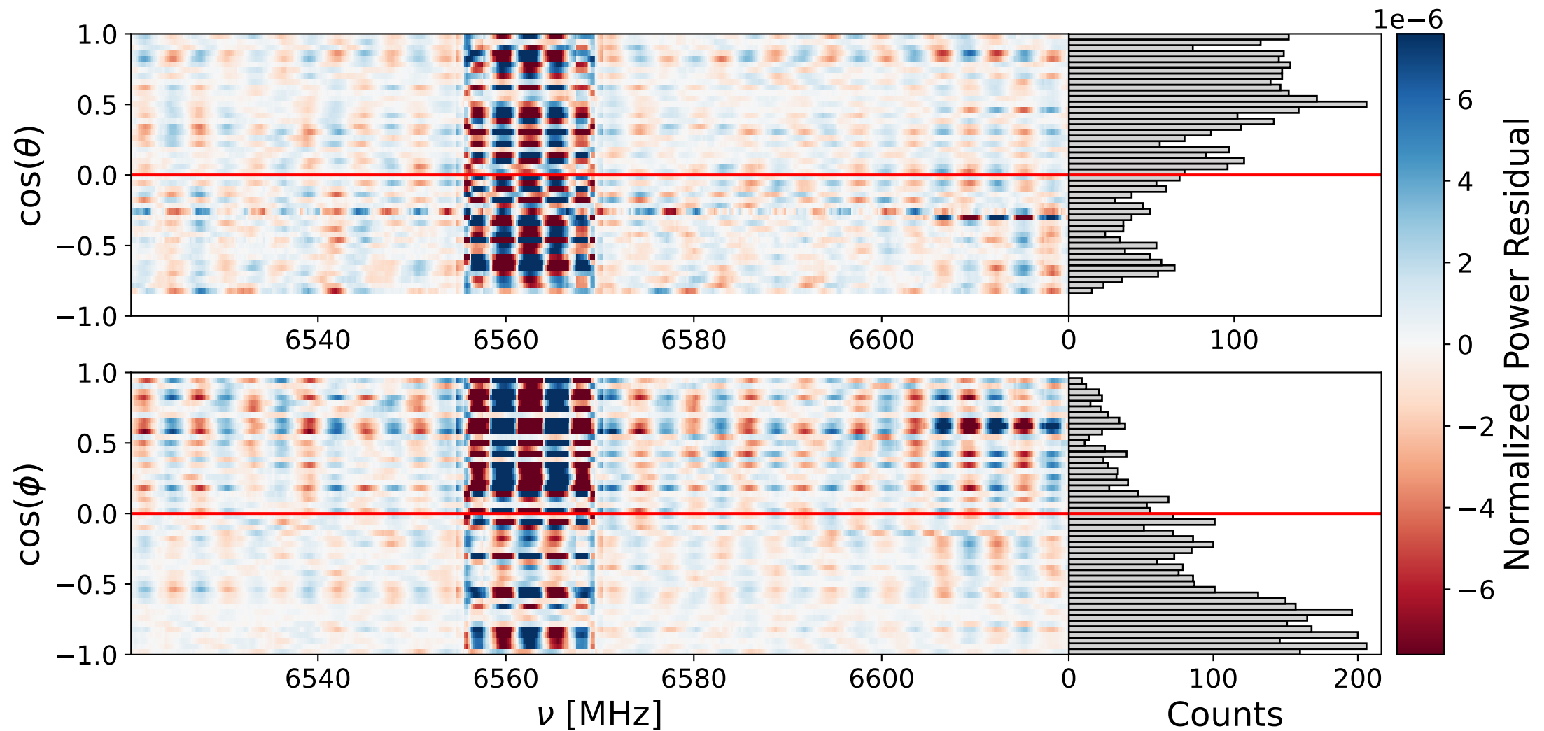
Bank 2 ann: 6520-6620 MHz
