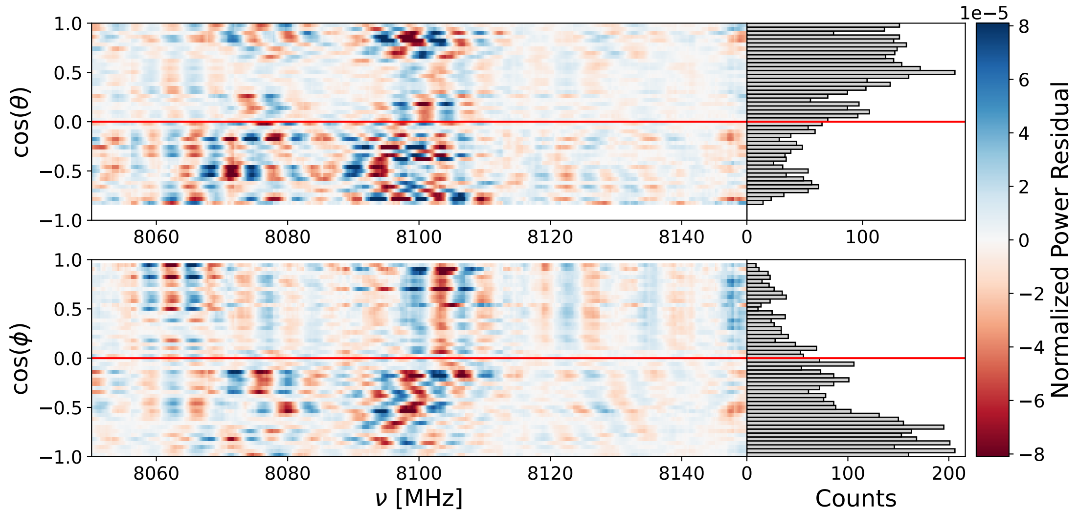
Bank 3 ann: 8050-8150 MHz
