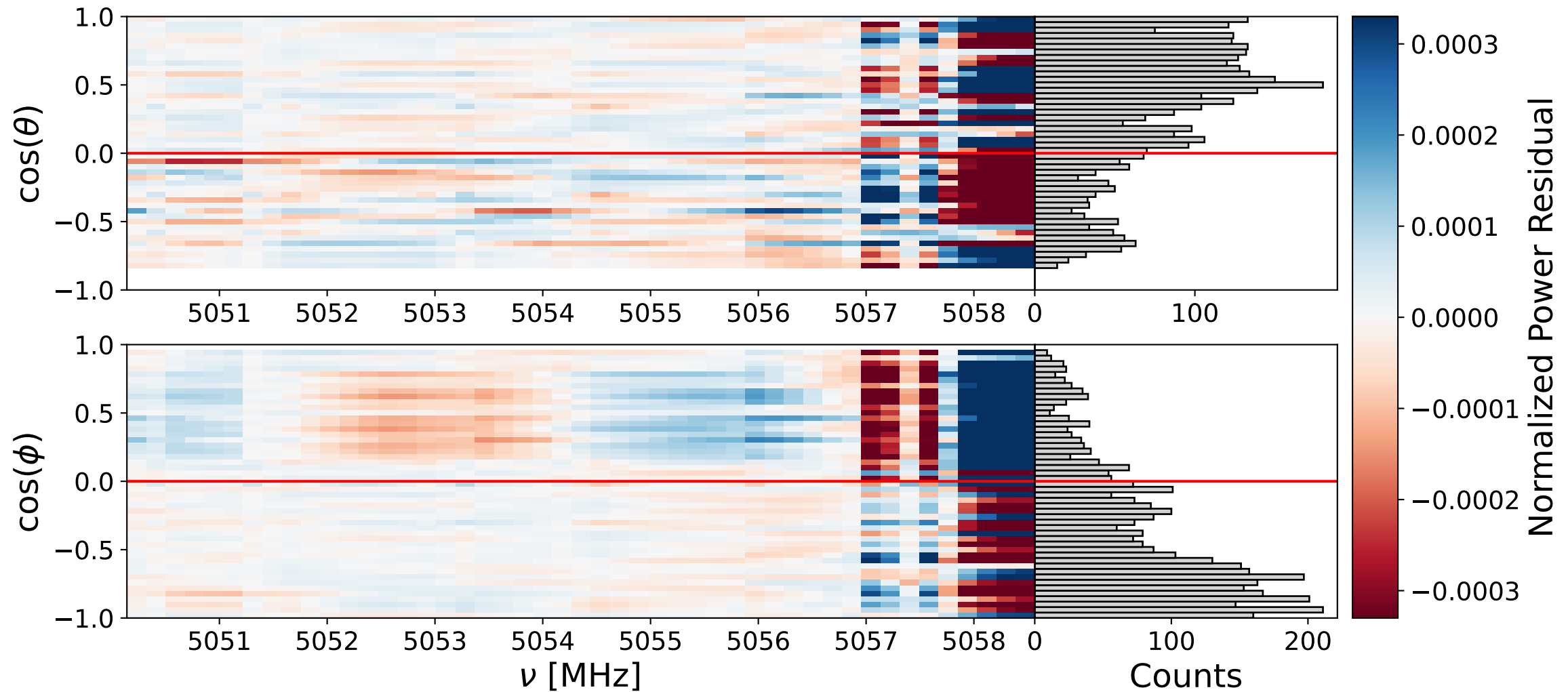
Bank 0 ann: 5050-5059 MHz
