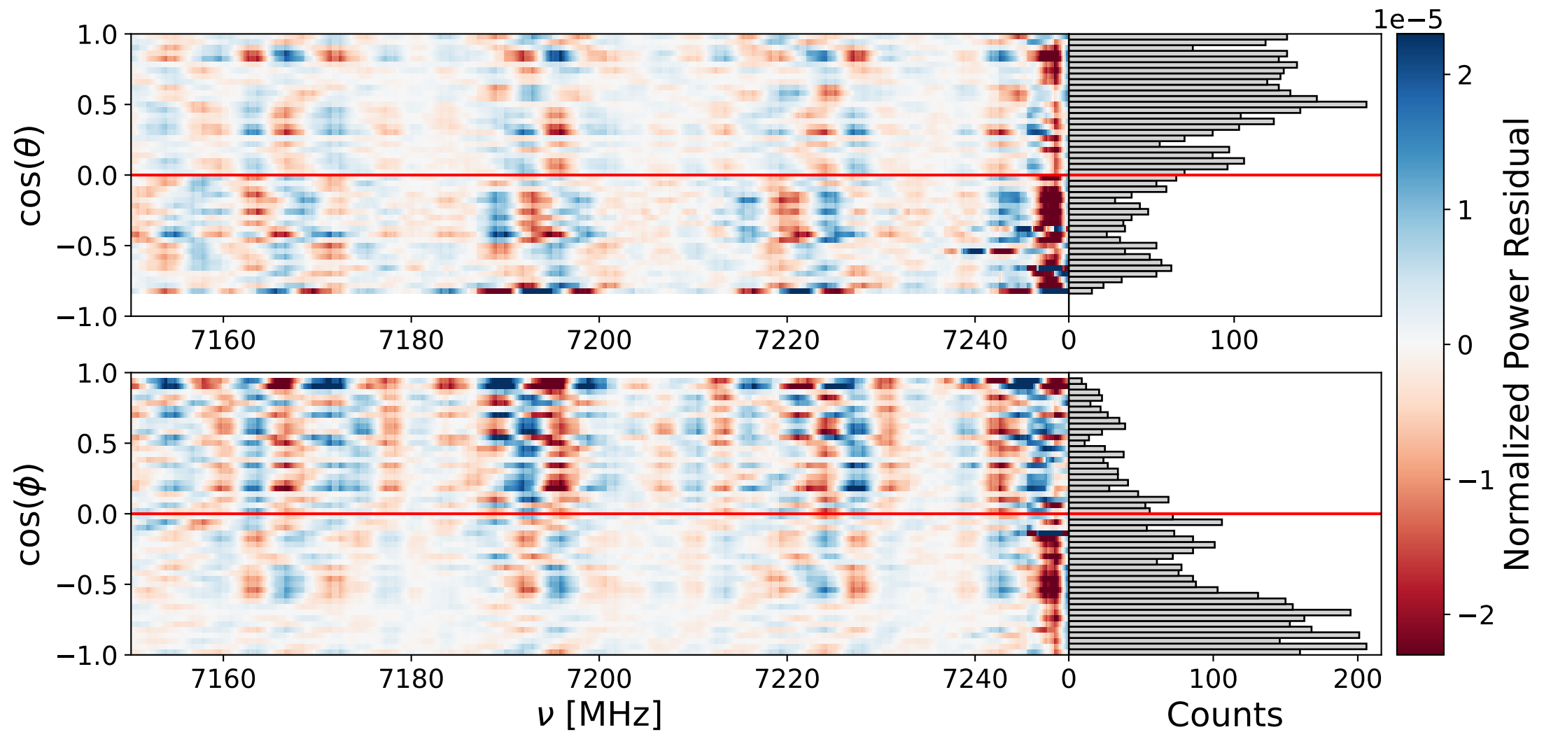
Bank 3 ann: 7150-7250 MHz
