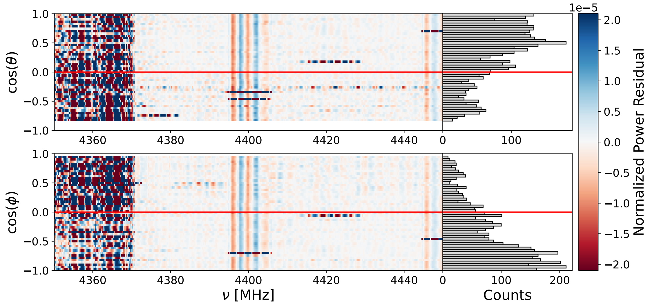
Bank 0 ann: 4350-4450 MHz
