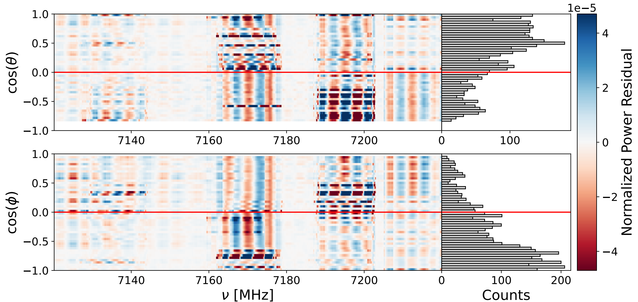
Bank 2 ann: 7120-7220 MHz
