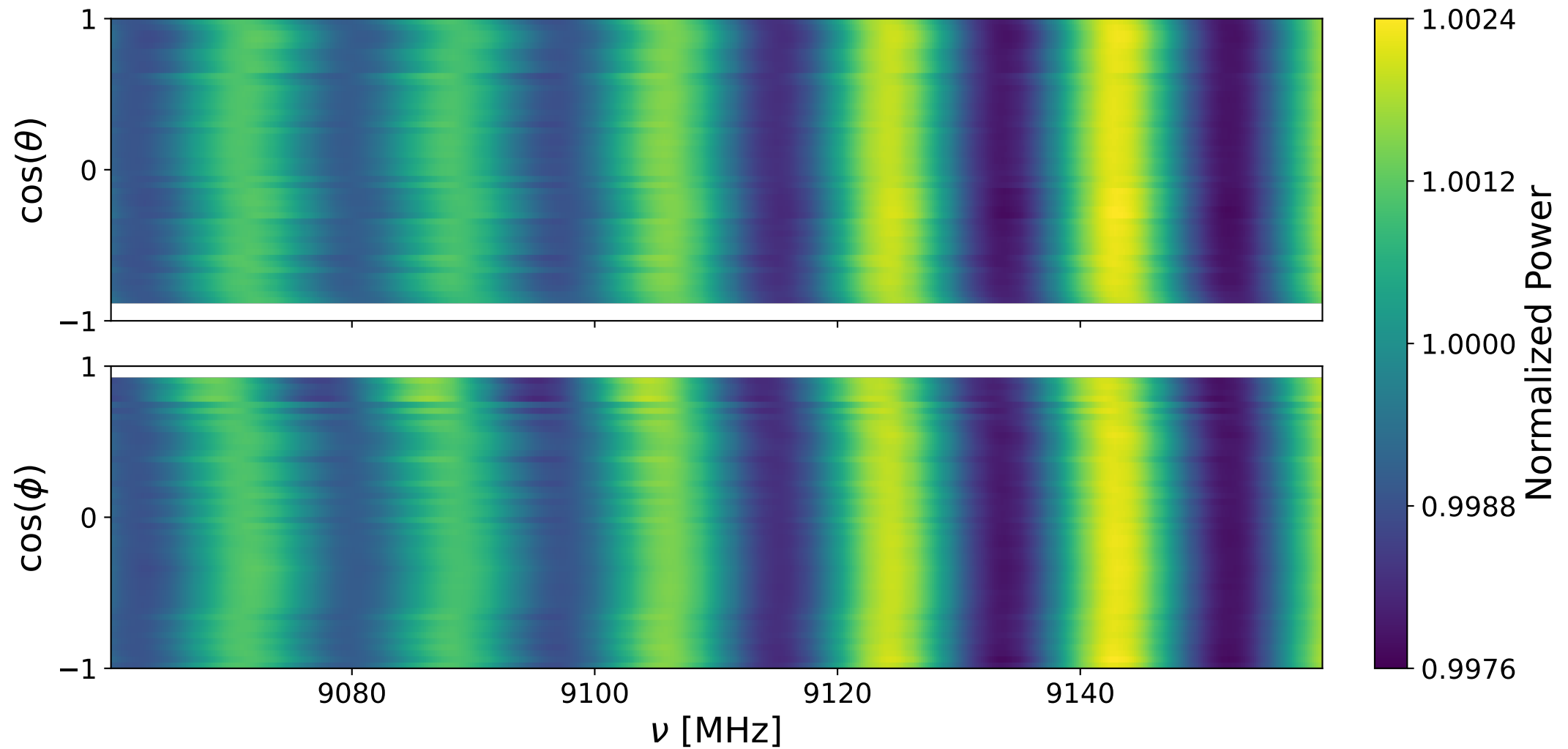
Bank 1 ann: 9060-9160 MHz
