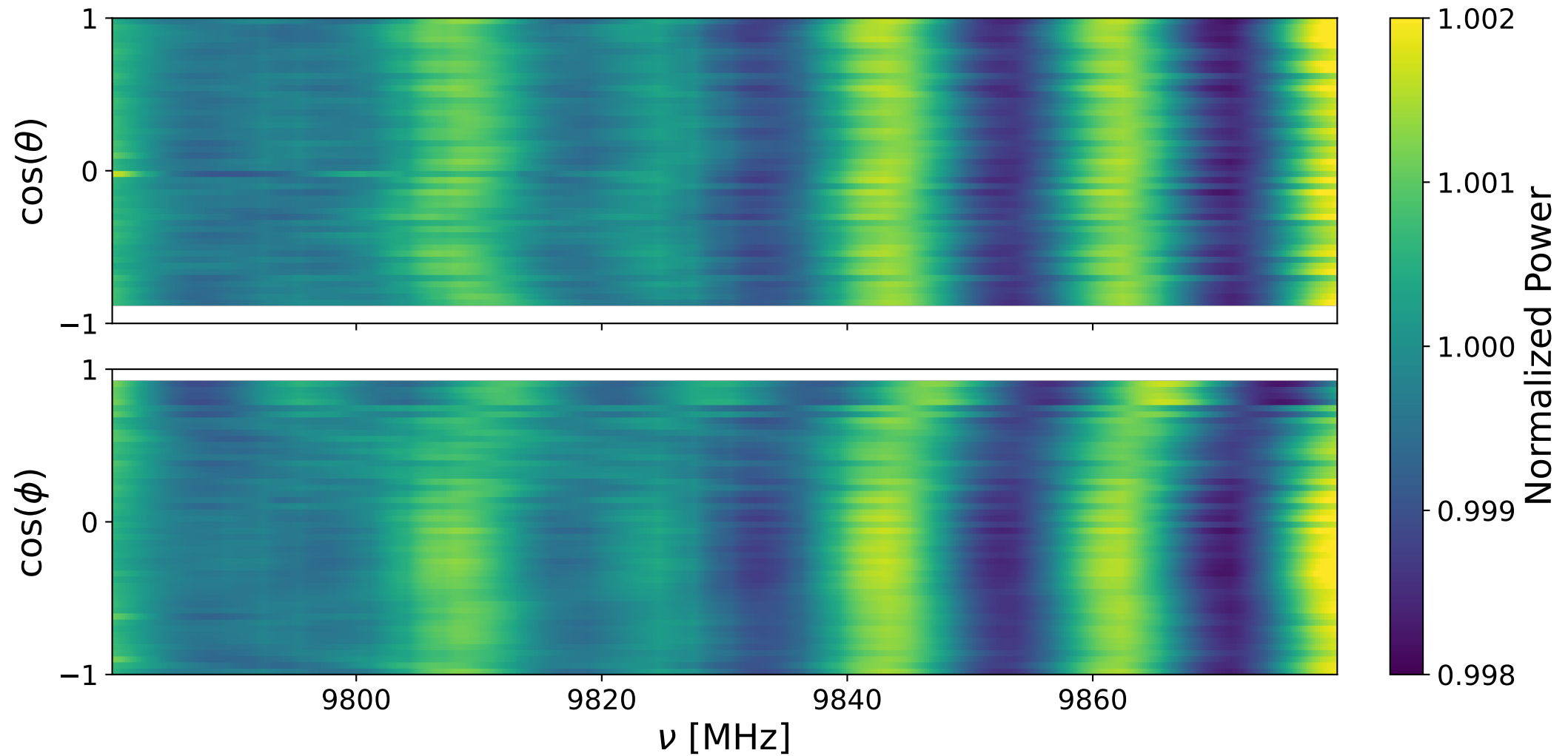
Bank 2 ann: 9780-9880 MHz
