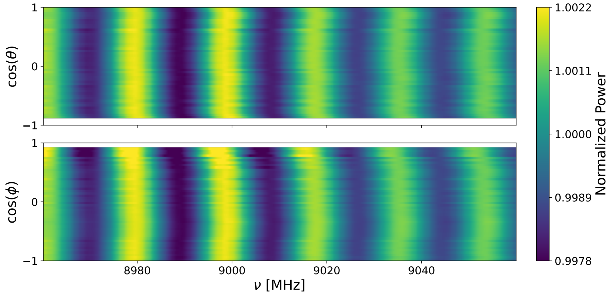
Bank 1 ann: 8960-9060 MHz
