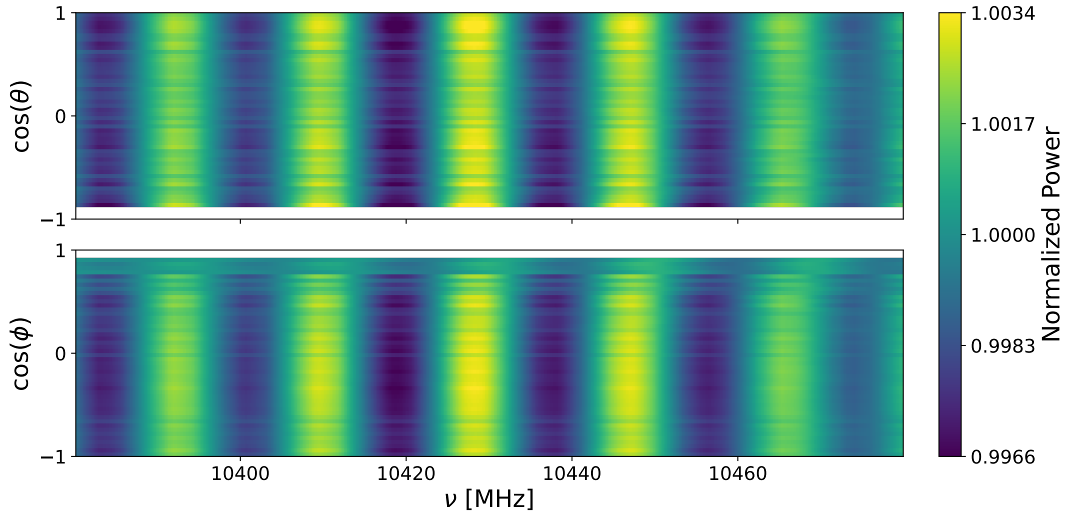
Bank 2 ann: 10380-10480 MHz
