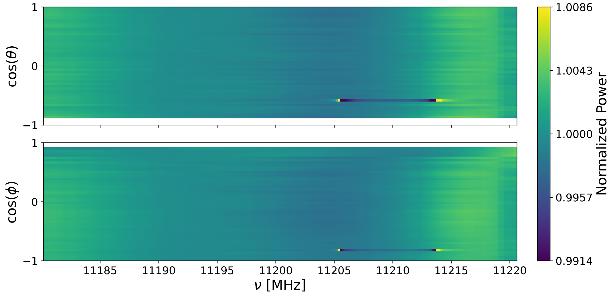
Bank 2 ann: 11180-11221 MHz
