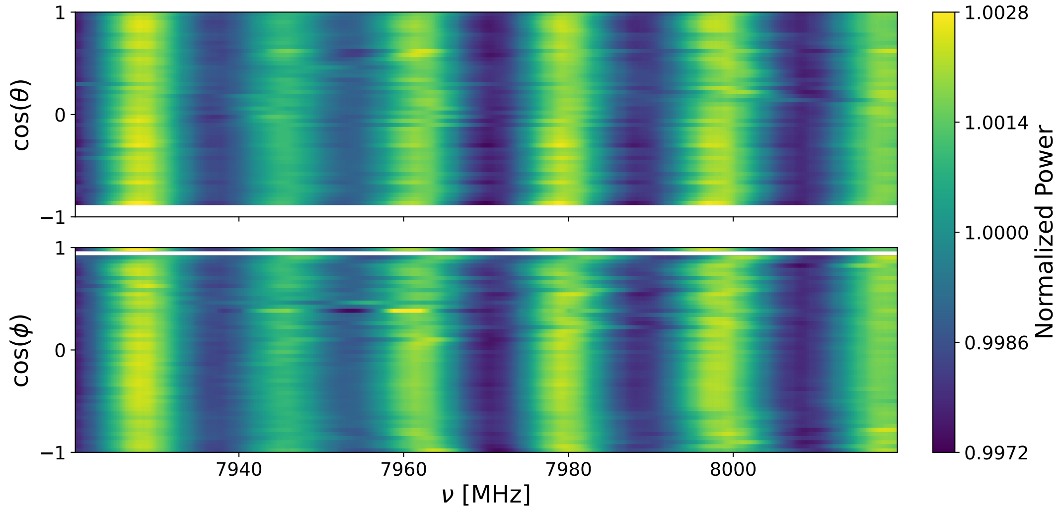
Bank 0 ann: 7920-8020 MHz
