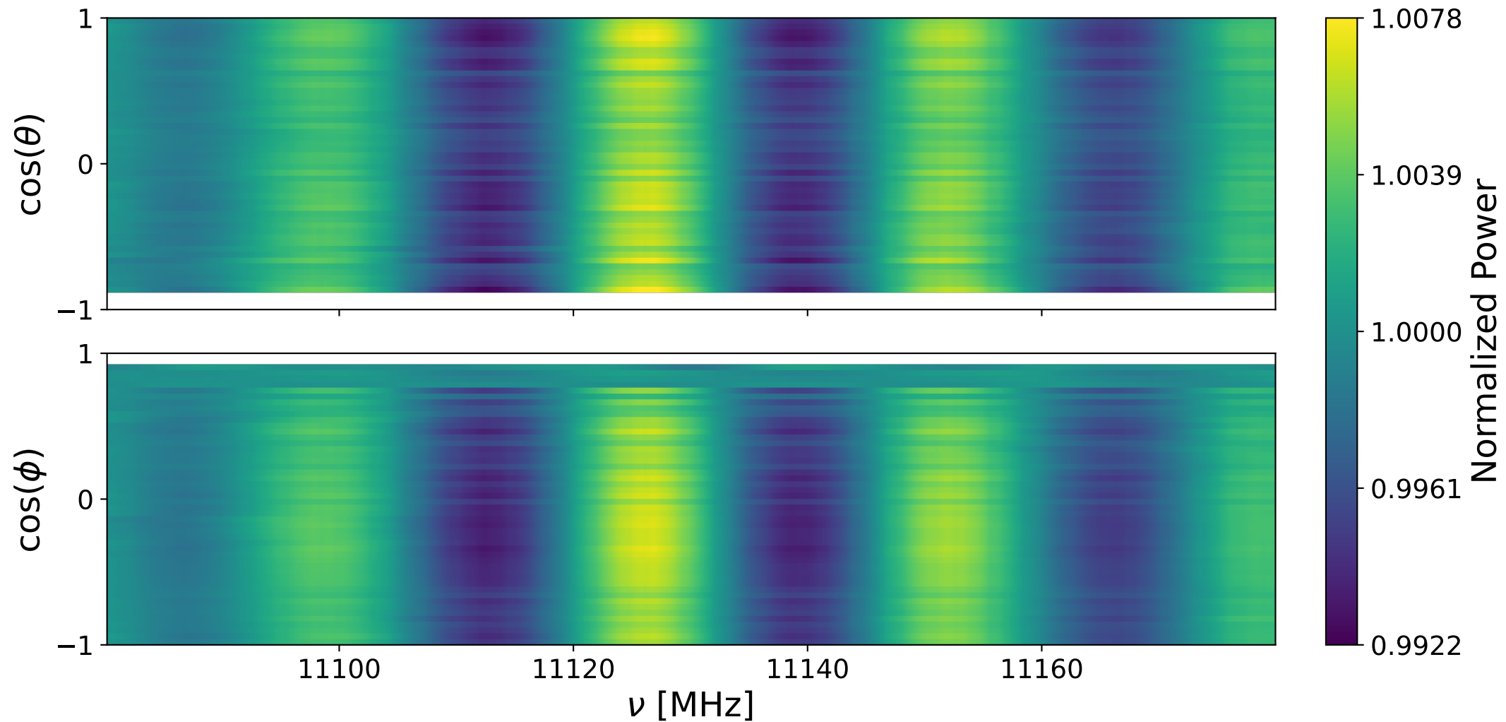
Bank 2 ann: 11080-11180 MHz
