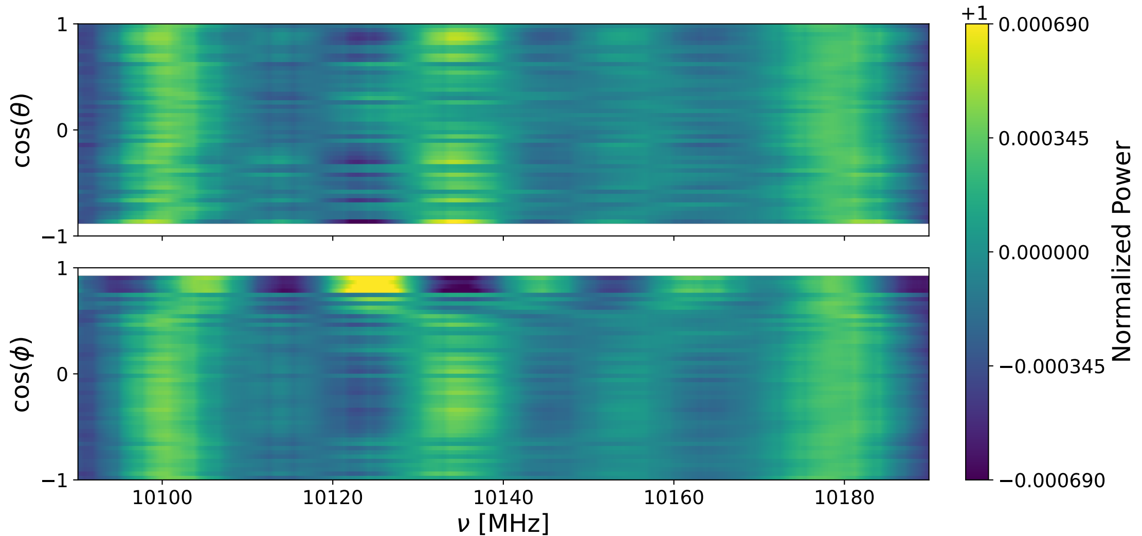
Bank 2 decay: 10090-10190 MHz
