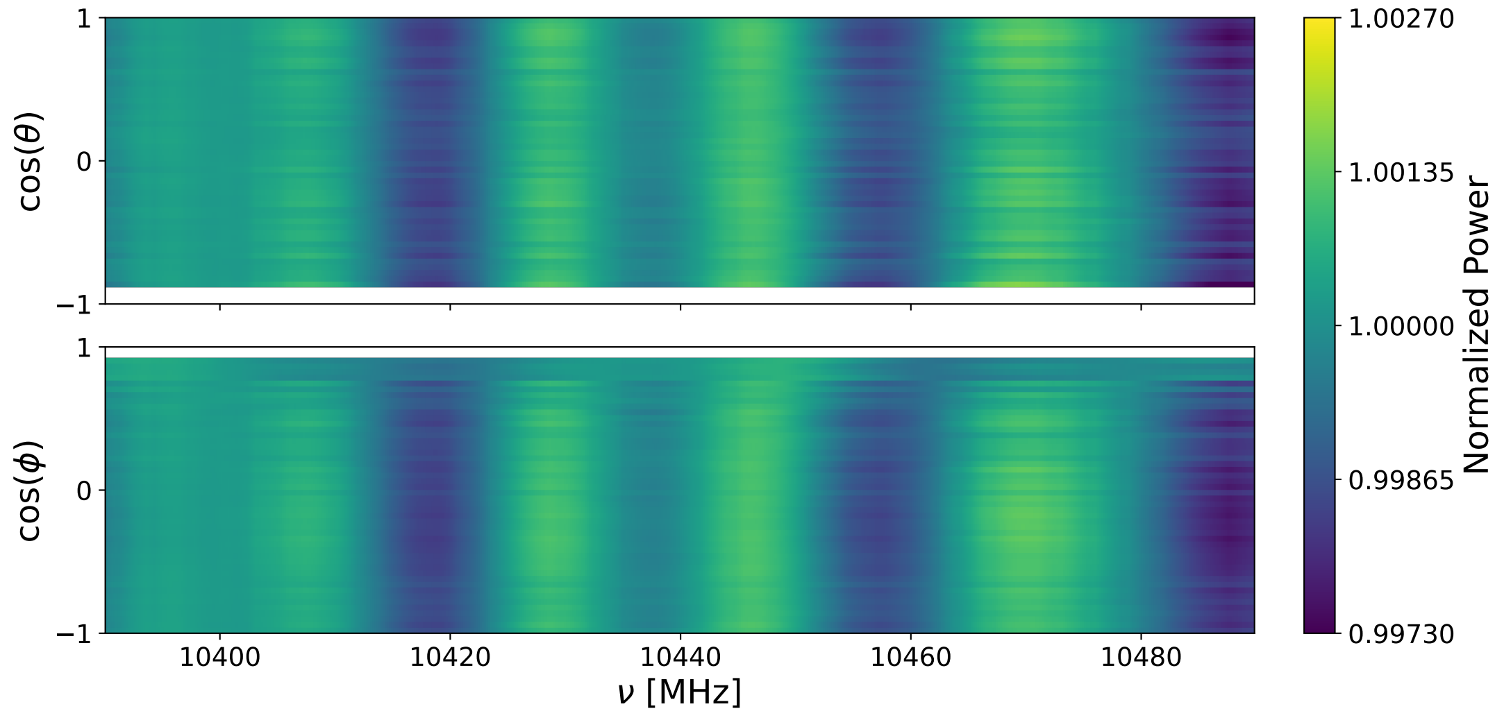
Bank 2 decay: 10390-10490 MHz
