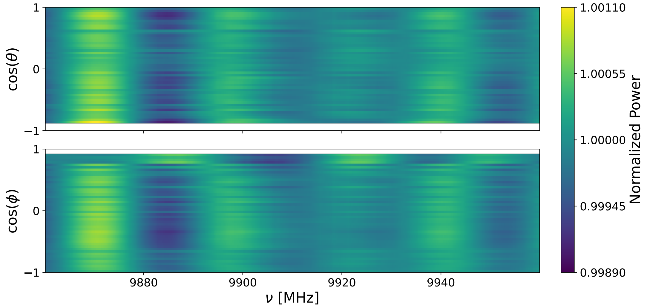
Bank 1 decay: 9860-9960 MHz
