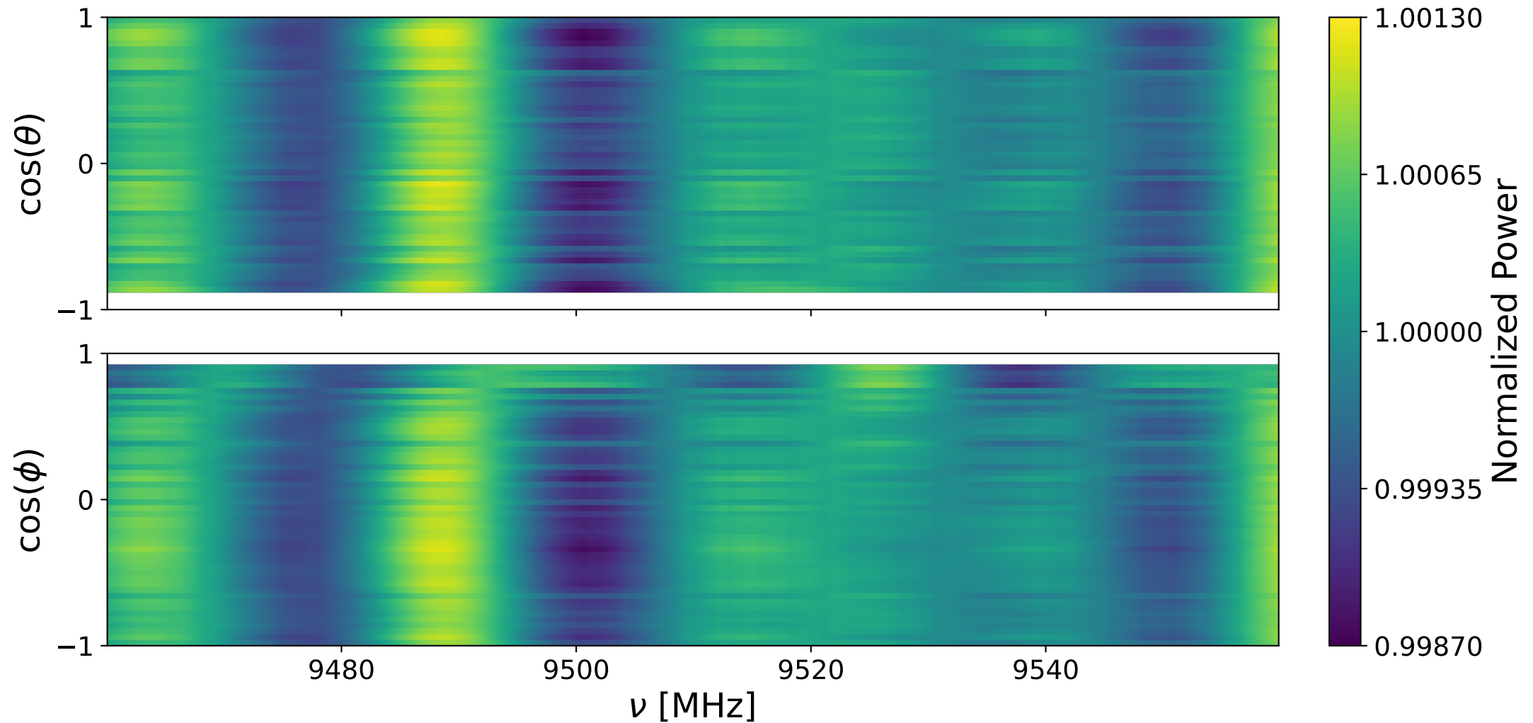
Bank 1 decay: 9460-9560 MHz
