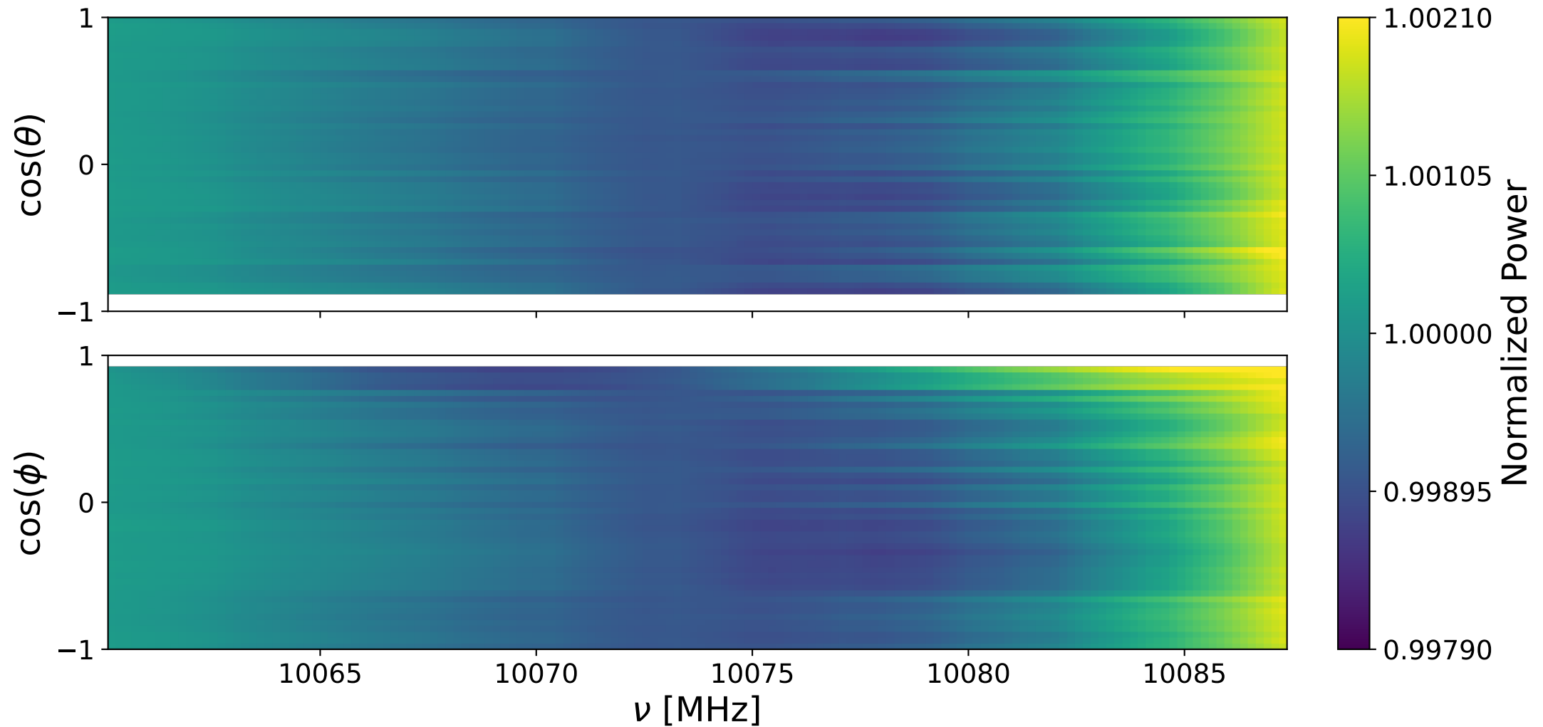
Bank 1 decay: 10060-10087 MHz
