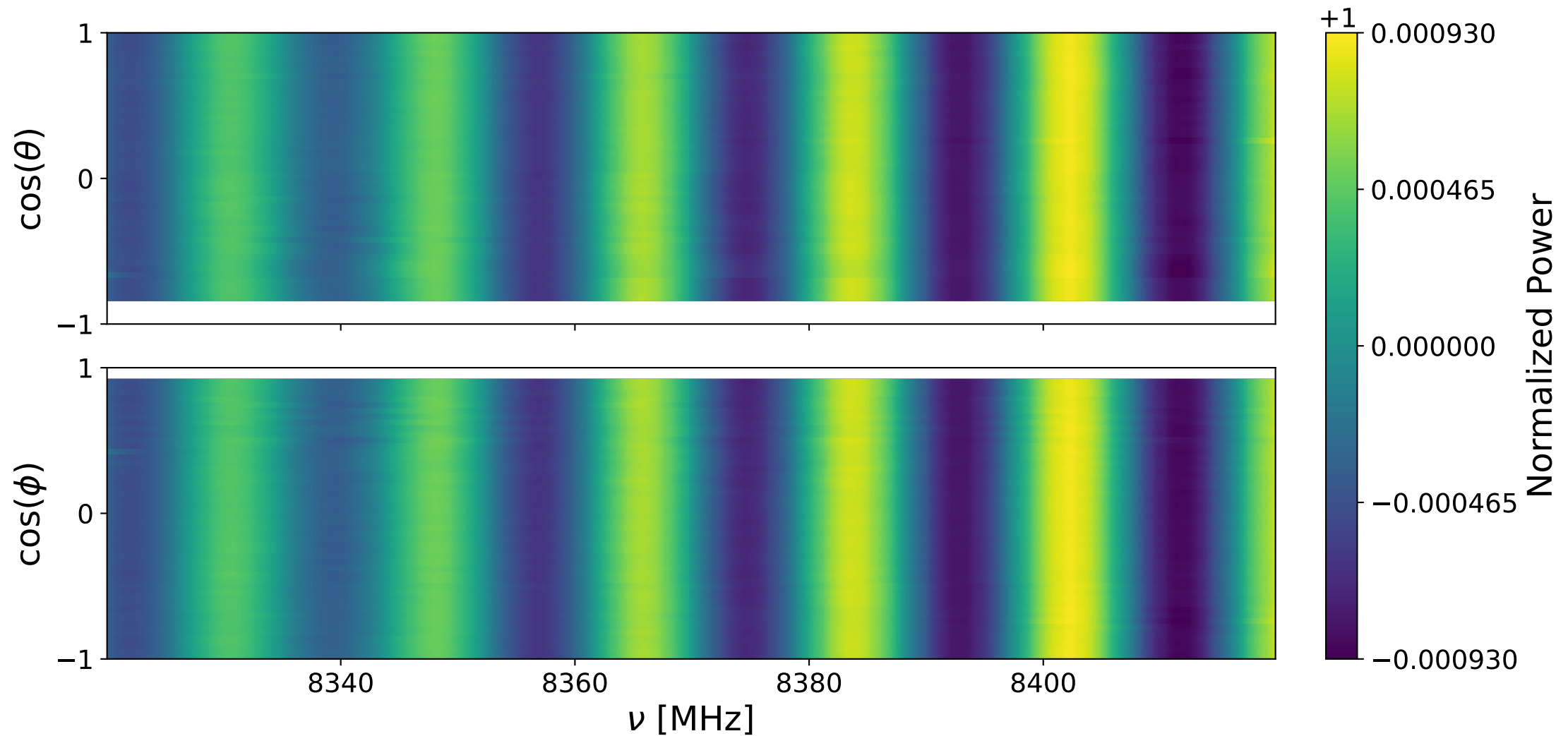
Bank 0 ann: 8320-8420 MHz
