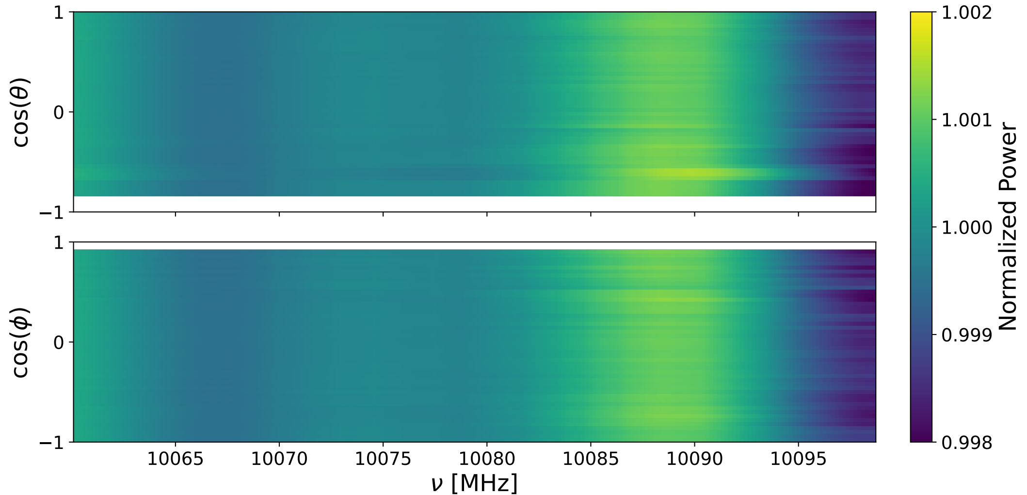
Bank 1 ann: 10060-10099 MHz
