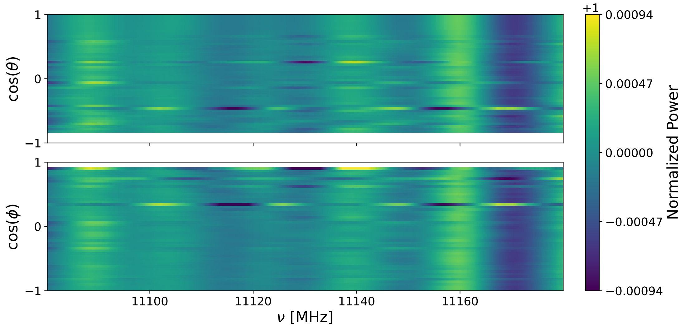
Bank 2 ann: 11080-11180 MHz
