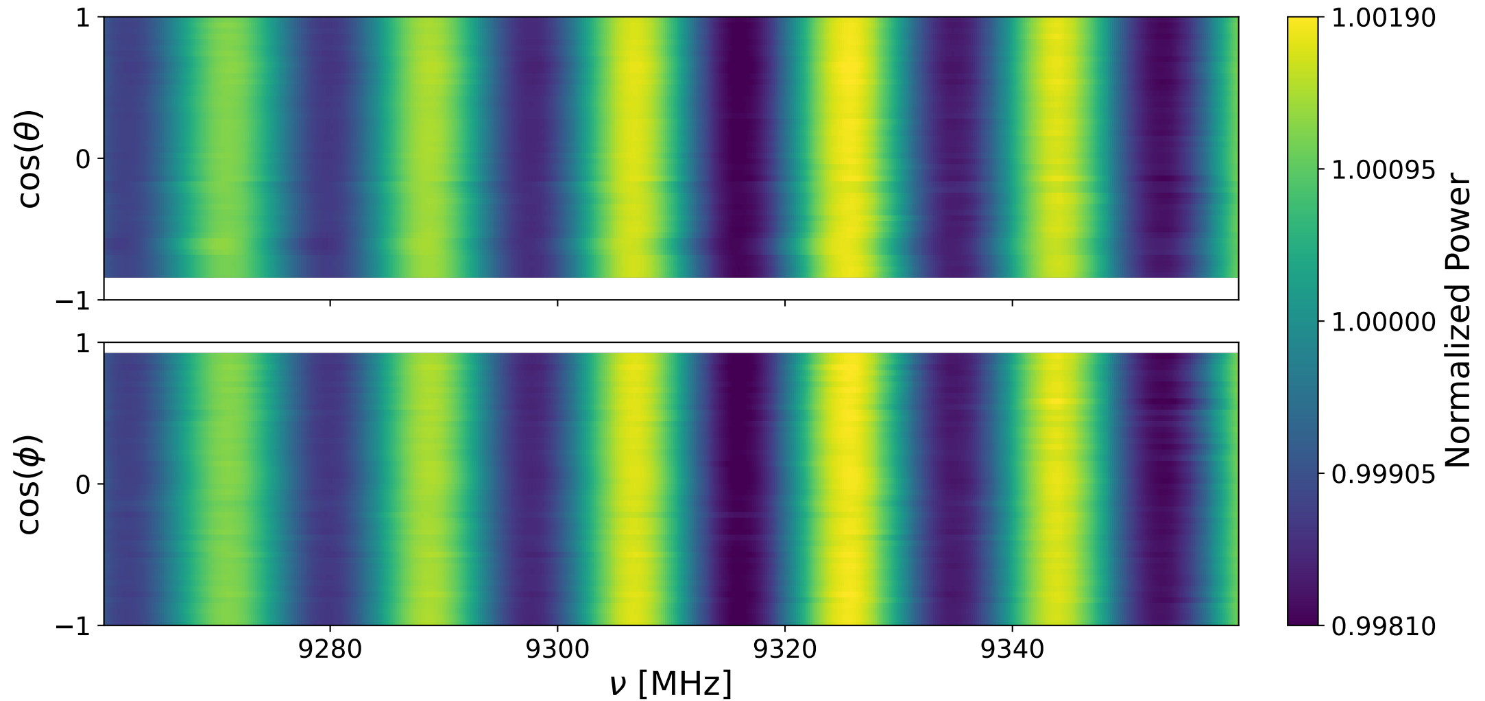
Bank 1 ann: 9260-9360 MHz
