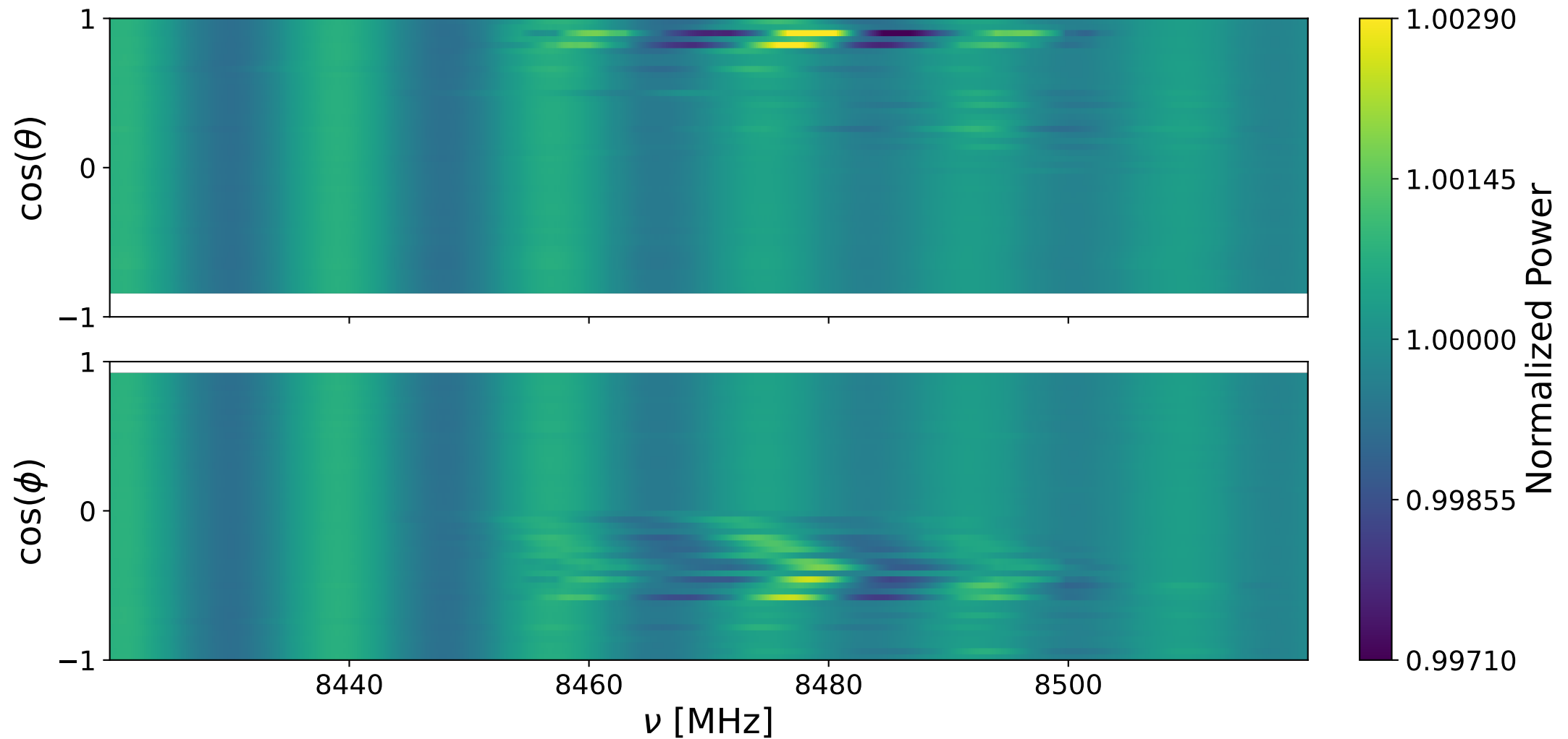
Bank 0 ann: 8420-8520 MHz
