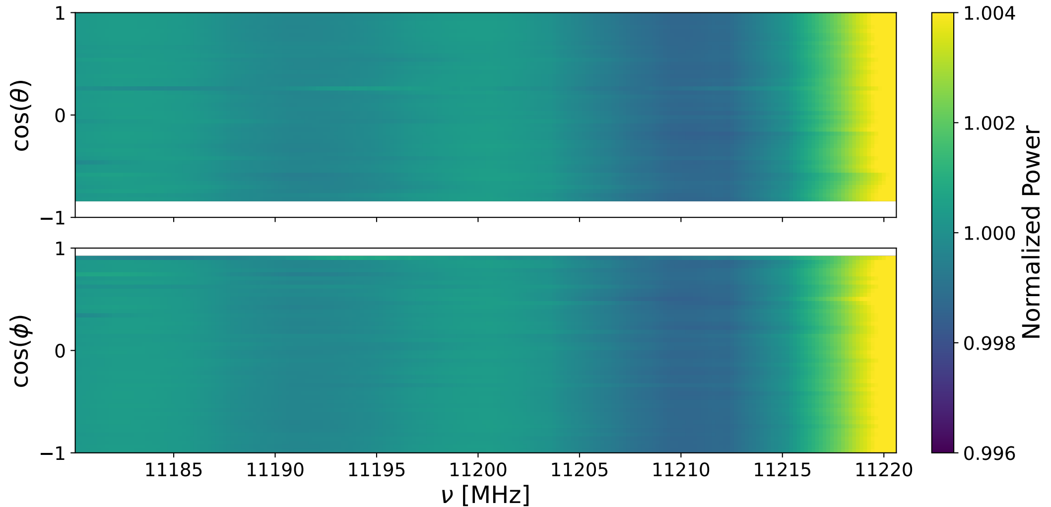
Bank 2 ann: 11180-11221 MHz
