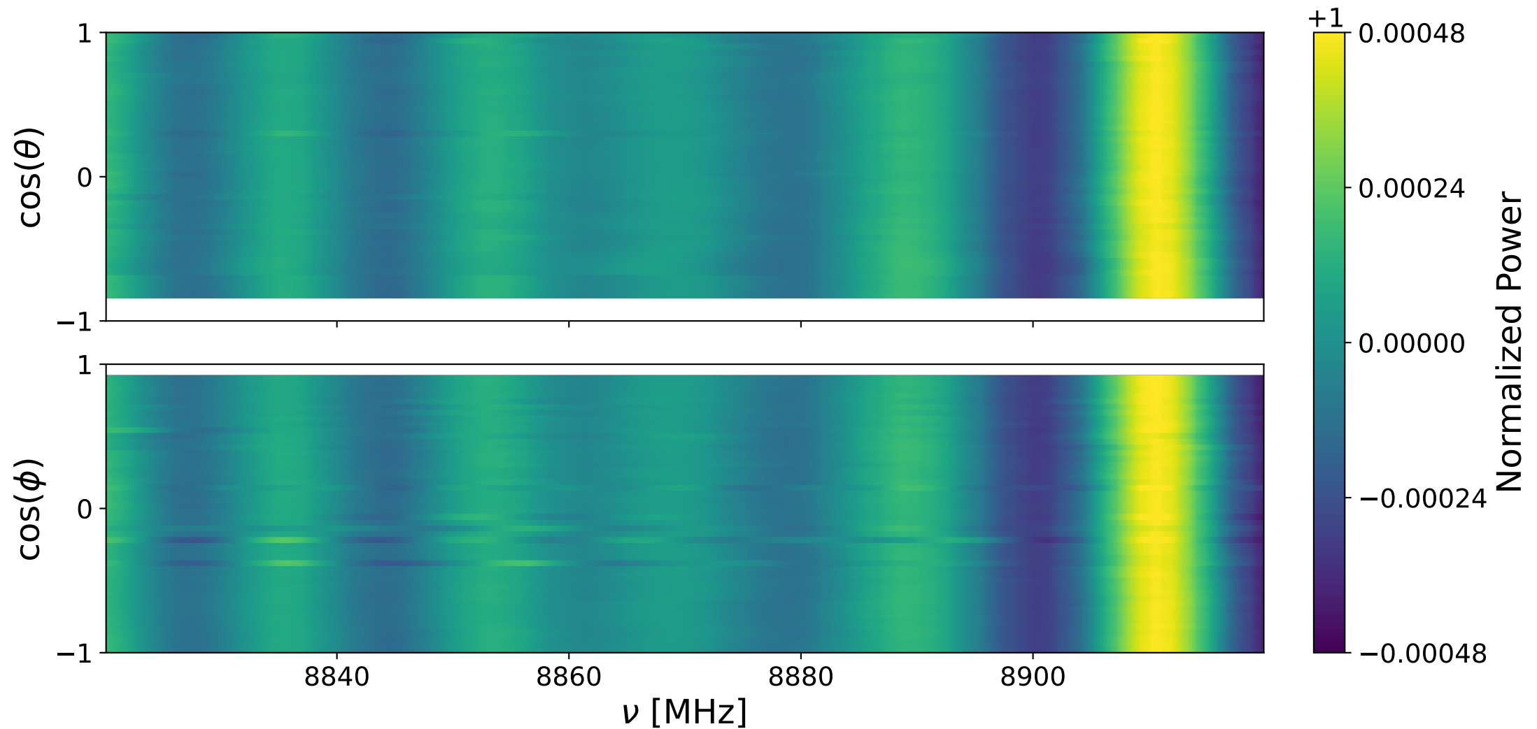
Bank 0 ann: 8820-8920 MHz
