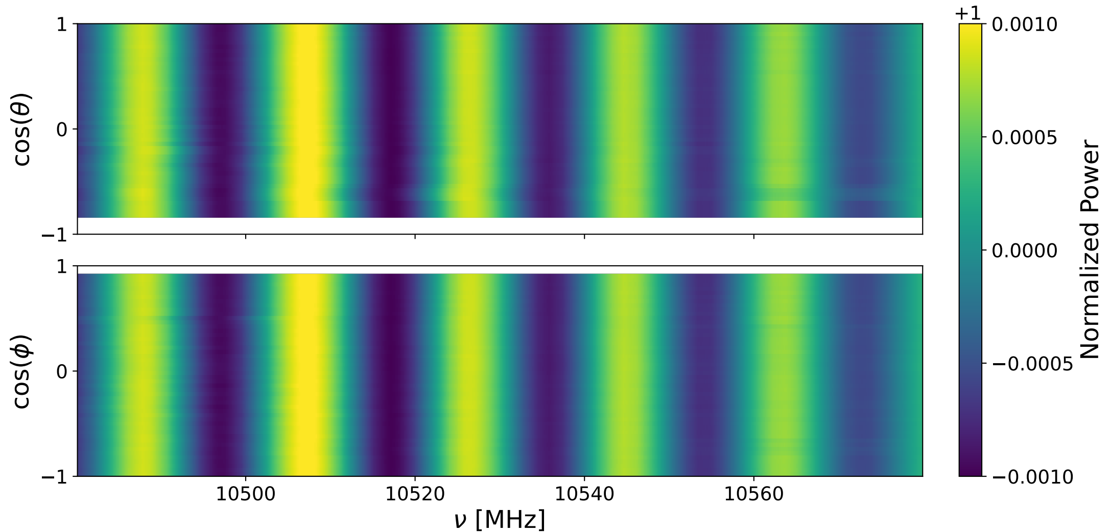
Bank 2 ann: 10480-10580 MHz
