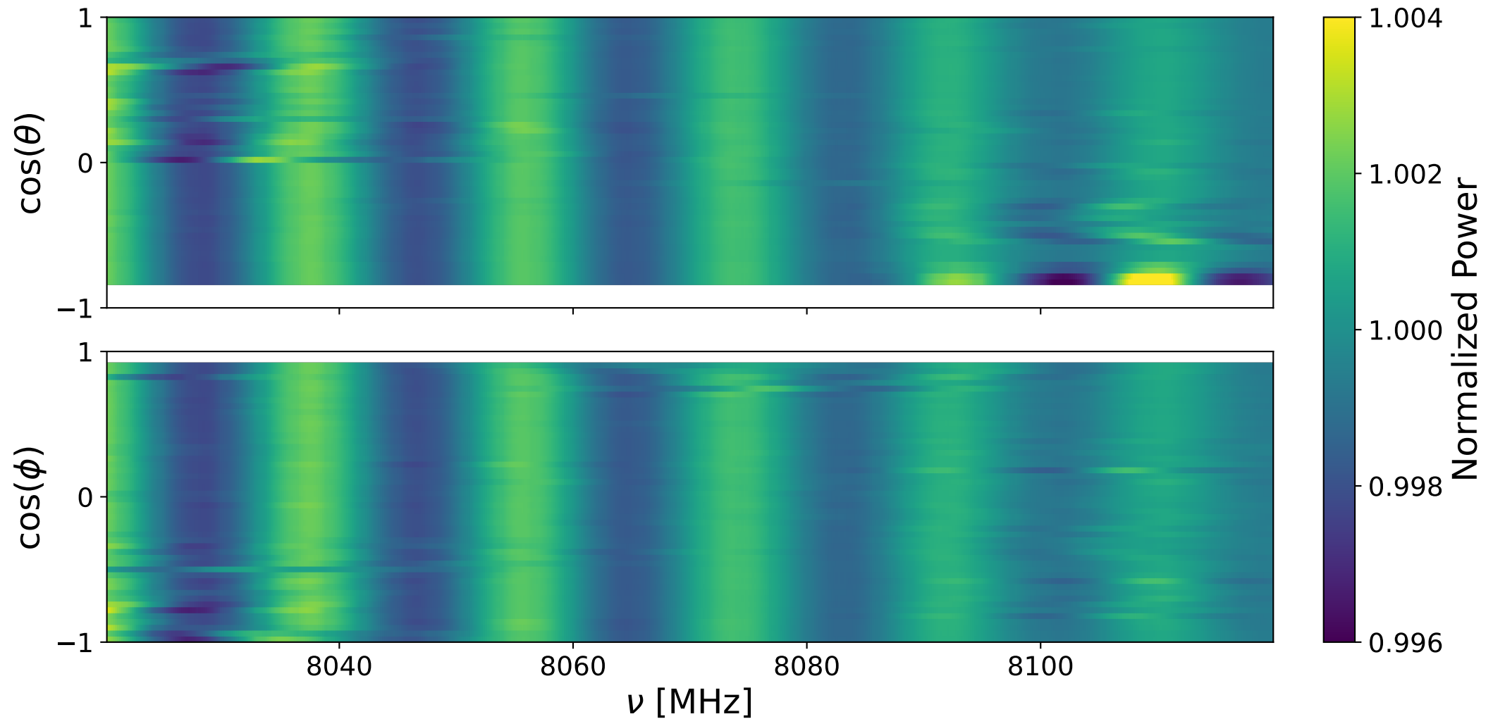
Bank 0 ann: 8020-8120 MHz
