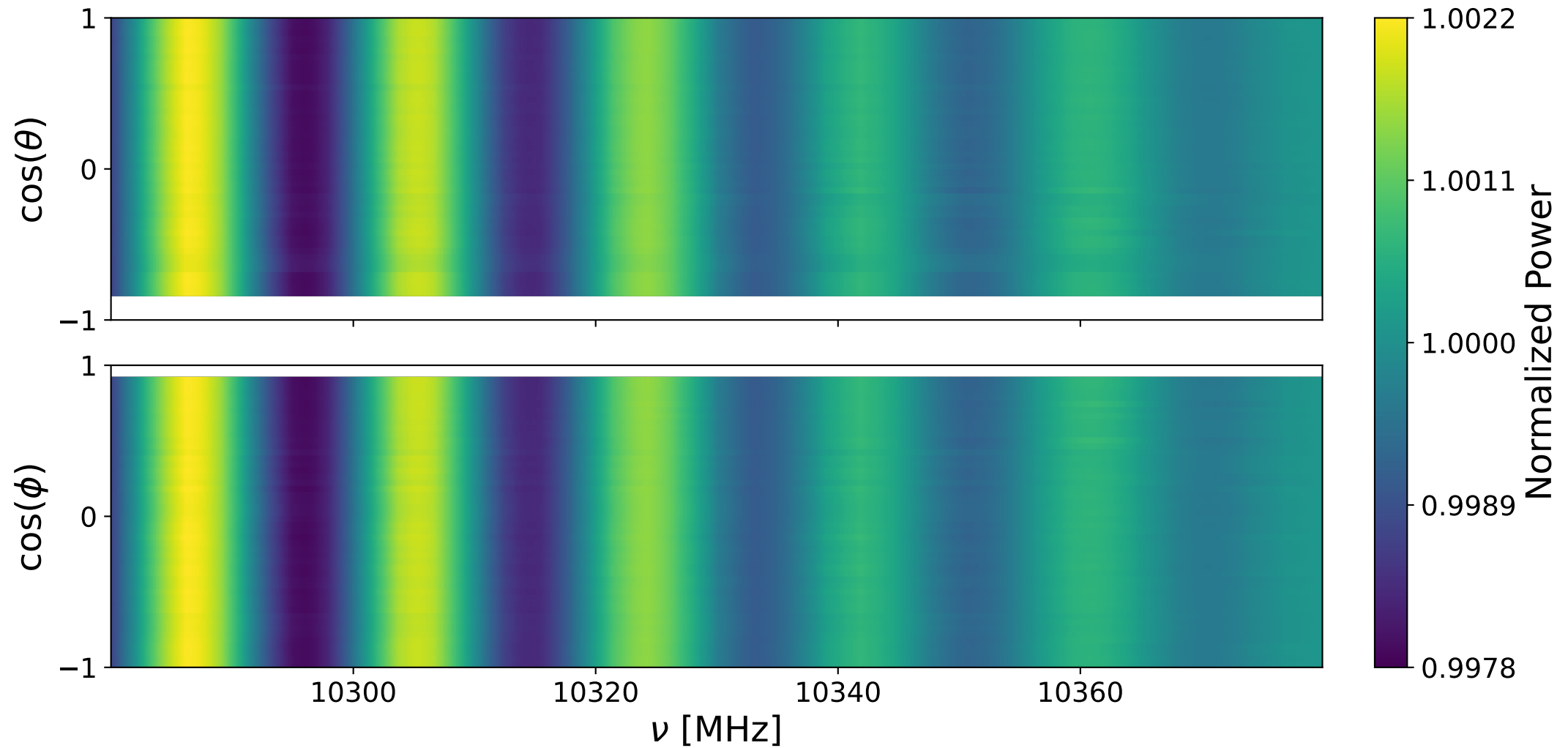
Bank 2 ann: 10280-10380 MHz
