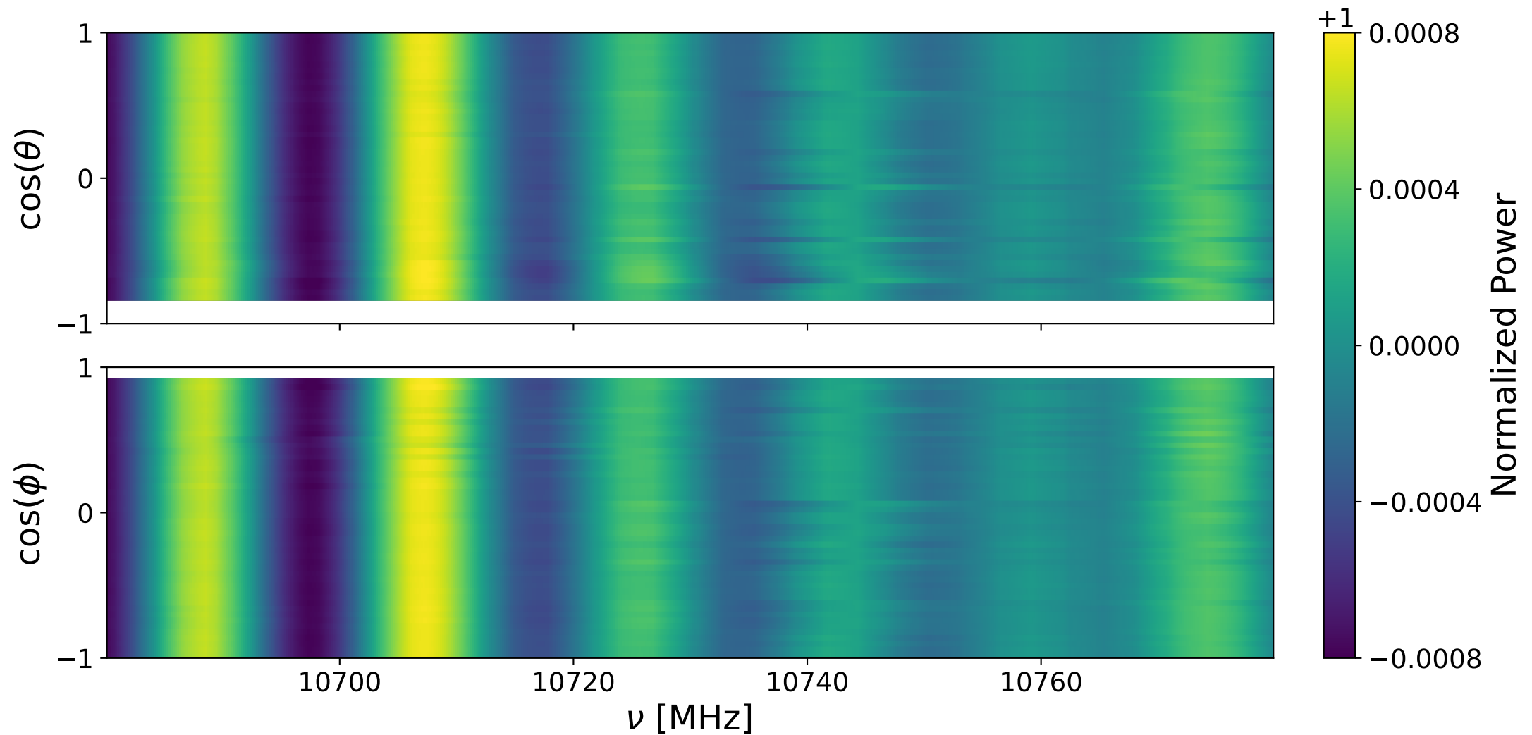
Bank 2 ann: 10680-10780 MHz
