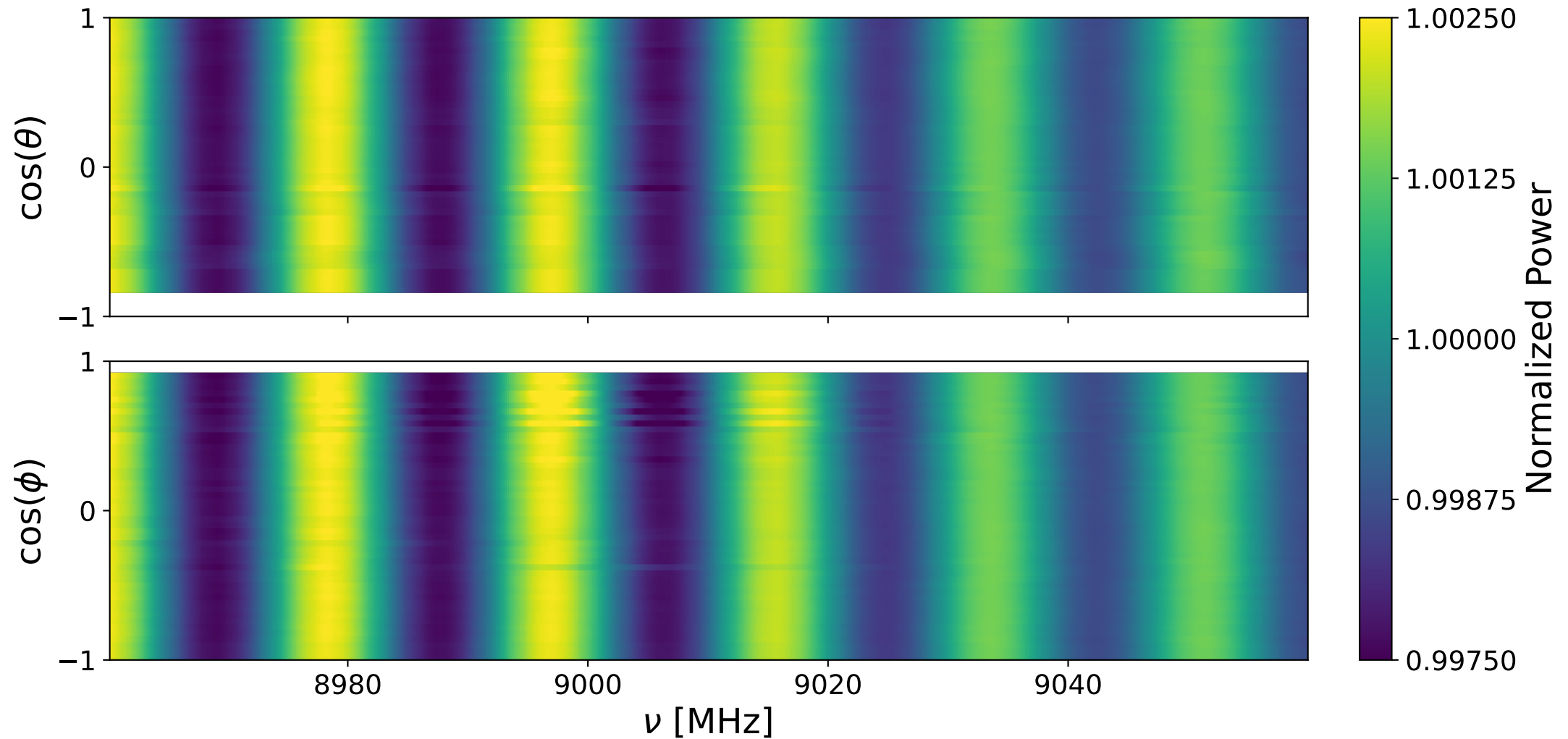
Bank 1 ann: 8960-9060 MHz
