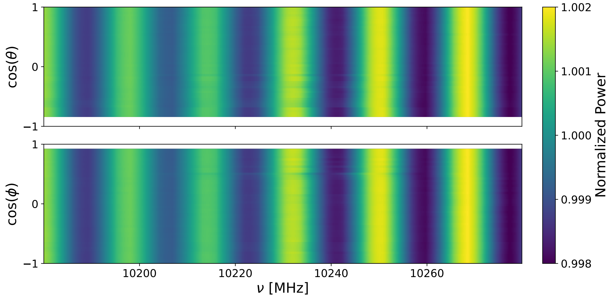
Bank 2 ann: 10180-10280 MHz
