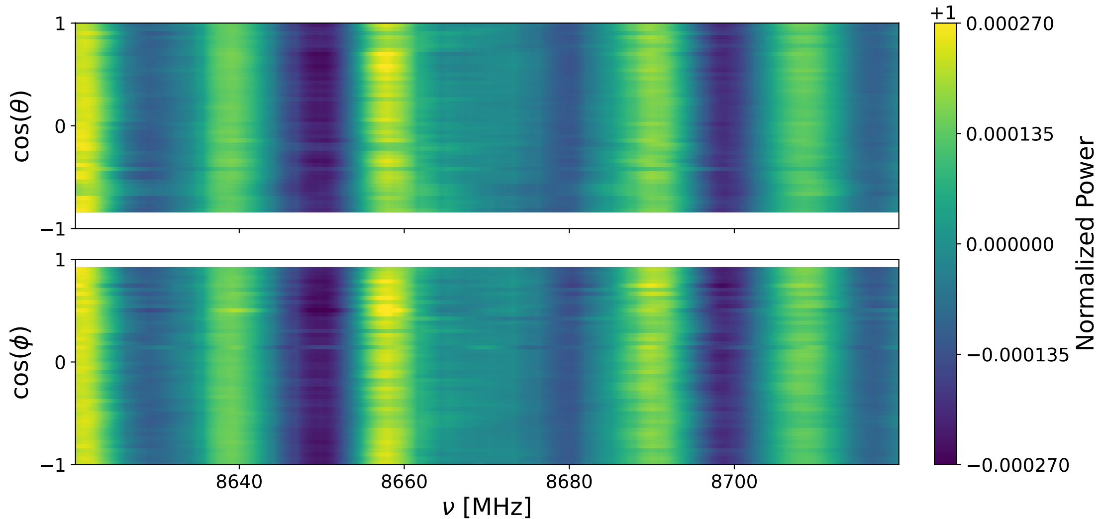
Bank 0 ann: 8620-8720 MHz
