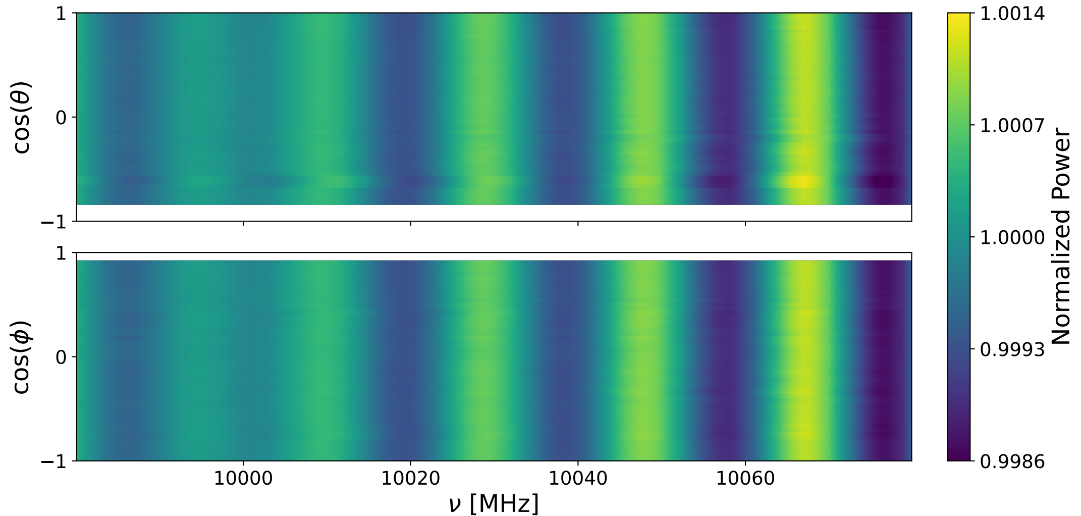
Bank 2 ann: 9980-10080 MHz
