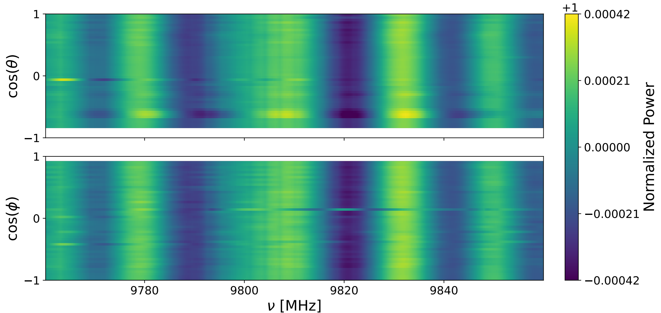
Bank 1 ann: 9760-9860 MHz
