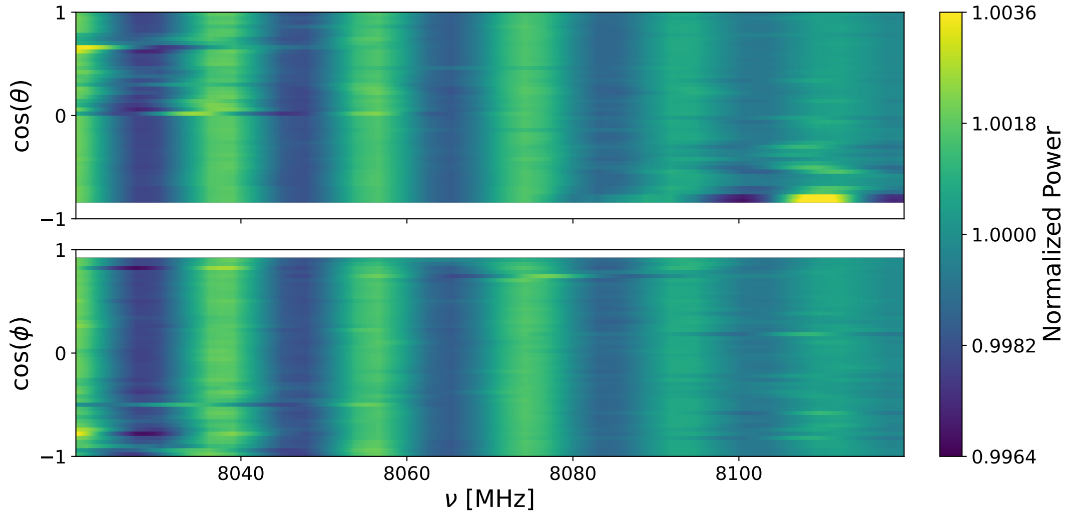
Bank 0 decay: 8020-8120 MHz
