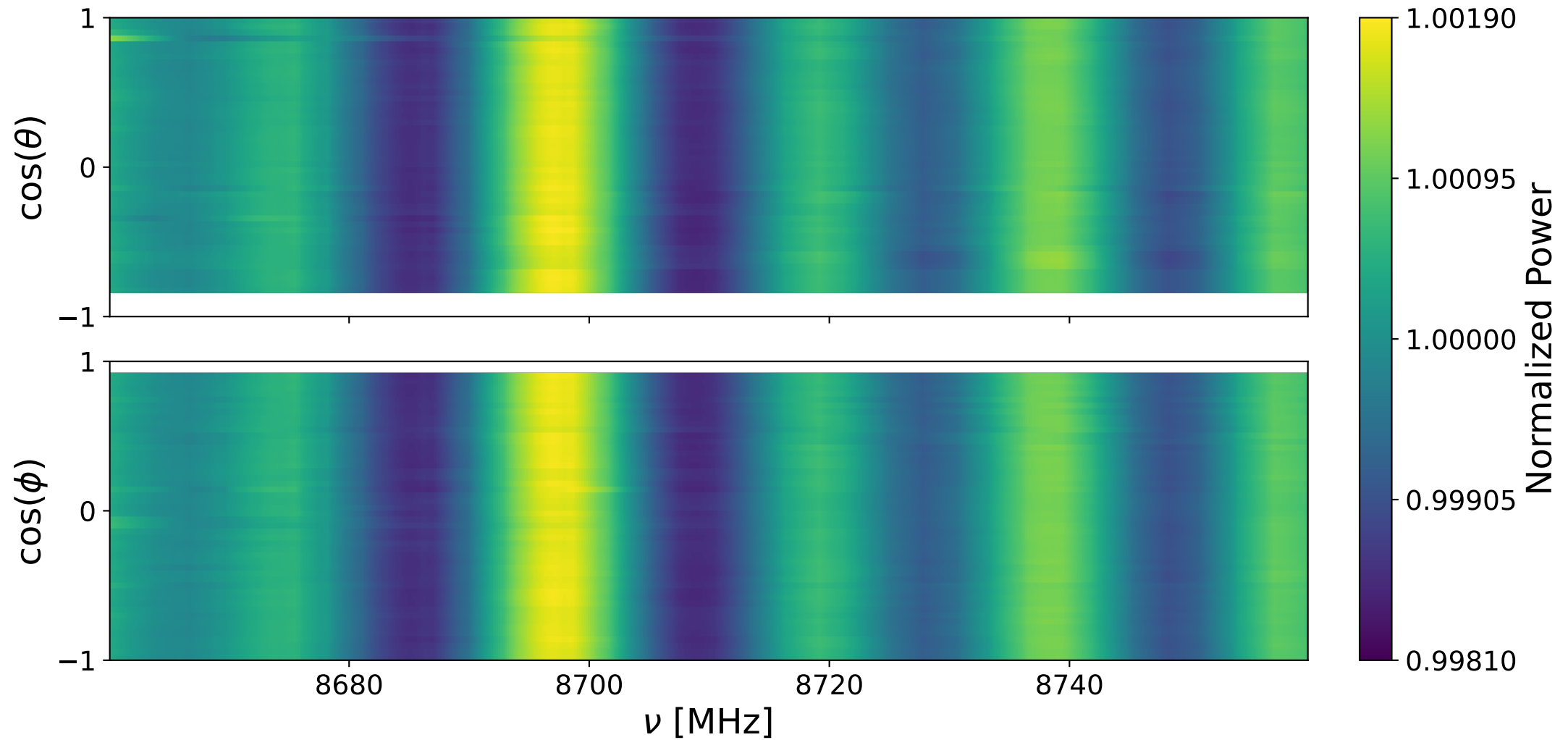
Bank 1 decay: 8660-8760 MHz
