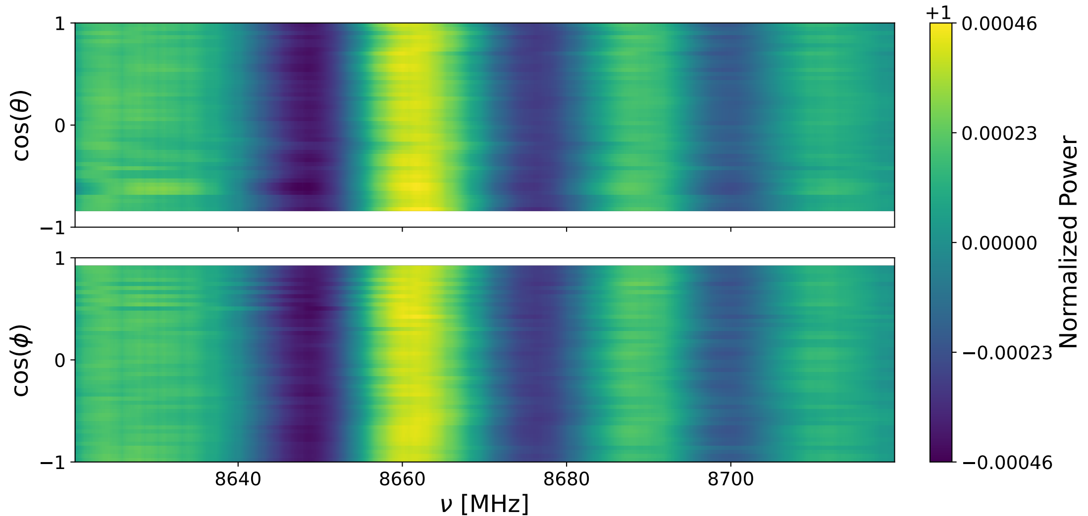
Bank 0 decay: 8620-8720 MHz
