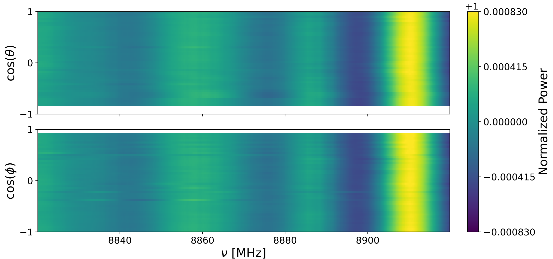
Bank 0 decay: 8820-8920 MHz
