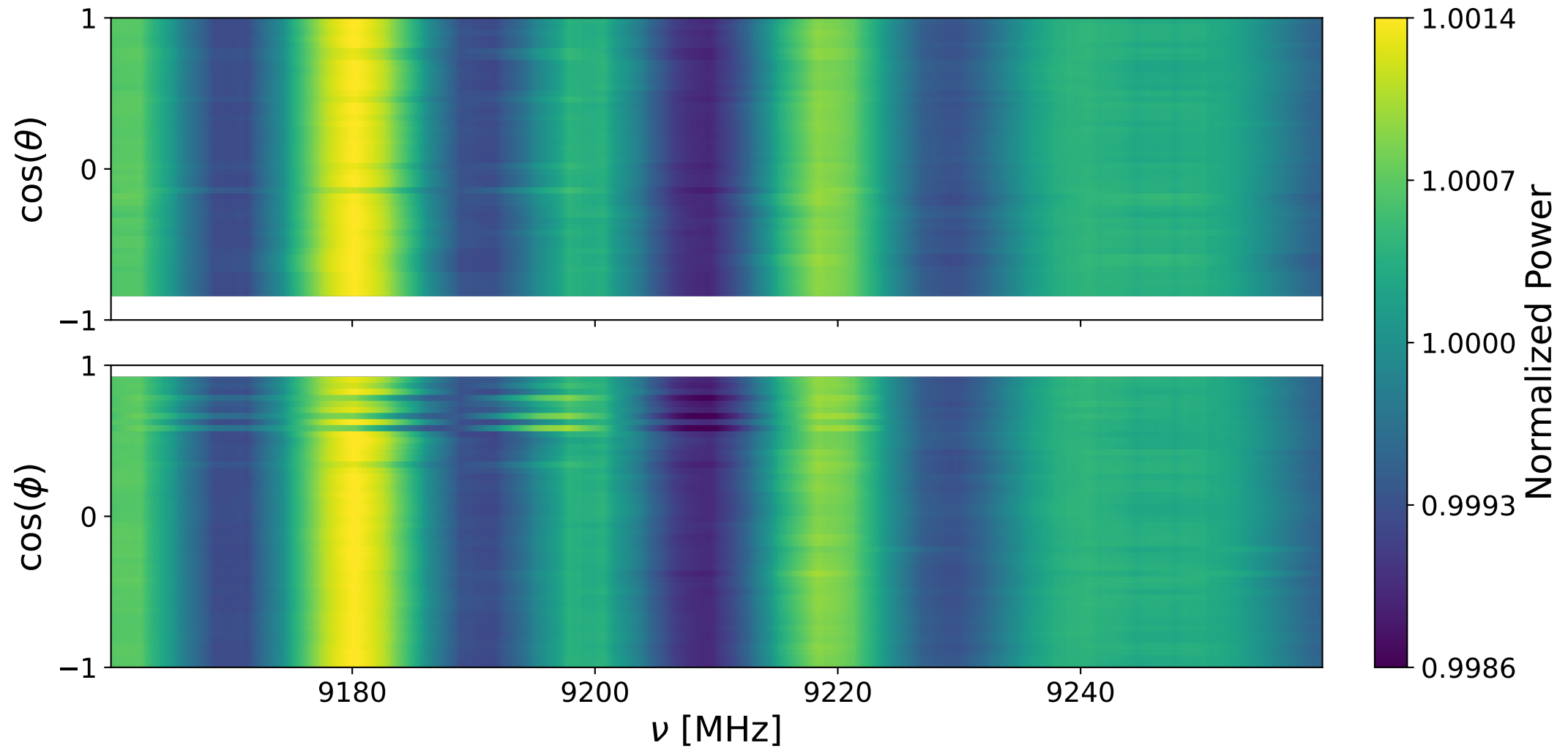
Bank 1 decay: 9160-9260 MHz
