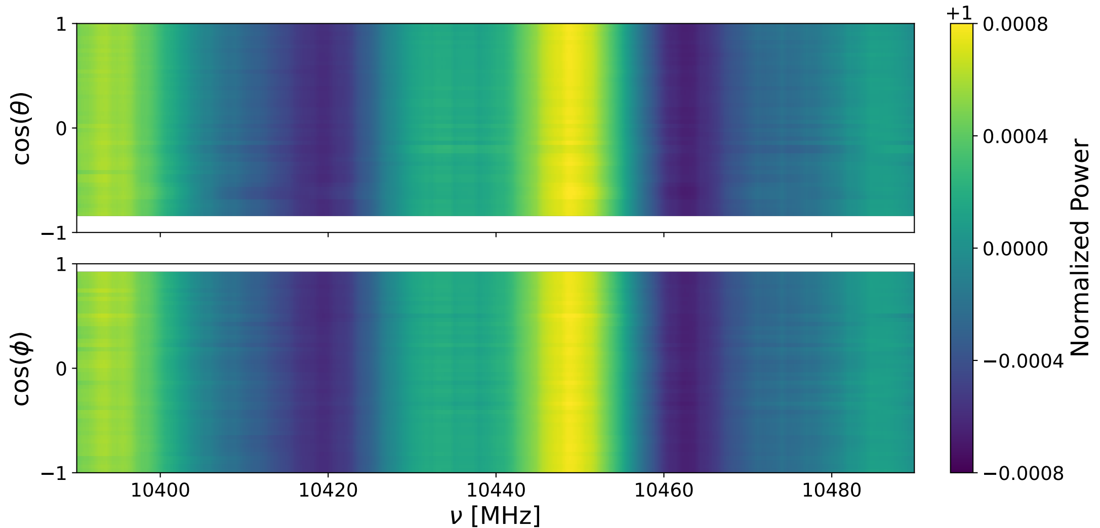
Bank 2 decay: 10390-10490 MHz
