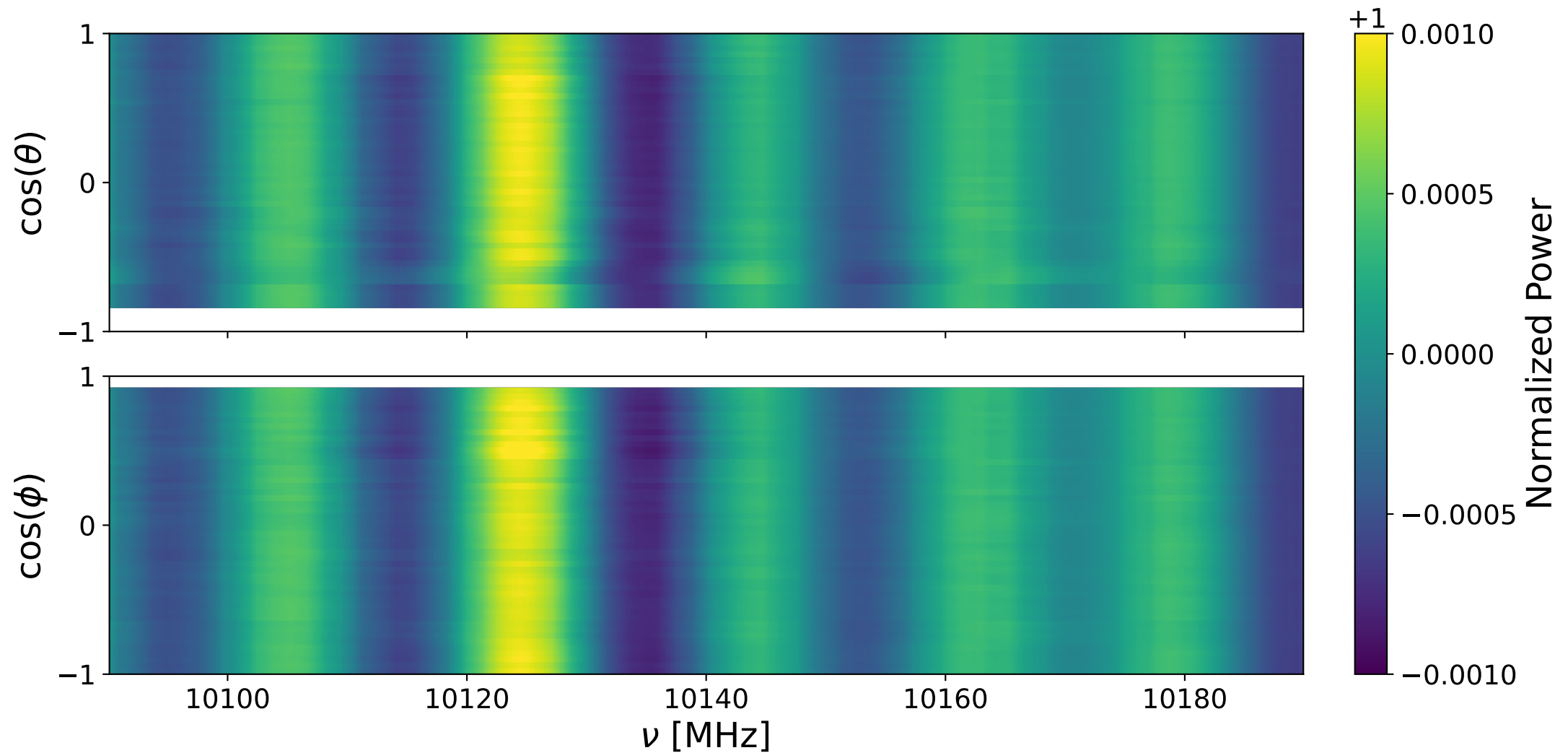
Bank 2 decay: 10090-10190 MHz
