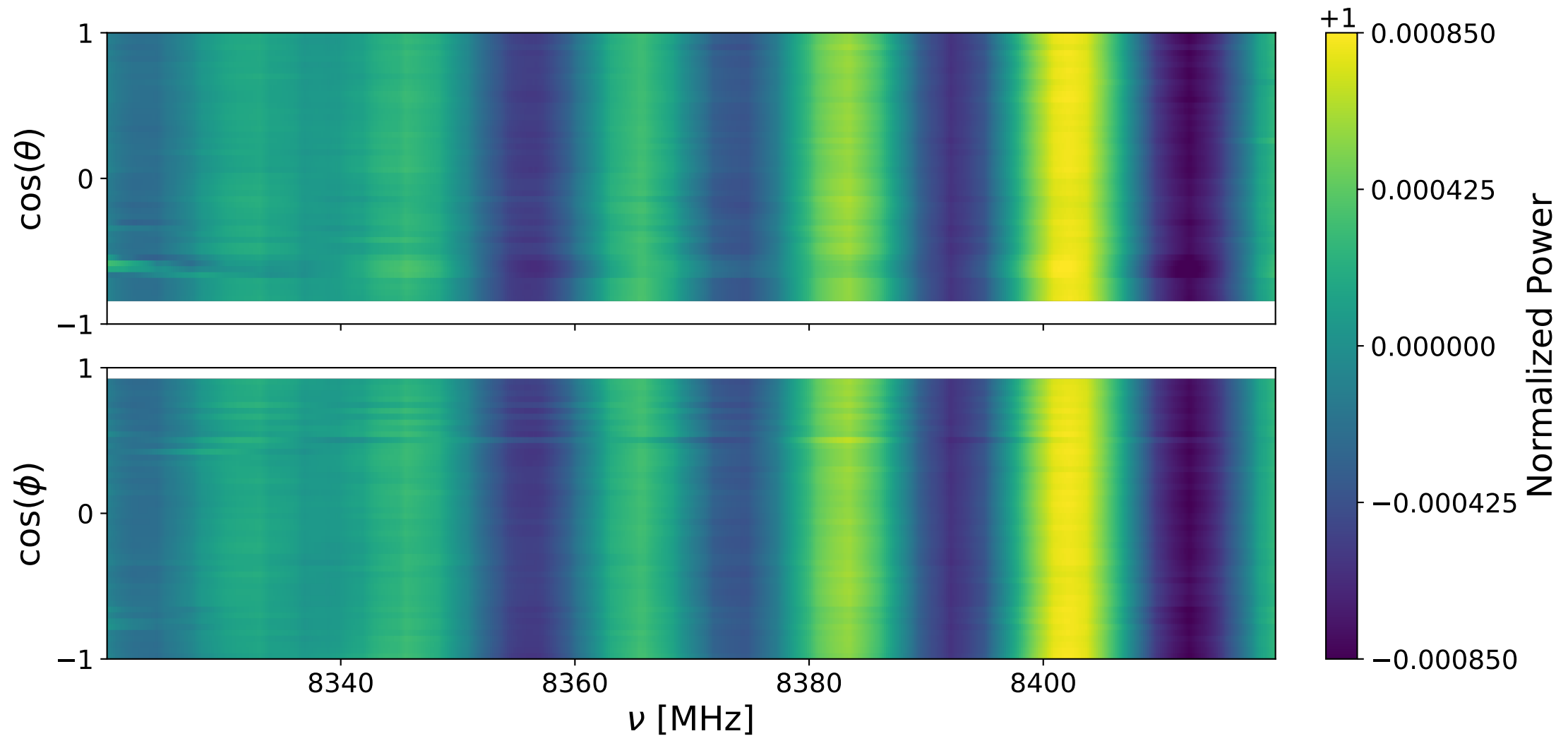
Bank 0 decay: 8320-8420 MHz
