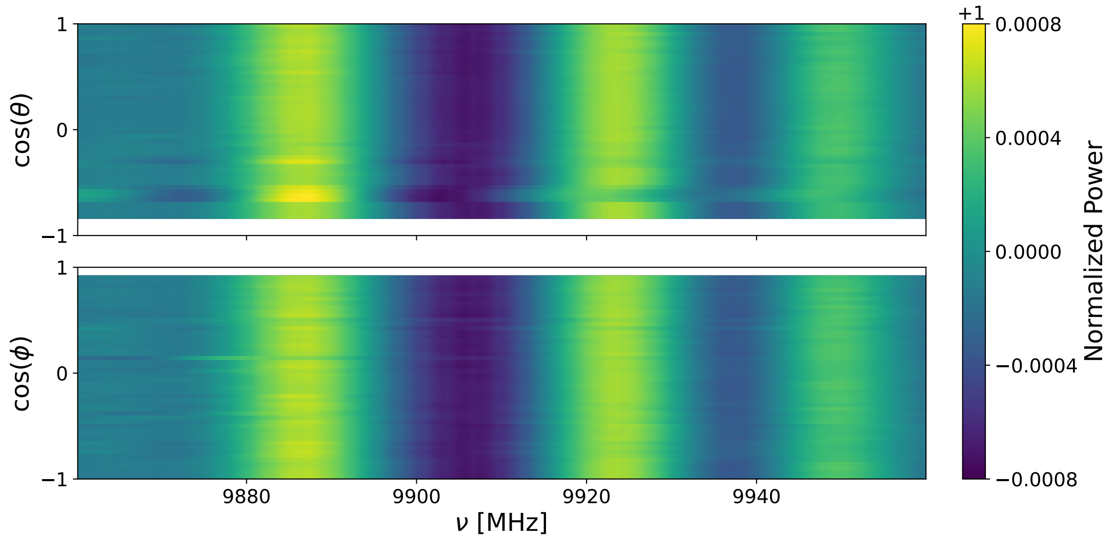
Bank 1 decay: 9860-9960 MHz
