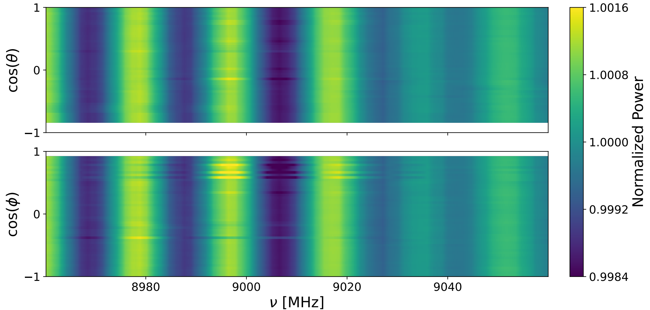
Bank 1 decay: 8960-9060 MHz
