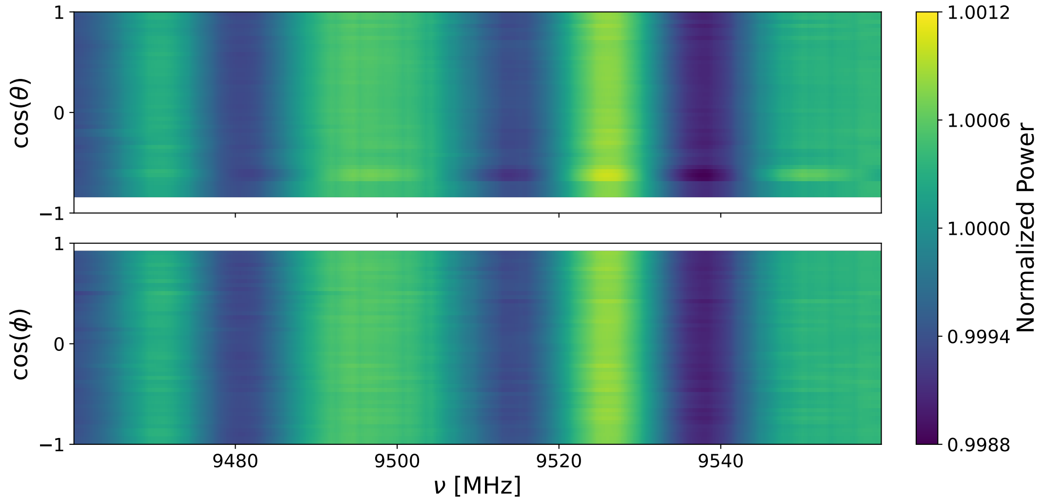
Bank 1 decay: 9460-9560 MHz
