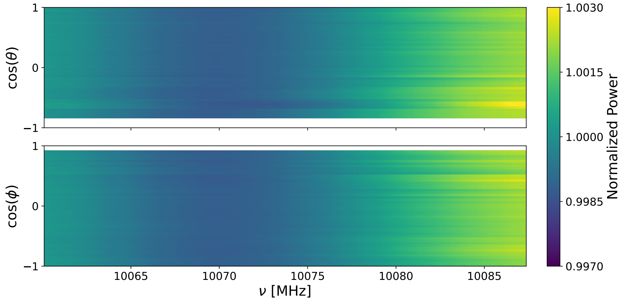
Bank 1 decay: 10060-10087 MHz
