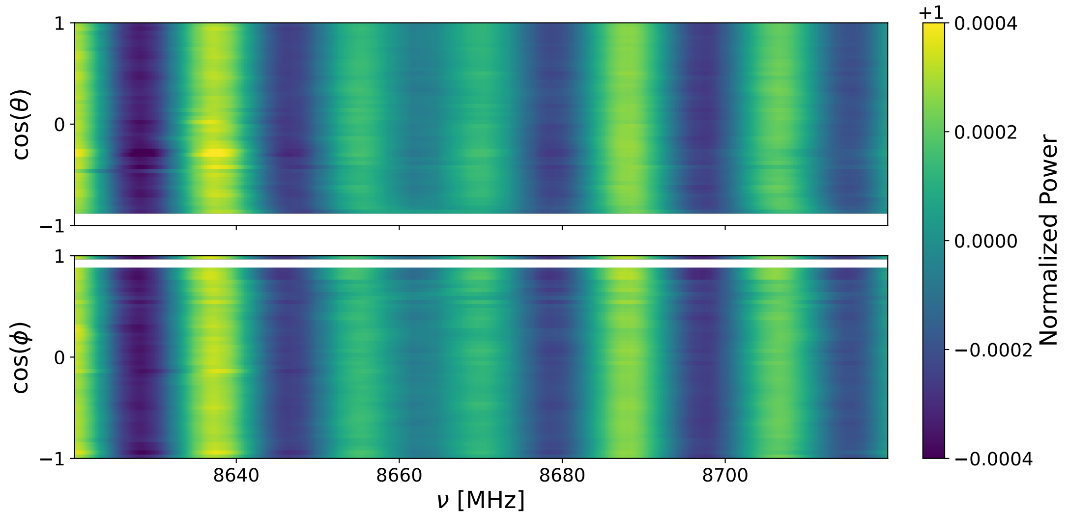
Bank 0 ann: 8620-8720 MHz
