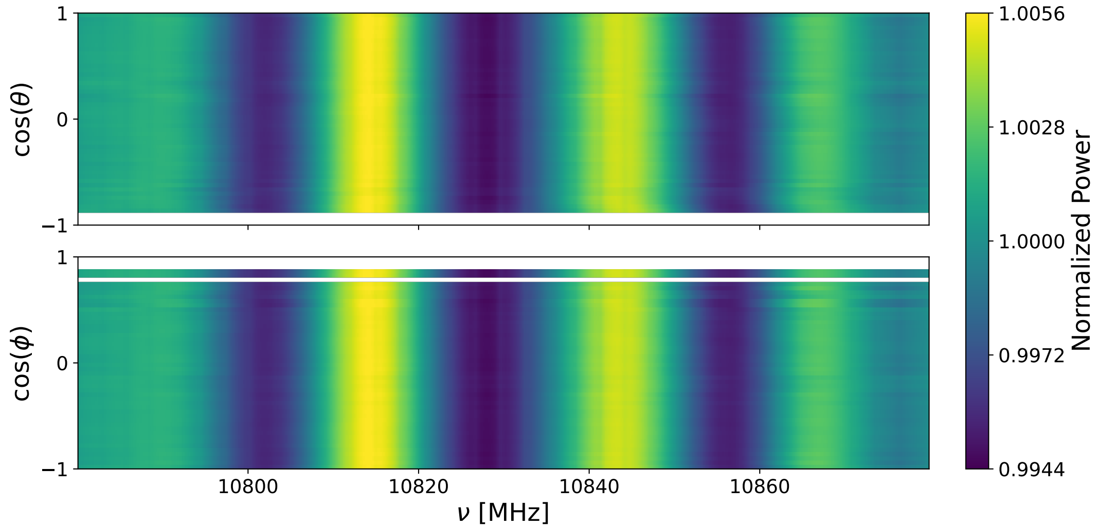
Bank 2 ann: 10780-10880 MHz
