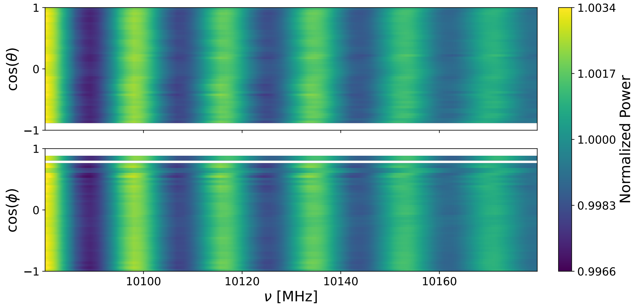
Bank 2 ann: 10080-10180 MHz
