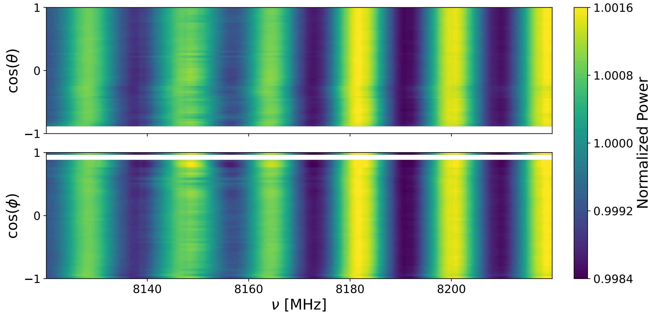
Bank 0 ann: 8120-8220 MHz
