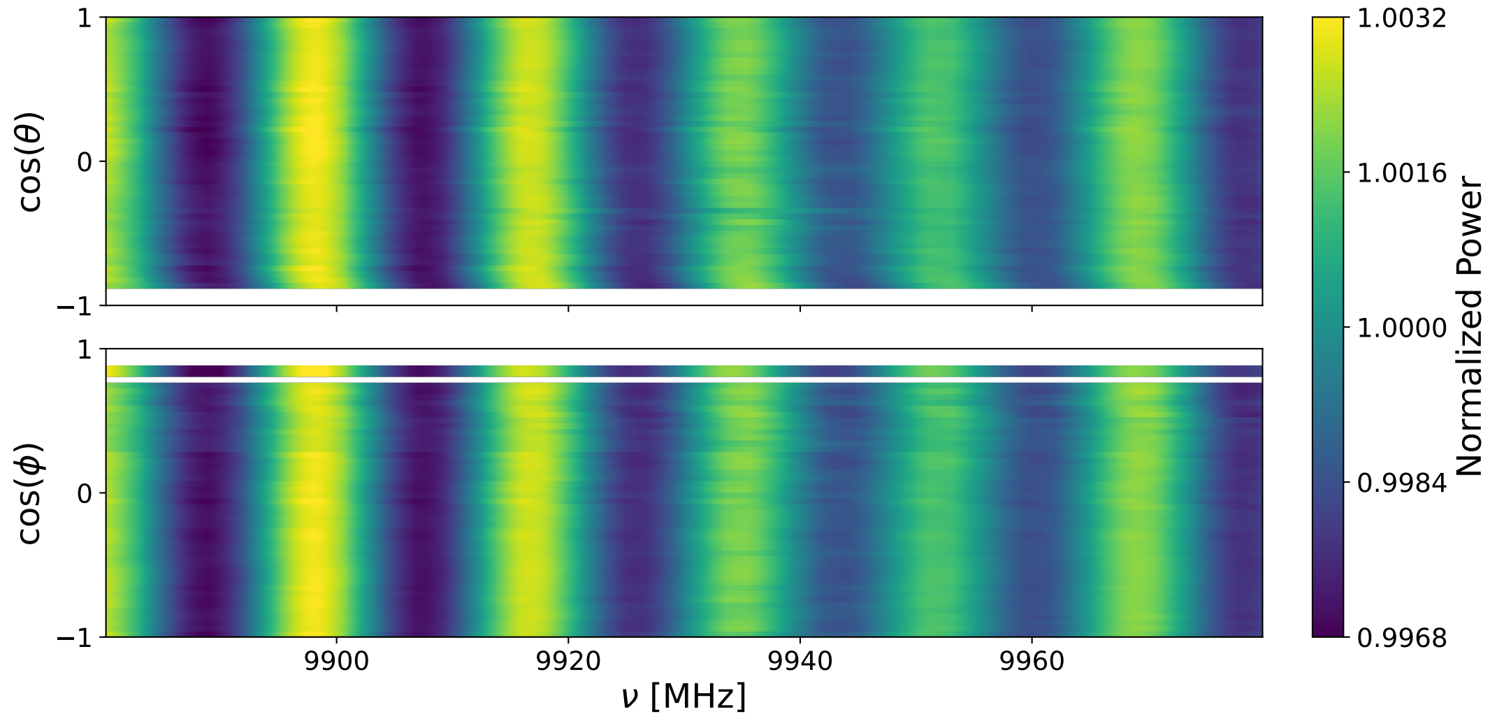
Bank 2 ann: 9880-9980 MHz
